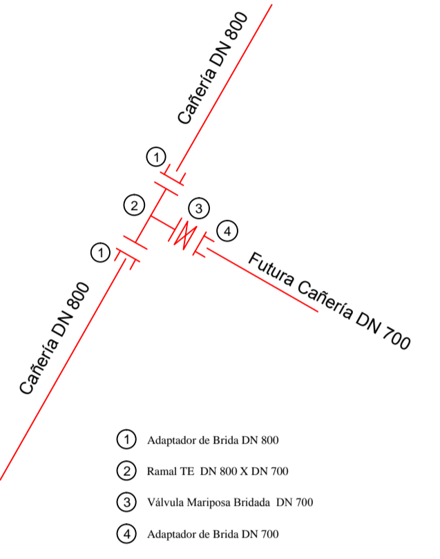
ESQUEMA (A) NUDO SALIDA OBRA 139
