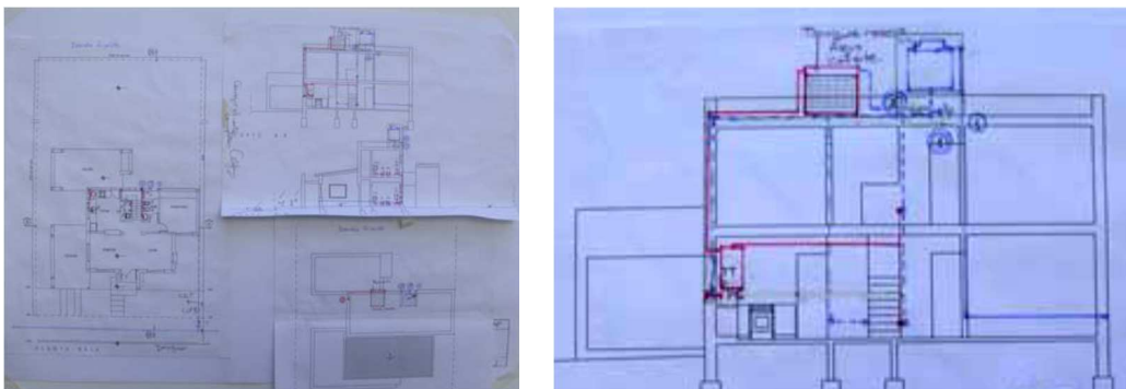
Figura 2. Agua fría y caliente con colector solar, plantas y corte
