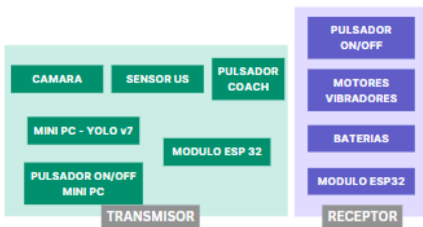
Figura N° 50 - Diagrama de bloques prototipo 3
