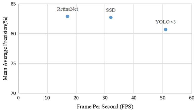
Figura 25 - Tasa de cuadros detectados por cada algoritmo
