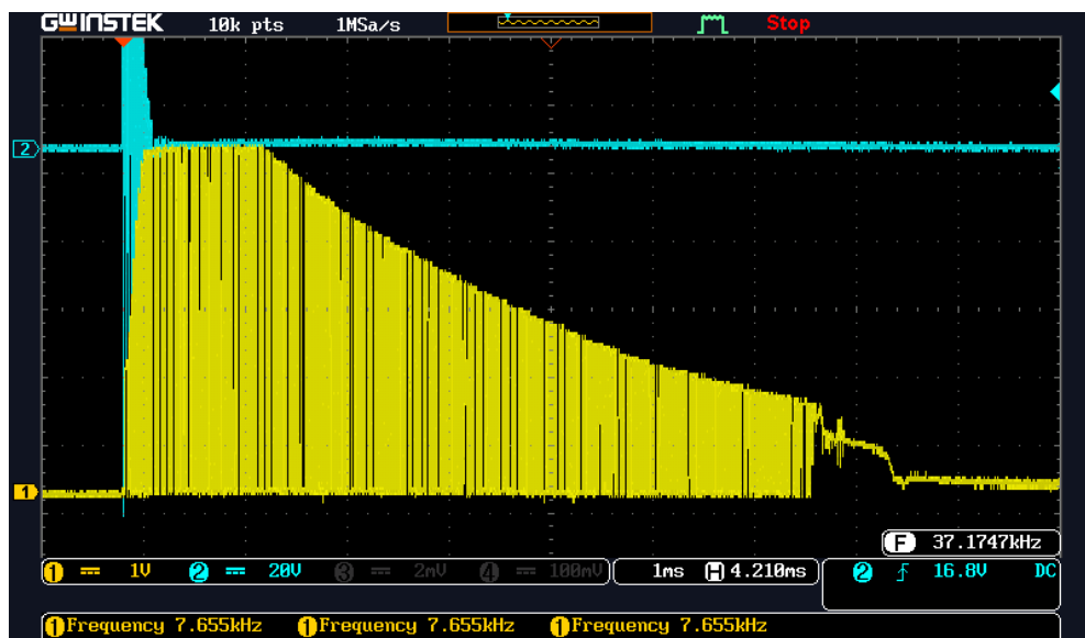
Figura N° 36: Resonancia de las señales
