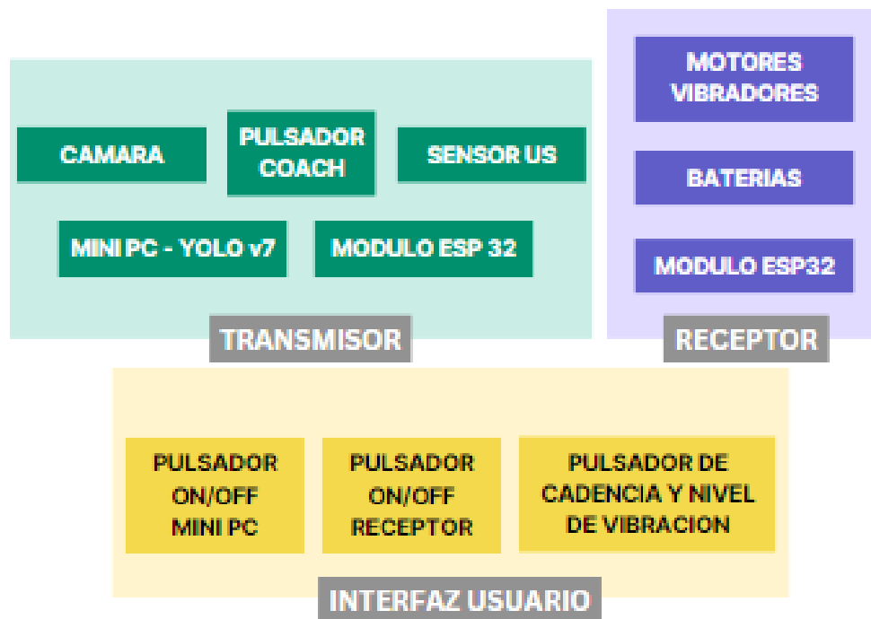
Figura 55 - Diagrama de bloques prototipo final
