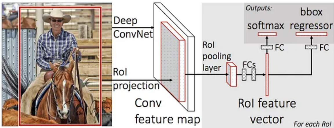
Figura 21 - Arquitectura de Faster R-CNN
