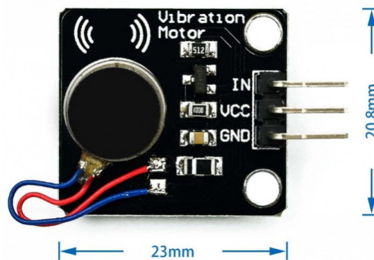
Figura N° 31: Módulo motor vibrador
