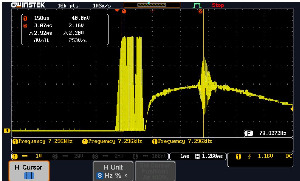
Figura N° 35 Onda de ultrasonido con obstáculo a 50 cm
