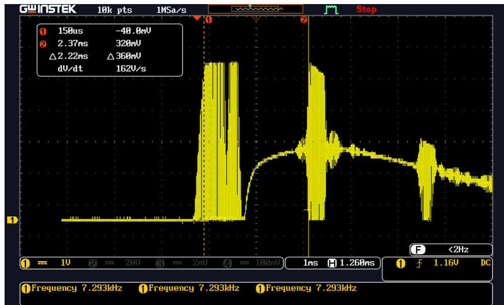
Figura N° 34: Onda de ultrasonido con obstáculo a 40cm
