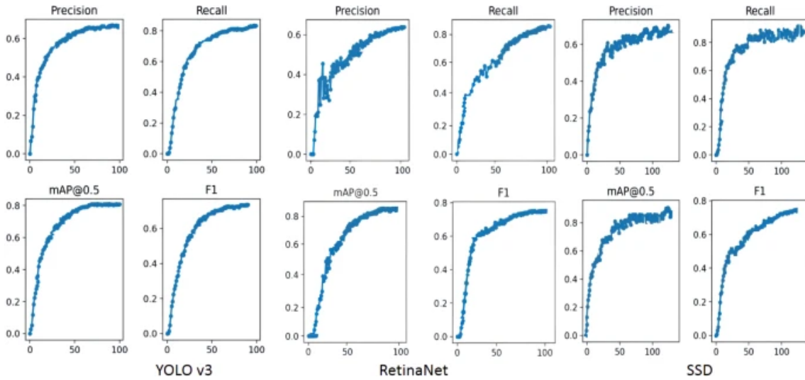
Figura 24 - Métricas de evaluación de los distintos algoritmos
