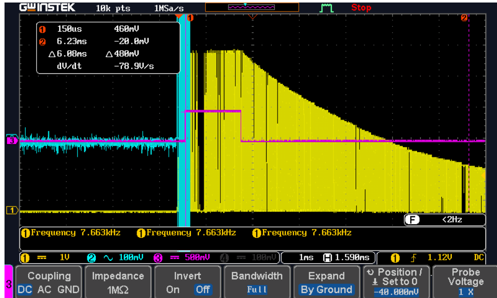
Figura N° 37: Onda de excitación de cristales piezoeléctricos
