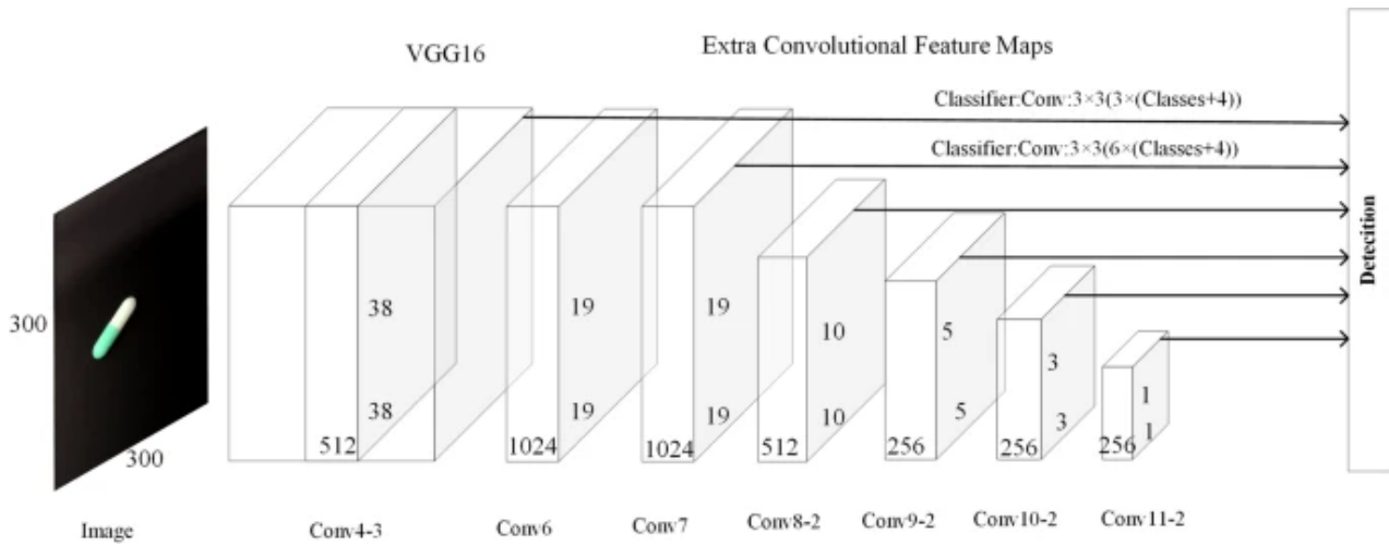
Figura 19 - Arquitectura de SSD
