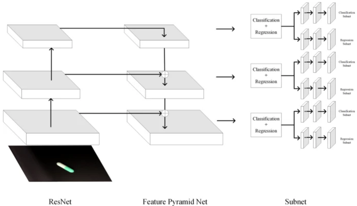
Figura 20 - Arquitectura de RetinaNet
