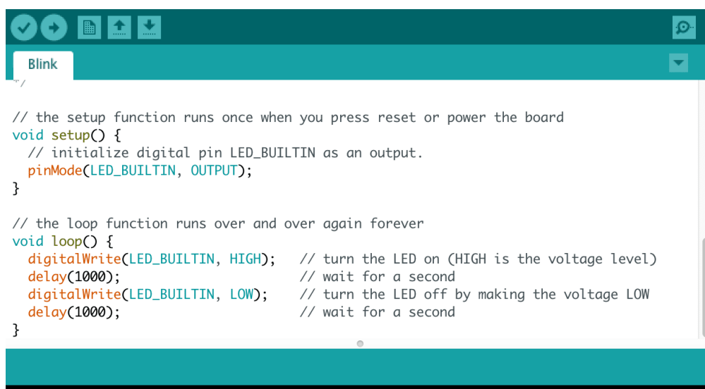
Figura N° 8: Entorno de desarrollo Arduino
