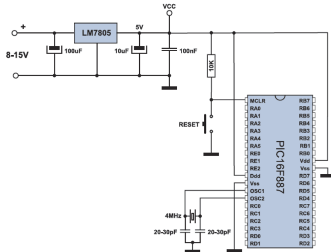
Figura N° 43: Esquema de alimentación del PIC 16F887
