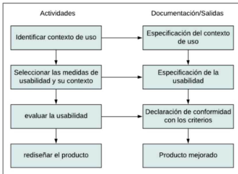
Figura N° 4: Plan recomendado para el análisis de usabilidad
