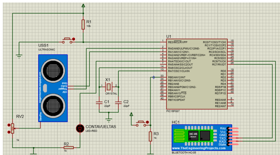
Figura N° 42: Esquema del circuito en Proteus
