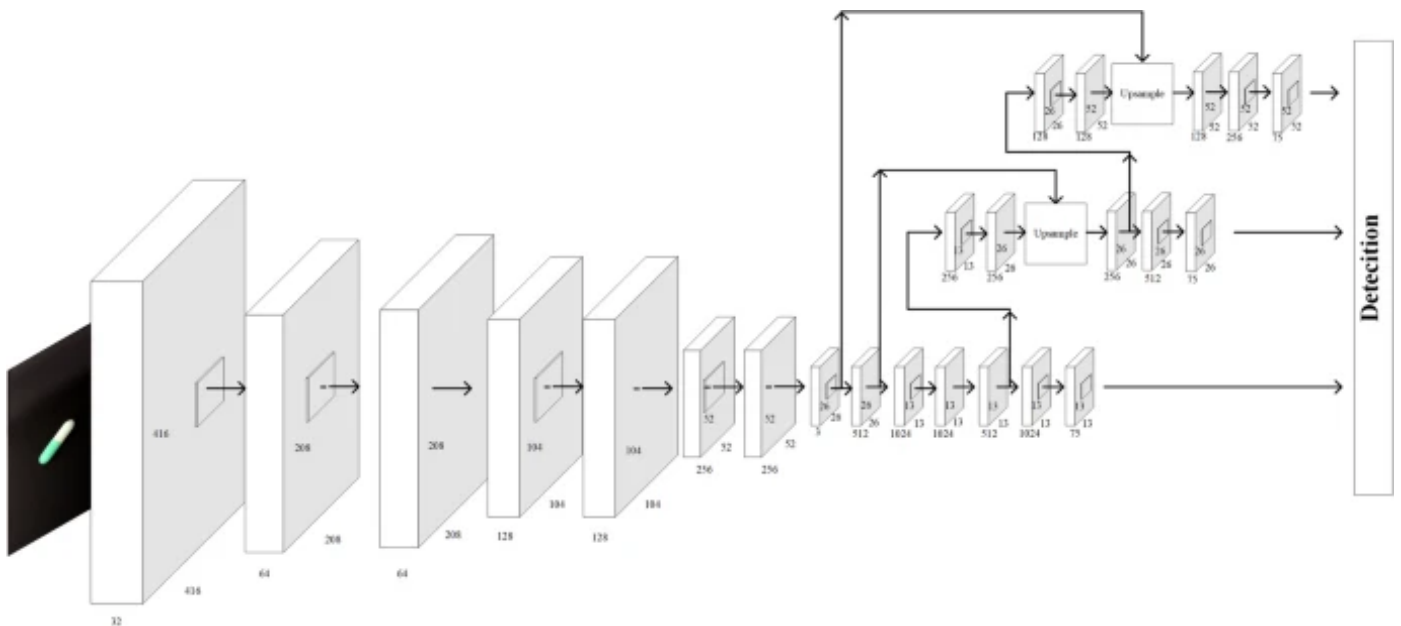
Figura 18 - Arquitectura de YOLOv3
