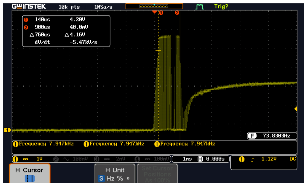
Figura N° 38: Onda de ultrasonido con recorte de goma eva sobre el sensor
