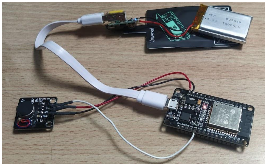
Figura N° 53: Aplicación del ESP32 en receptor. La carga de la batería se realiza de forma inalámbrica con una antena mediante un cargador Qi
