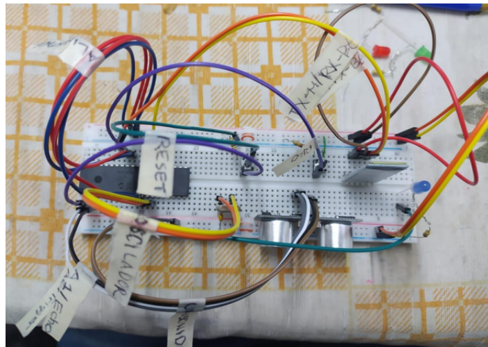
Figura N° 44: Armado y conexión de componentes en protoboard
