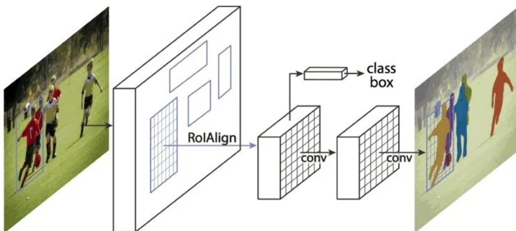
Figura 22 - Arquitectura de Mask R-CNN
