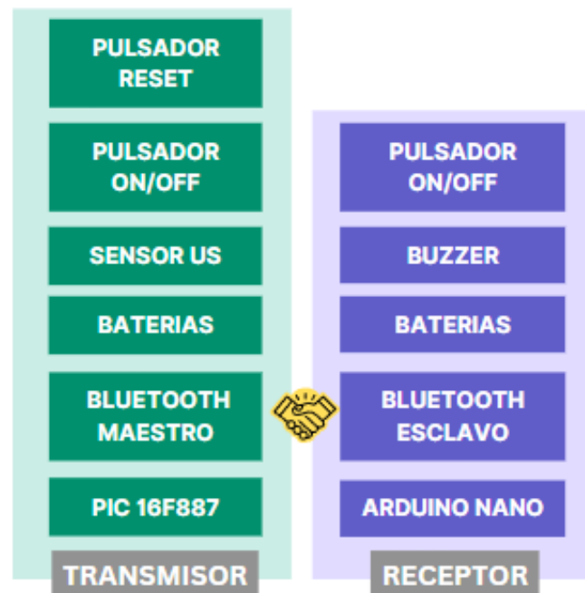
Figura 41 - Diagrama de bloques prototipo 1
