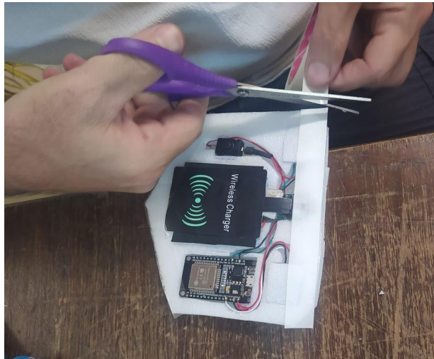
Figura N° 57: Módulo receptor, con componentes electrónicos internos a la vista
