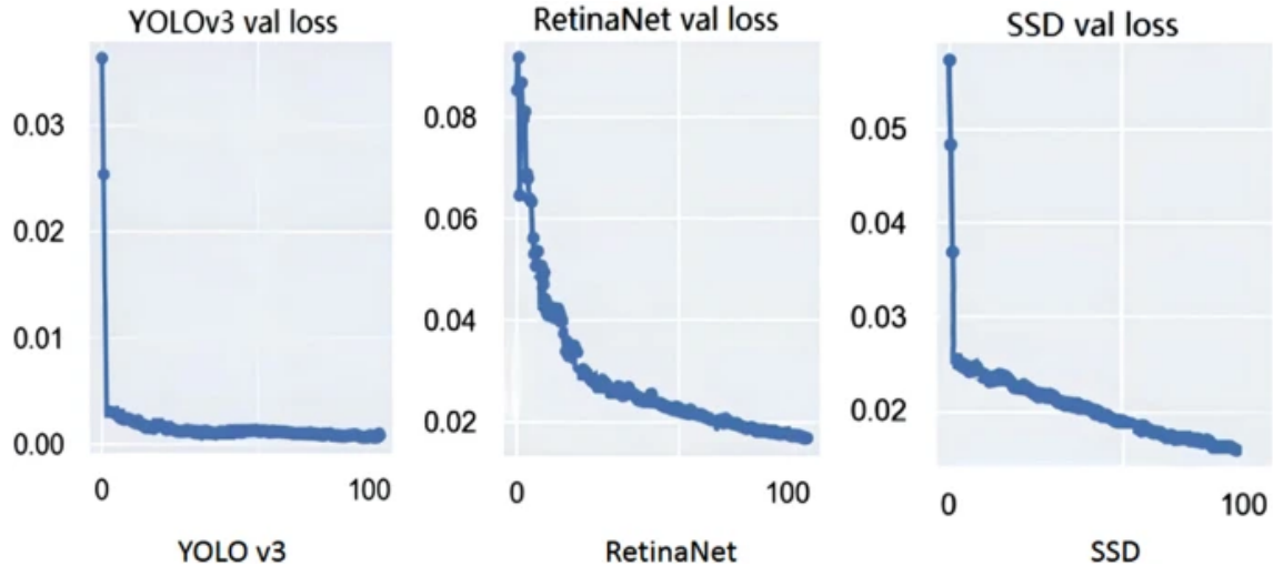
Figura 23 - Entrenamiento de algoritmos.
