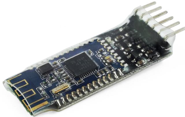
Figura N° 27: Módulo HM-10
