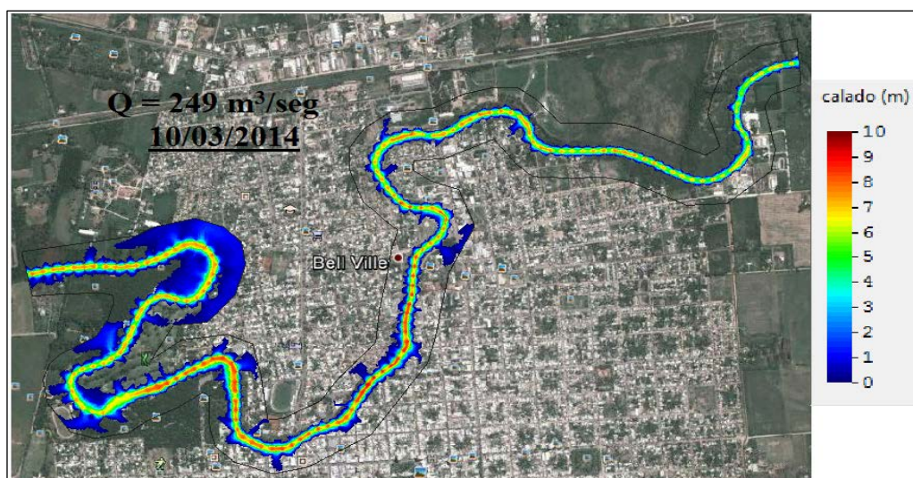
Figura 4. Esquema de áreas coloreadas de la altura de agua en el río Ctlamochita en su paso por la ciudad de Bell Ville.
