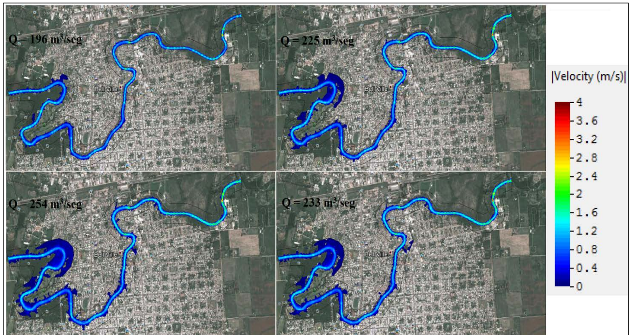
Figura 3. Esquema de áreas coloreadas de la velocidad media en el plano en el río Ctlamochita en su paso por la ciudad de Bell Ville.
