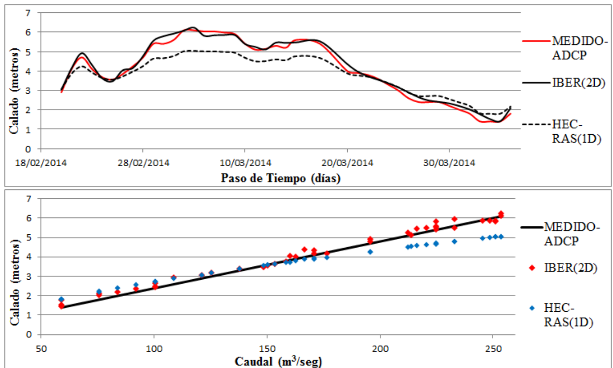
Figura 2. Resultados de calado de agua en la sección del dique Bell Ville obtenidos en campo y en los modelos numéricos unidimensional HEC-RAS y bidimensional IBER.
