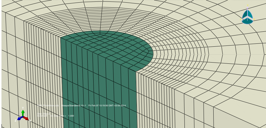
Figura 4: Detalle de la malla utilizada en el entorno del pilote. Modelo en Abaqus.
