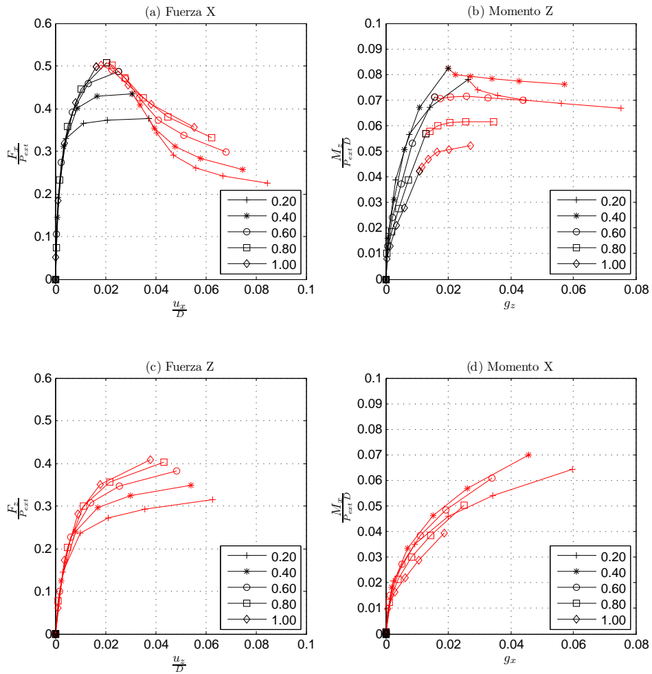
Figura 7: Curvas de respuesta del modelo en Abaqus, para las distintas profundidades desde la superficie del estrato. (a) Fuerza x vs. desplazamiento x . (b) Momento z vs giro z . (c) Fuerza z vs. desplazamiento z . (d) Momento x vs giro x . En negro corresponde a la Etapa 1 de carga y en rojo corresponde a la Etapa 2 de carga.
