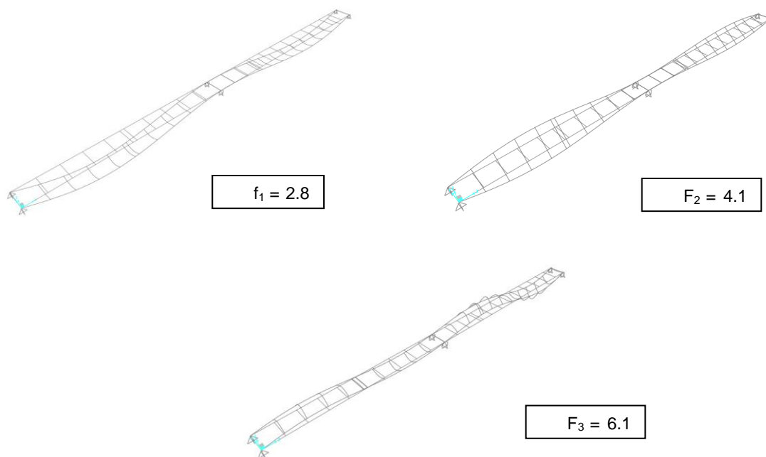
Figura 10. Primeras formas modales del puente
