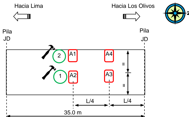
Figura 14. Disposición de sensores y puntos de impacto para el ensayo de los tramos del puente Izaguirre en Panamericana Norte. Ensayo en tramo continuo
