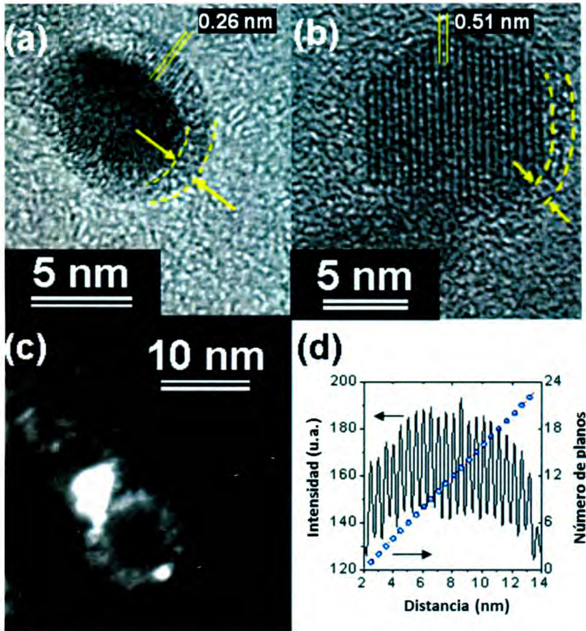
Figura 6. SPNPs de \text{Fe}_3\text{O}_4@\text{Pd-OA} : (a) micrografía HRTEM mostrando la distancia interplanar en la coraza de Pd. (b) micrografía HRTEM mostrando la distancia interplanar en el núcleo de \text{Fe}_3\text{O}_4 . (c) imagen de campo oscuro evidenciando la coraza de Pd sobre una nanopartícula. (d) Eje izquierdo : intensidad interplanar de la sección transversal del núcleo de (b) ; Eje derecho : número de planos cruzados como función de la distancia (círculos). La pendiente es la distancia interplanar: 0.51 nm.
