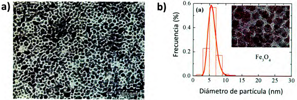
Figura 14. a) Micrografía TEM, b) histograma de la distribución de tamaños de partícula obtenida por TEM de las MNPs Fe 3 O 4 -OA y su ajuste a una función lognormal.
