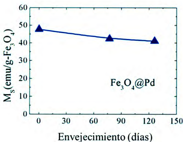
Figura 10. Medidas de magnetización de saturación ( M_s ) en función del tiempo de SPNPs de \text{Fe}_3\text{O}_4 @Pd-OA.
