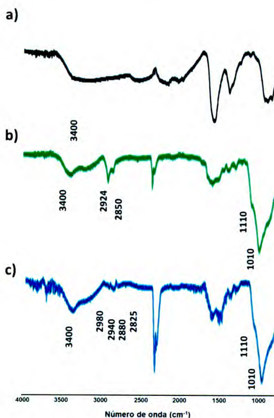
Figura 3. Espectros FT-IR en mayor detalle y en el rango 4000 - 850 \text{cm}^{-1} de a) \text{Fe}_3\text{O}_4 , b) \text{Fe}_3\text{O}_4 @APTES y c) \text{Fe}_3\text{O}_4 @APTES-cooct.
