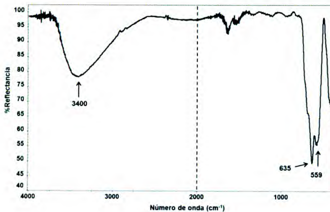
Figura 2. Espectro DRIFT de las MNPs de \gamma -Fe 2 O 3 .
