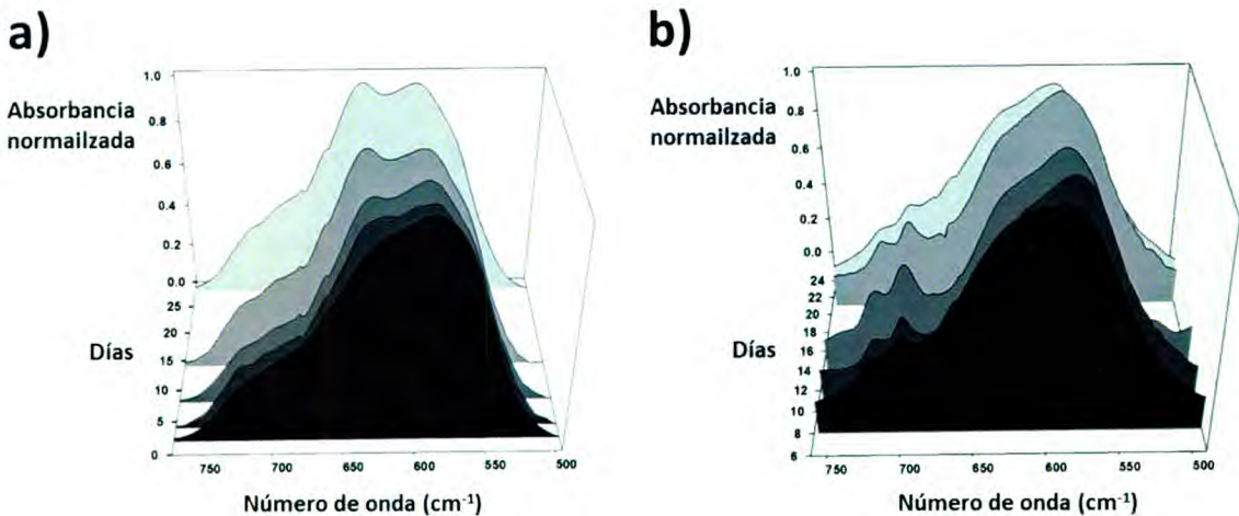
Figura 5. Espectros FT-IR de SPNPs de a) \text{Fe}_3\text{O}_4\text{-OA} y b) \text{Fe}_3\text{O}_4\text{@Pd-OA} en función del tiempo en el rango 500\text{-}760\text{ cm}^{-1} .
