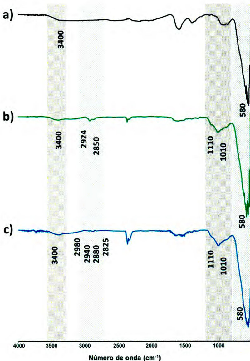
Figura 2. Espectros FT-IR a) \text{Fe}_3\text{O}_4 , b) \text{Fe}_3\text{O}_4@APTES y c) \text{Fe}_3\text{O}_4@APTES\text{-cooct} .
