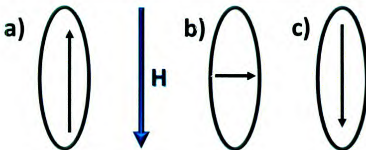
Figura All-8. Mecanismo de magnetización en partículas monodominio.
