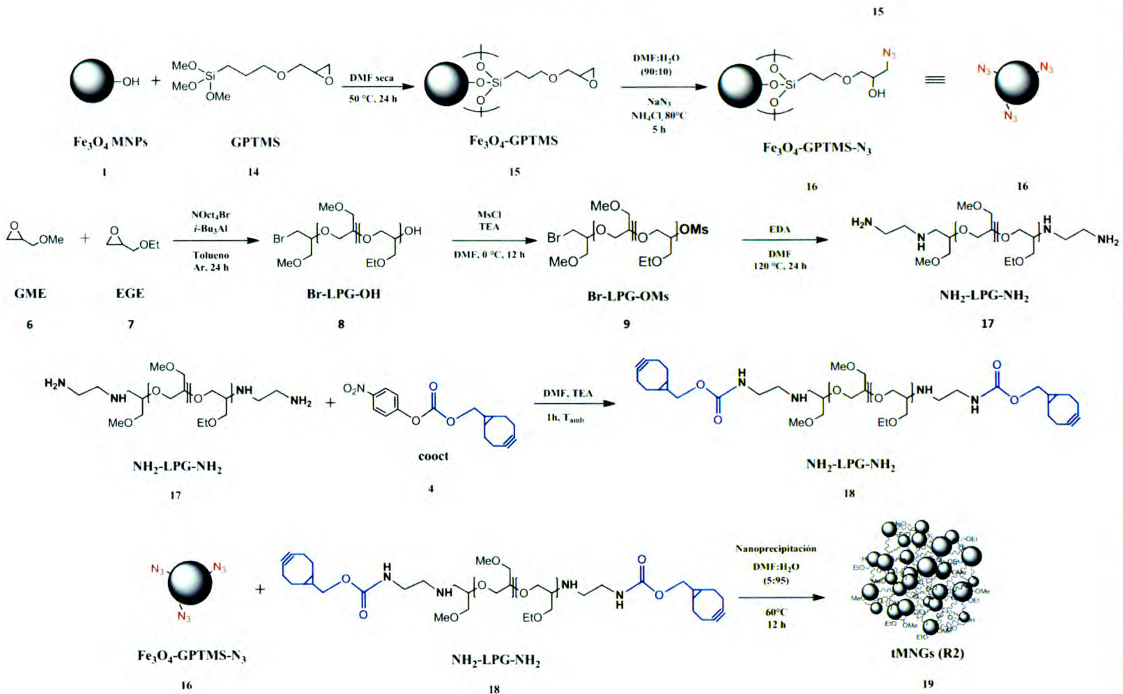
Esquema 2. Ruta sintética 2 para la obtención tMNGs basados en MNPs de \text{Fe}_3\text{O}_4 y co-polímeros termosensibles (2,5, 5 y 15 kDa) derivados de poliglicerol.
