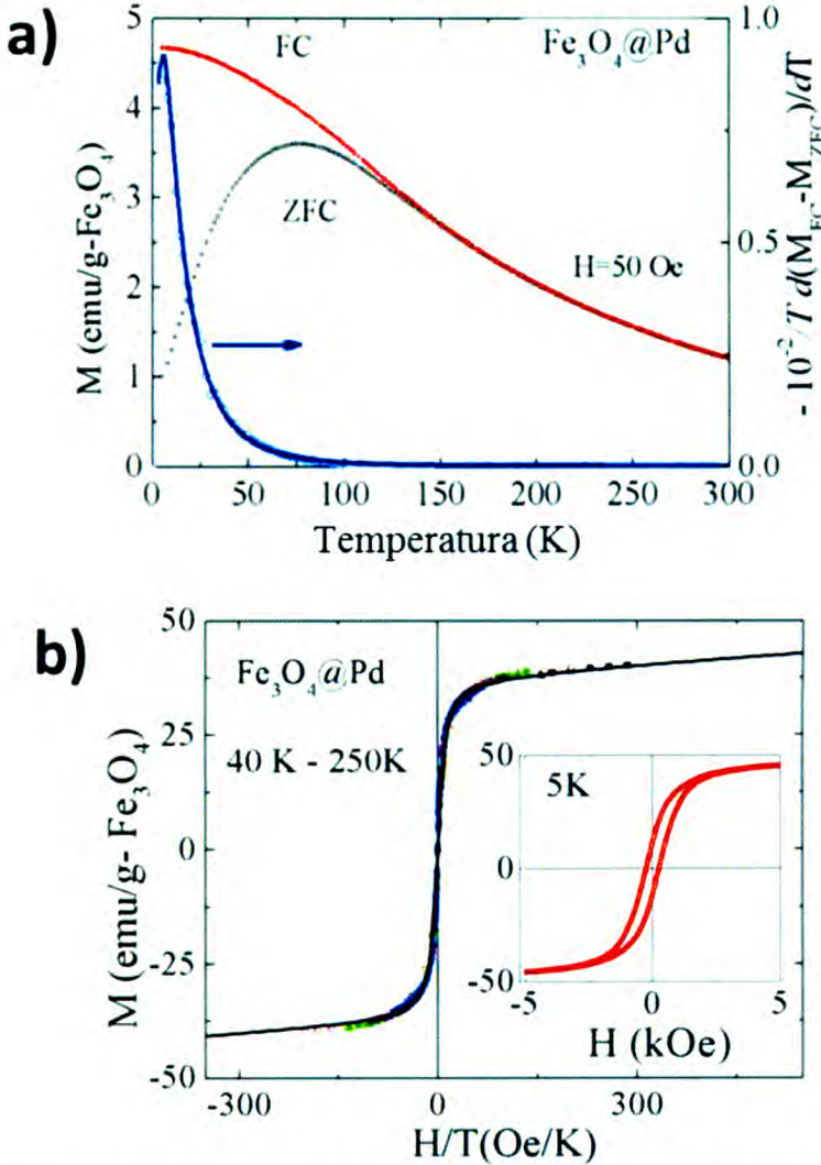
Figura 9. a) Curvas ZFC y FC ( M vs. T ) medidas a 50 Oe y b) Curva universal M vs H/T (recuadro pequeño: curva M vs. H a 5 K mostrando un pequeño ciclo de histéresis) de Fe_3O_4@Pd -OA.
