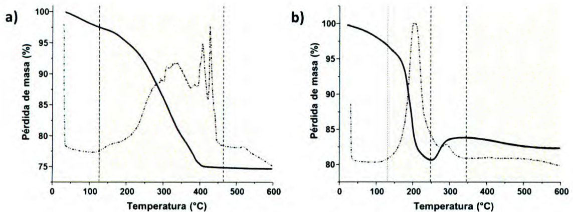
Figura 8. Curvas TGA (línea sólida) y DSC (línea punteada) de a) Fe 3 O 4 -OA y b) Fe 3 O 4 @Pd-OA.
