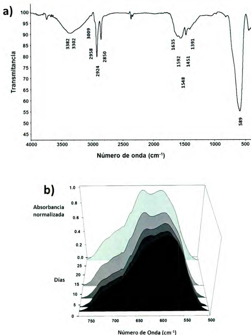
Figura 12. a) Espectro FT-IR, b) seguimiento de la oxidación de MNPs de \text{Fe}_3\text{O}_4 -OA.
