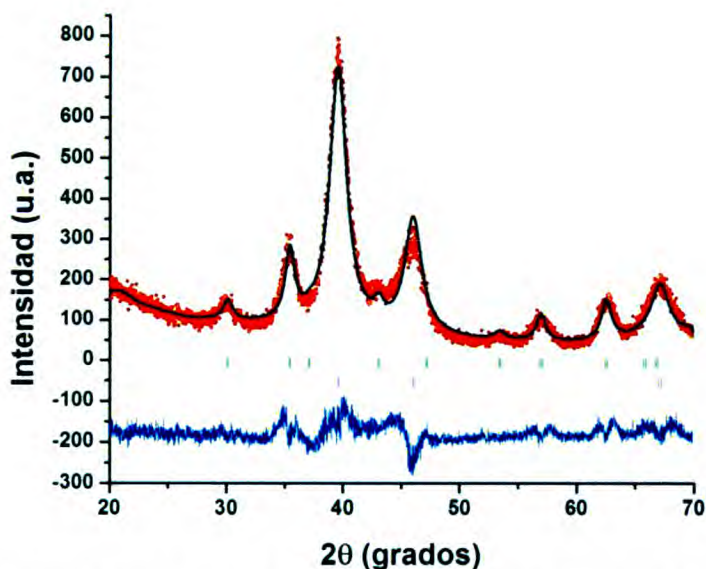
Figura 4. Refinamiento patrón PXRD de \text{Fe}_3\text{O}_4 @Pd-OA, patrón experimental ( \bullet ), patrón calculado ( - ), posiciones de Bragg de \text{Fe}_3\text{O}_4 ( \uparrow ), posiciones de Bragg de Pd ( \uparrow ) diferencia entre patrones experimental y calculado ( - ).
