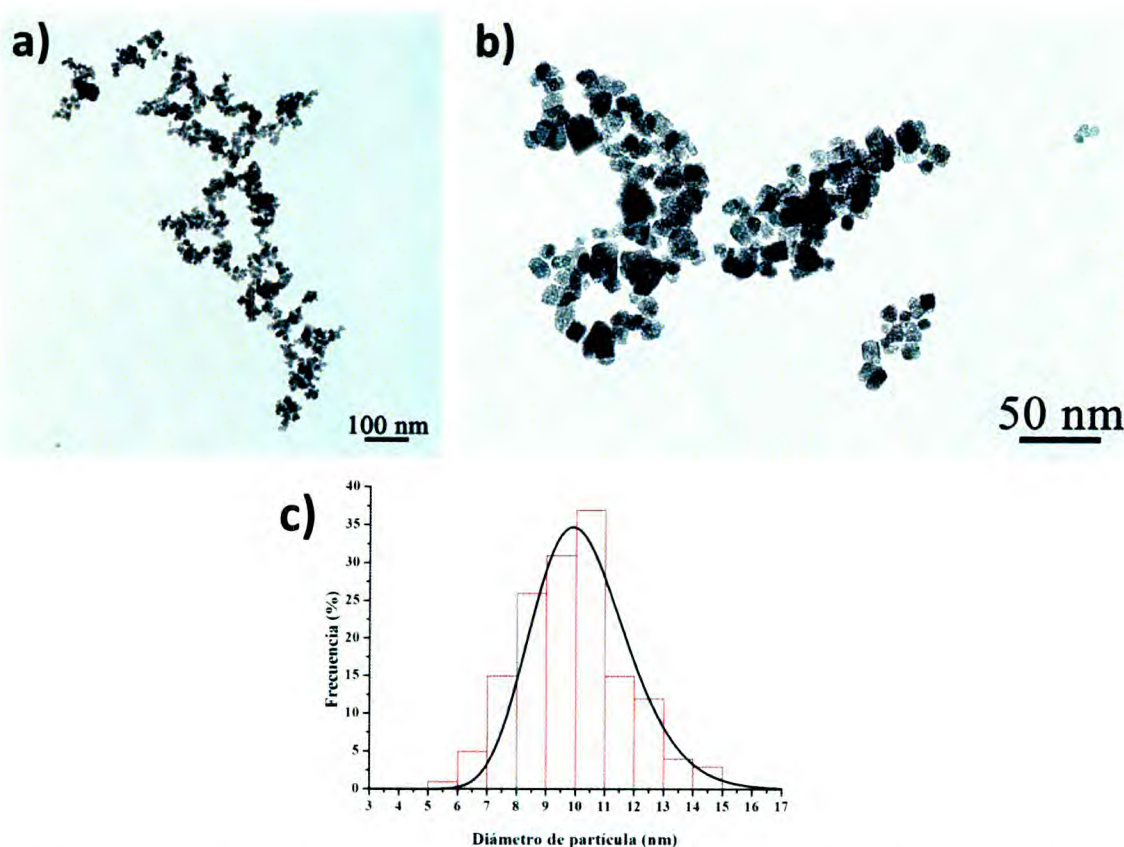
Figura 1. Micrografías TEM de MNPs de \text{Fe}_3\text{O}_4 obtenidas por co-precipitación, a) menor magnificación, b) mayor magnificación y c) histograma de distribución de tamaños.
