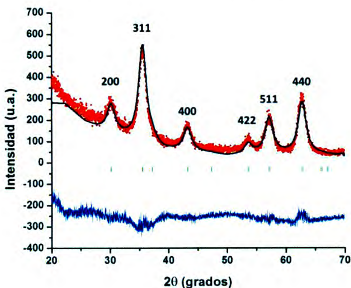
Figura 11. Refinamiento patrón PXRD de \text{Fe}_3\text{O}_4 -OA en el grupo espacial Fd-3m , patrón experimental (●), patrón calculado (—), posiciones de Bragg (|), diferencia entre patrones experimental y calculado (—).
