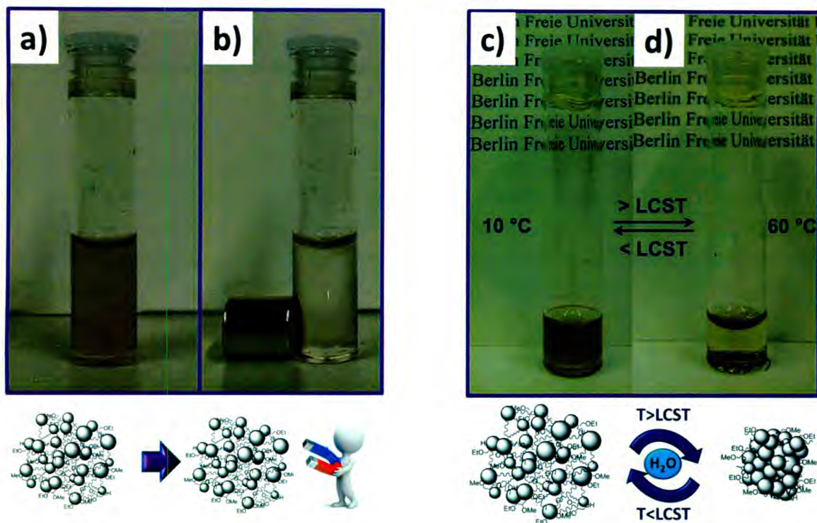
Figura 11. tMNGs (R1b): a) dispersados en H_2O MQ a T_{amb} , b) atraídos por imán a T_{amb} , c) dispersados en H_2O MQ a 10\text{ }^\circ\text{C} y d) precipitados a 60\text{ }^\circ\text{C} sin la necesidad de un imán.
