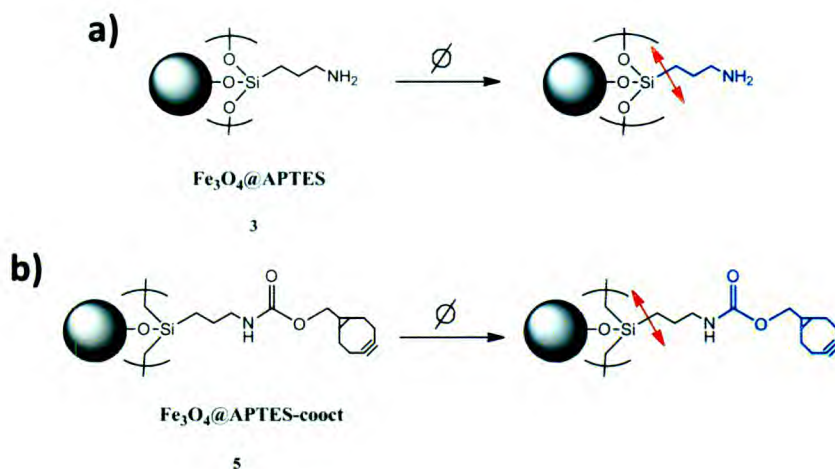
Figura 4. Representación de la degradación térmica asociada al fragmento orgánico de las MNPs modificadas: a) con APTES, b) con APTES y cooct.
