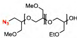
\text{N}_3\text{-LPG-OH}
