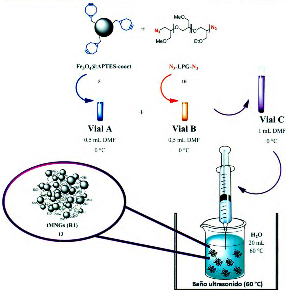
Esquema 3. Síntesis de tMNGs (R1b): Metodología nanoprecipitación.
