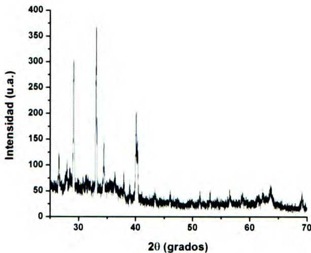
Figura 16. Patrón PXR de una muestra sintetizada por descomposición del complejo Fe-Urea en aire a 350 °C.
