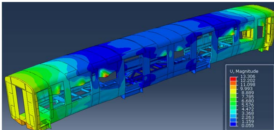
Figura 6. Deformada del coche para la combinación C.2. Unidades: mm.
