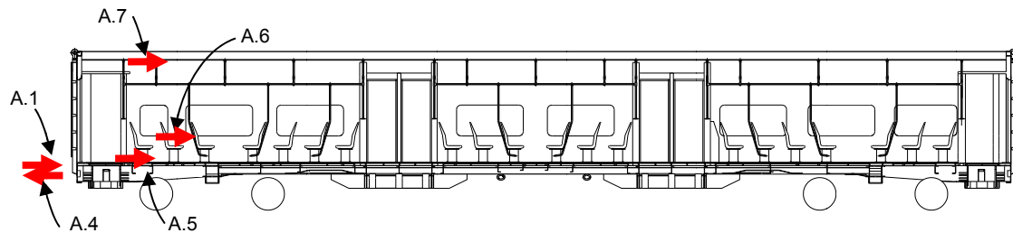
Figura 2. Cargas horizontales de verificación según la normativa Requisitos de dimensionamiento de las estructuras de los vehículos ferroviarios
