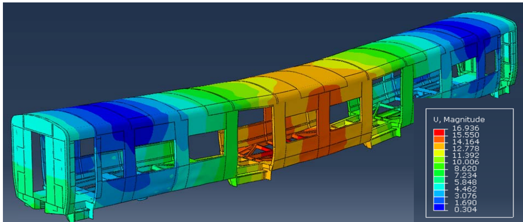
Figura 7. Deformada del coche para el estado de carga A.8 (vista 3D). Unidades: mm.
