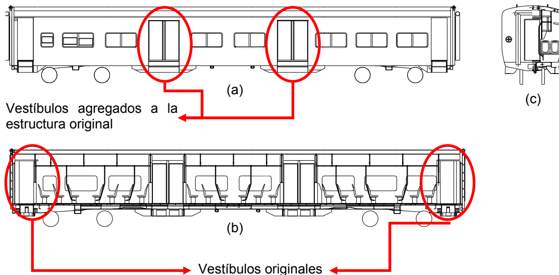
Figura 1. Geometría general del coche AERFER T1000 modificado. (a) Vista lateral. (b) Corte longitudinal. (c) Corte transversal.
