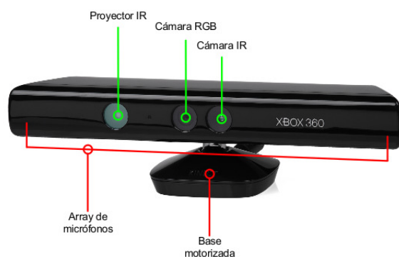
Fig. 1: Microsoft Kinect. (Adaptado de Wikipedia, 2012).
