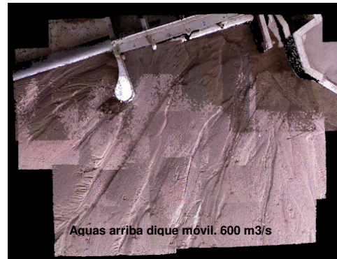
Fig. 9: Área relevada aguas arriba del dique móvil. Mosaico de imágenes RGB.
