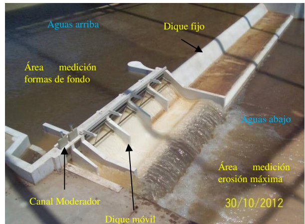
Fig. 4: Modelo físico del Dique Los Molinos. Obras de regulación. Ensayo para medición de erosión. Caudal= 900 m 3 /s.
