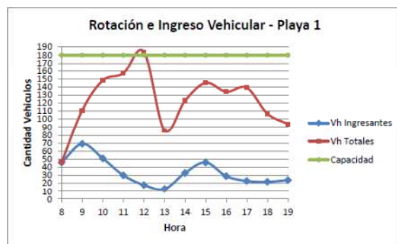
Figura 7. Variación horaria de la demanda.
