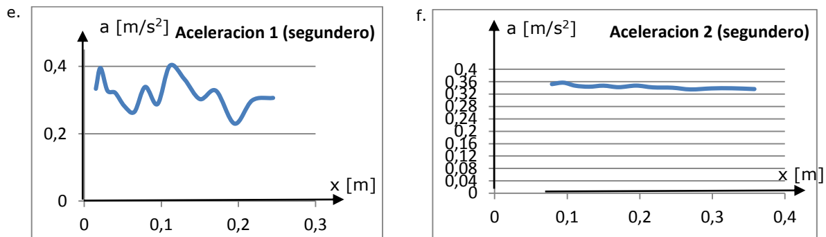
Figura 11. Representaciones gráficas de aceleración vs. Posición, por los tres métodos.
