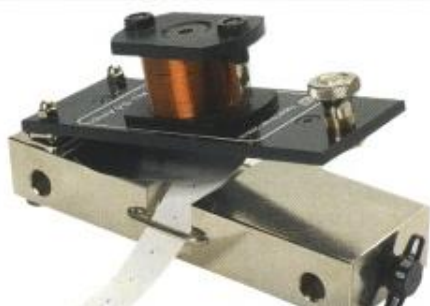
Figura 4. Registrador de movimientos.
