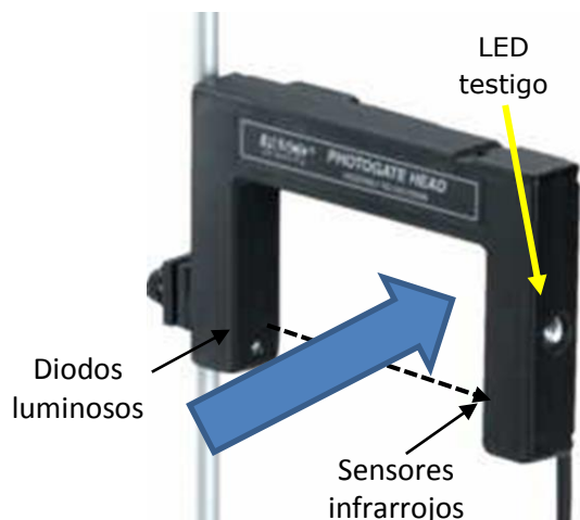
Figura 6. Barrera infrarroja.
