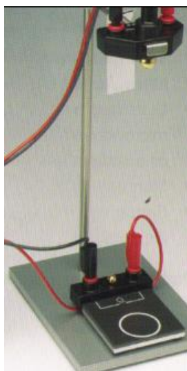
Figura 5. Electroimán sosteniendo un cuerpo - Práctica de caída libre.
