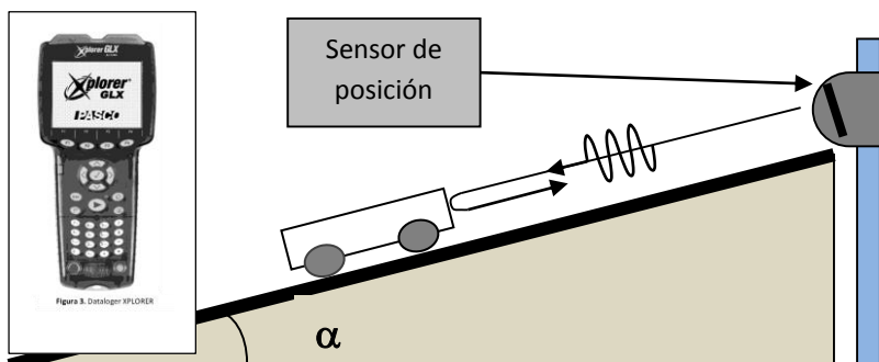
Figura 7. SAD con sensor ultrasonoro de posición.
