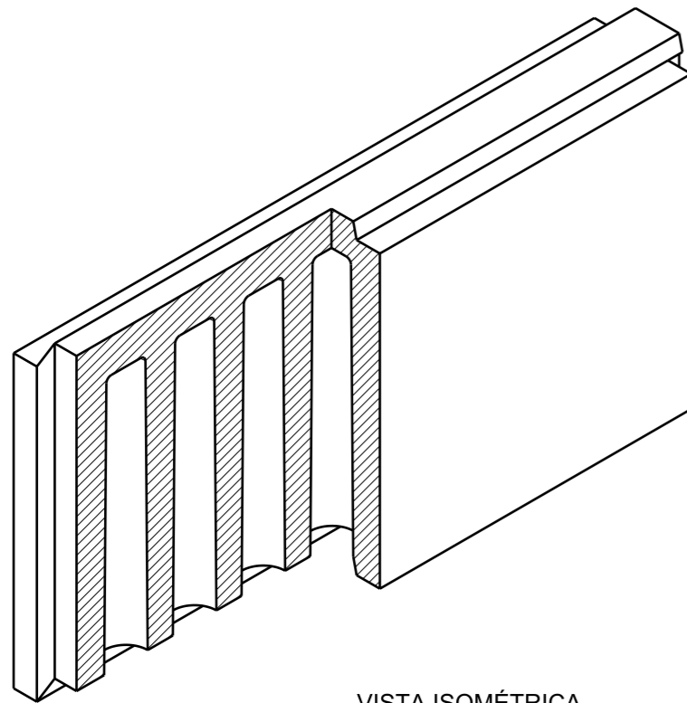
VISTA ISOMÉTRICA ESCALA 1:5
