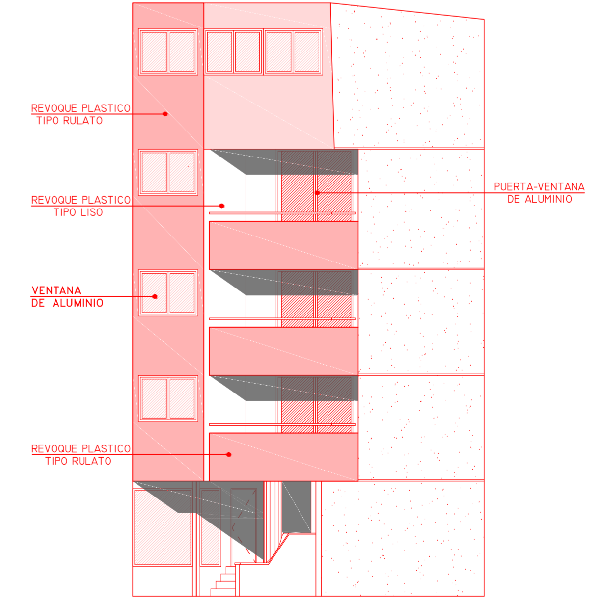
FACHADA CALLE RIVERA
