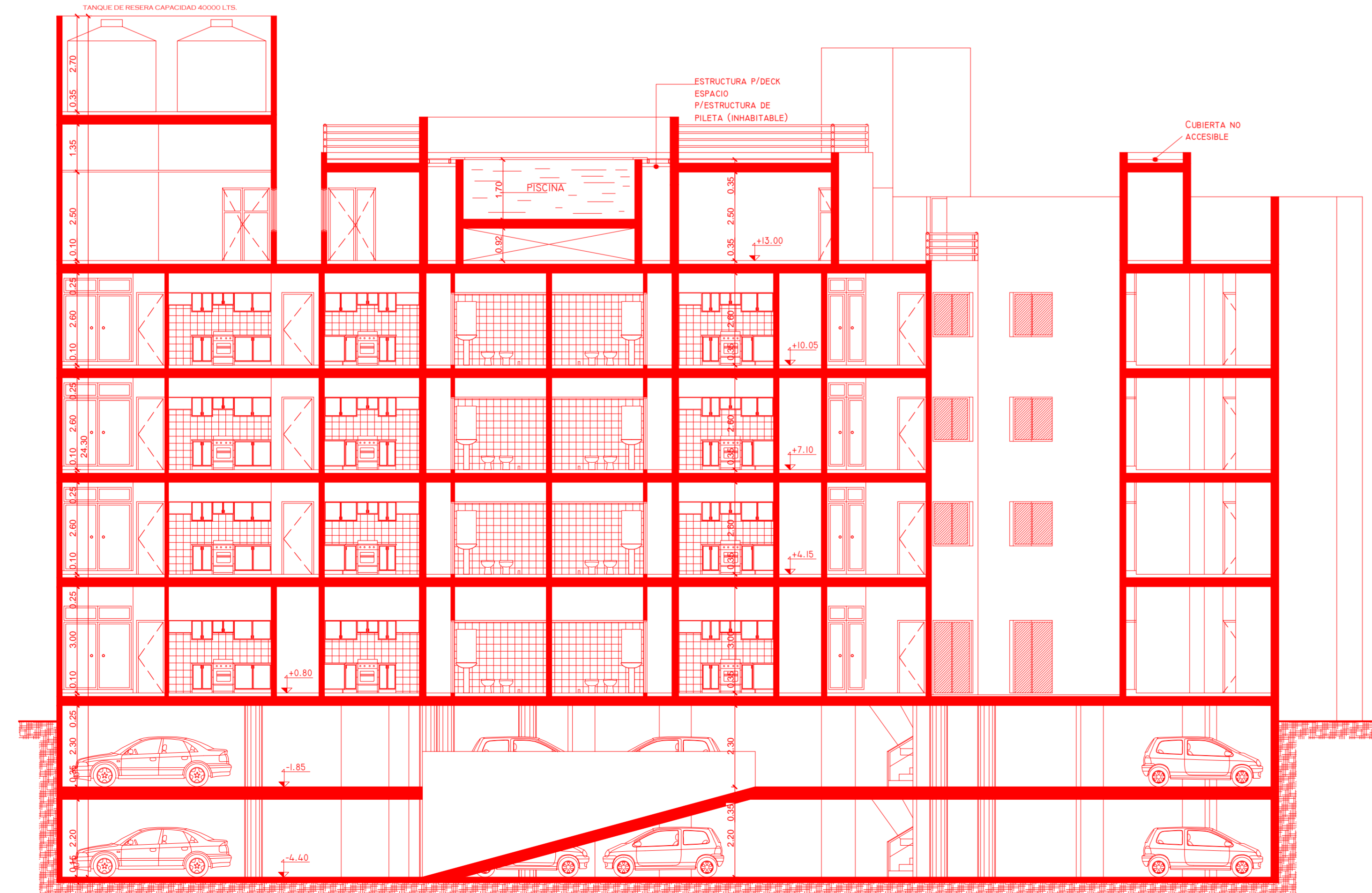
CORTE BB ESC. 1:100
