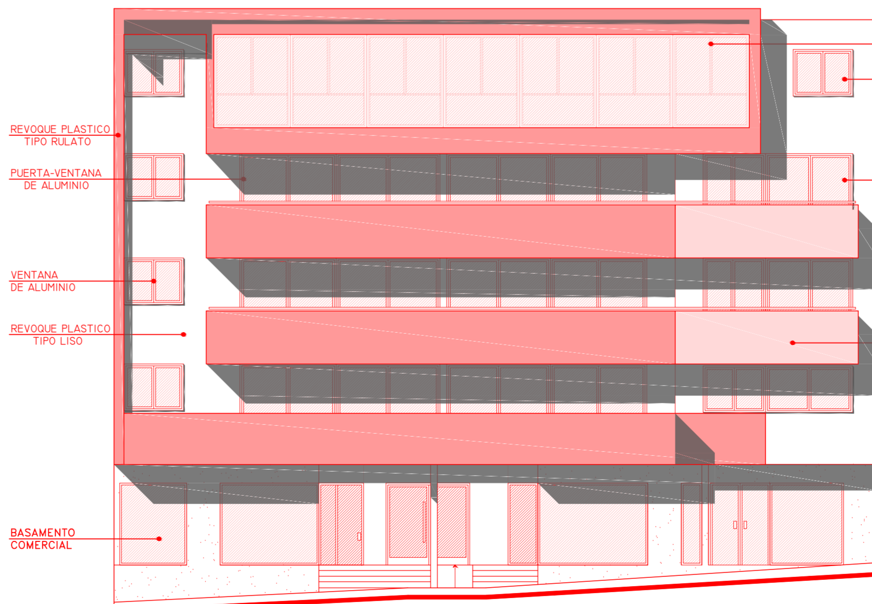
FACHADA CALLE JUAN B. JUSTO
