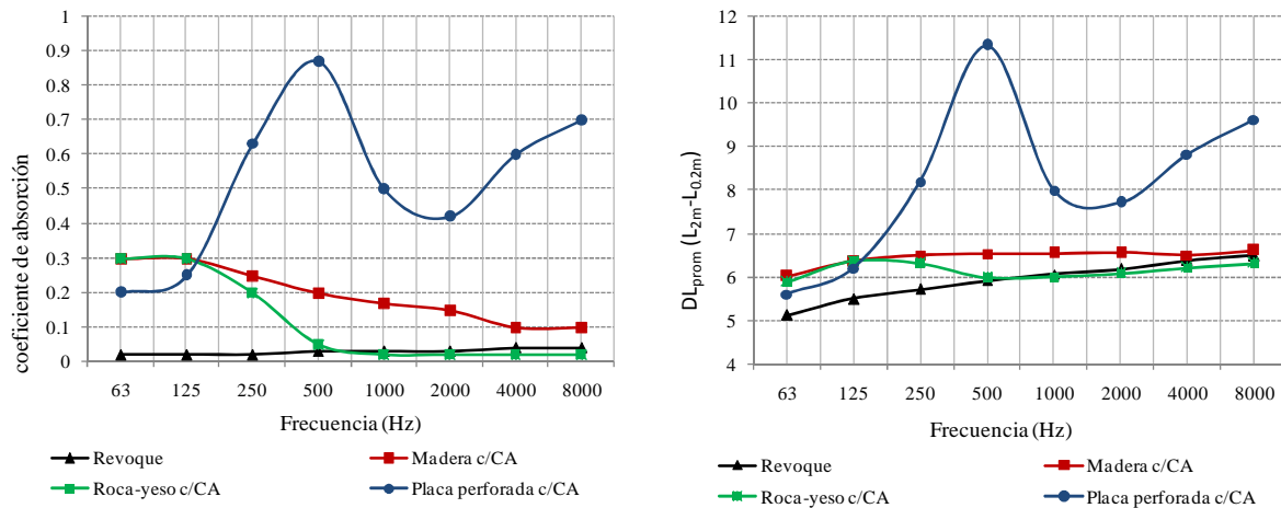
Figura 12: Absorción cielorraso y diferencia L promedio ( L_{2m} - L_{0,20m} )- tipo B5
