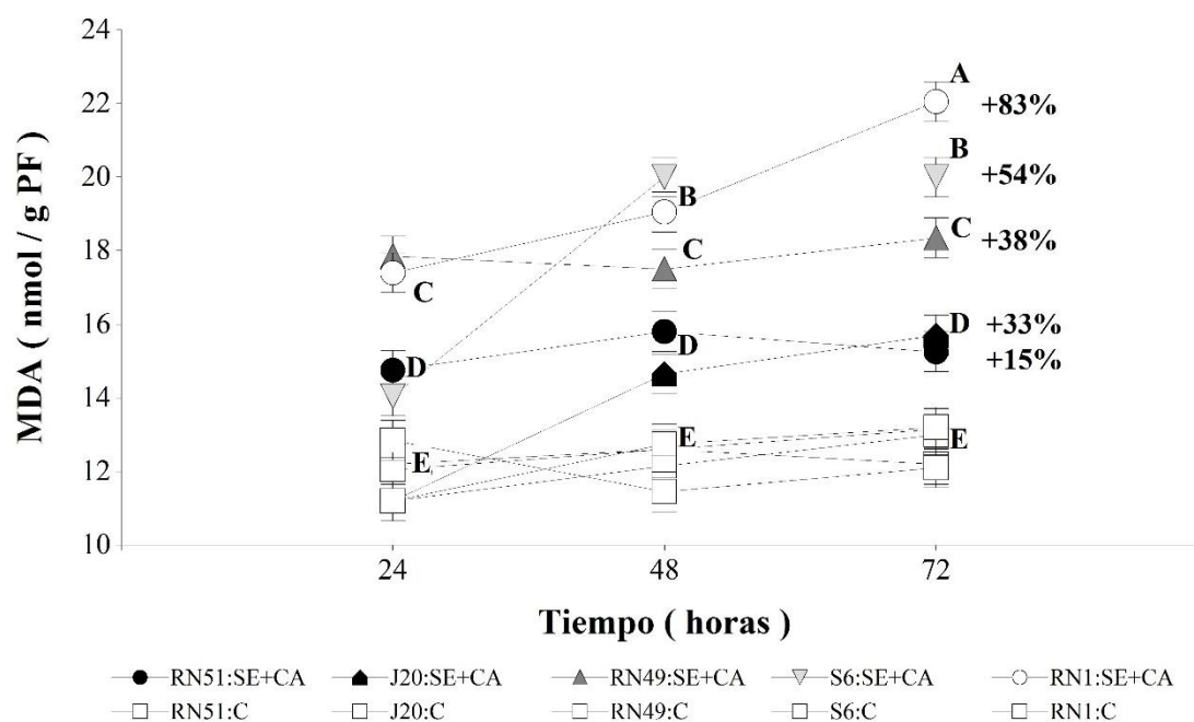
Fig. 4.2. Contenido de malondialdehído (MDA) medido a las 24, 48 y 72 horas de estrés combinado por sequía y calor en los genotipos RN51, RN1, RN49, J20 y S6. Cada punto representa el promedio de seis repeticiones. Las barras de error representan el error estándar. Letras distintas indican diferencias significativas ( p < 0,05 ). Los valores en porcentaje representan el incremento en el valor promedio del tratamiento de estrés combinado respecto del valor promedio del tratamiento control.
