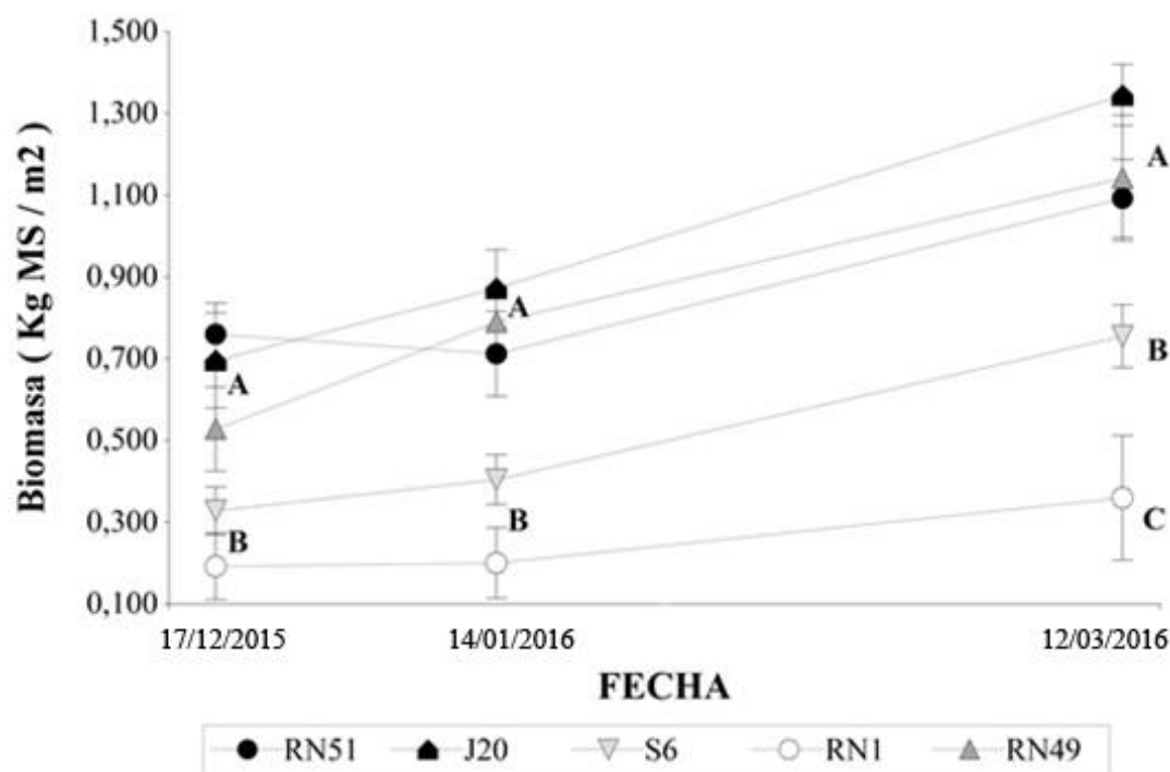
Fig. 4.8. Comparación de producciones de Biomasa en Kg de Peso seco / m 2 obtenidas en cada cosecha en el período de crecimiento del cultivo entre diciembre – marzo para los genotipos RN51, RN1, RN49, J20 y S6, evaluados en condiciones de campo en la localidad de Quilino (Noroeste de Córdoba, Argentina). Cada punto representa el valor promedio de cinco repeticiones. Las barras de error representan el error estándar. Letras distintas indican diferencias significativas ( p < 0,05 ).
