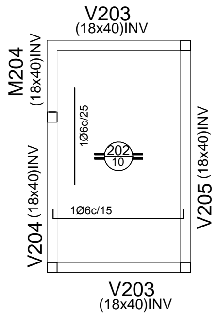
S/ ESCALERA
