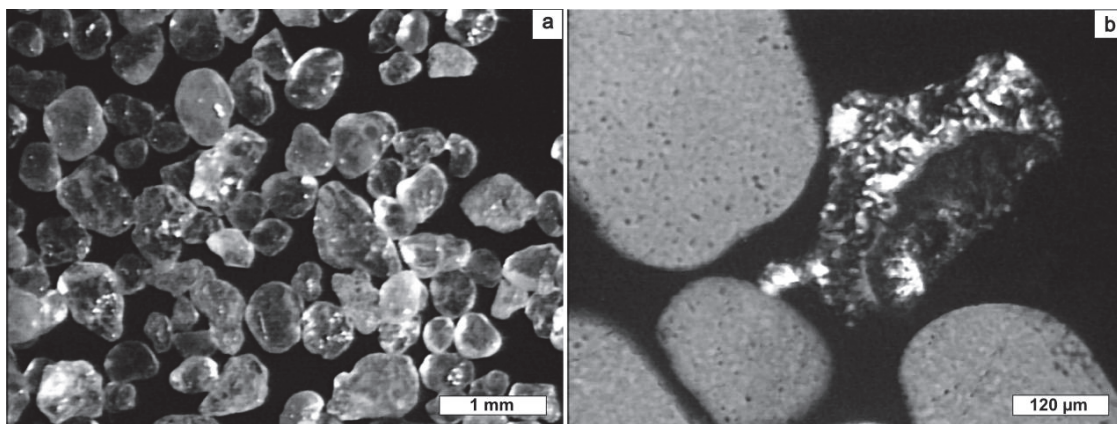
Figura 1: Material retenido en el tamiz # 60 mediante estereomicroscopio (a) y microscopio óptico de polarización (b) sobre sección delgada (nicoses cruzados).
