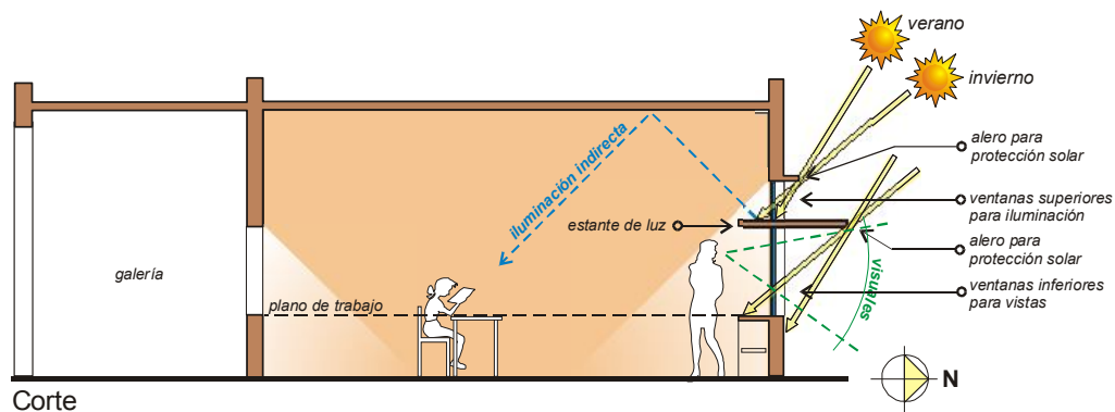
Fig. 4. Corte esquemático de ventanas con estantes de luz de la propuesta.
