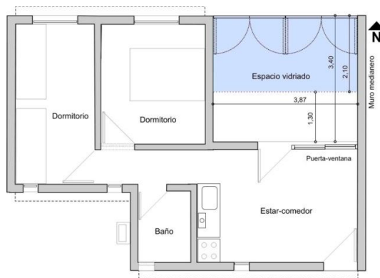
Figura 2: Planta de la vivienda con incorporación del espacio vidriado
