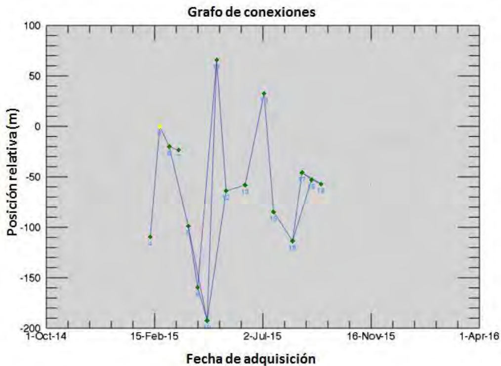
Figura 83: Gráfico de conexiones para las imágenes descendentes luego de descartar interferogramas muy ruidosos.
