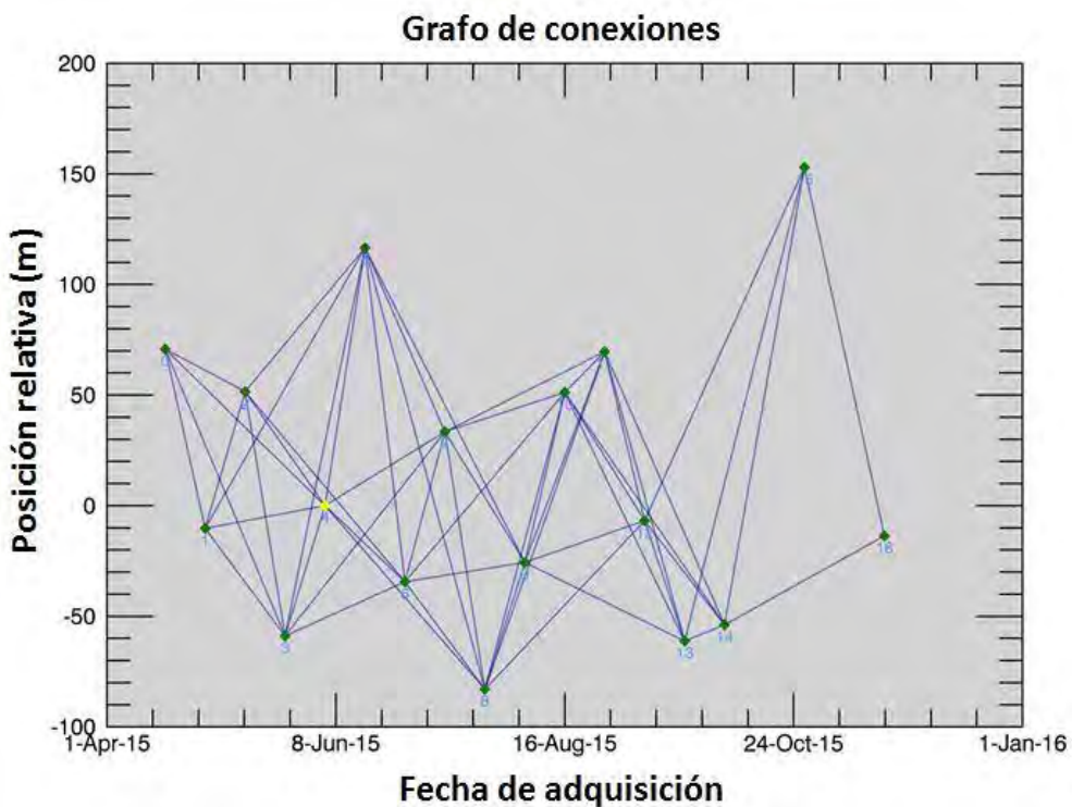
Figura 76: Gráfico de conexiones para imágenes Sentinel-1A Ascendentes, mostrando todas las combinaciones posibles empleando un umbral de B_{TEMP} = 48 días.
