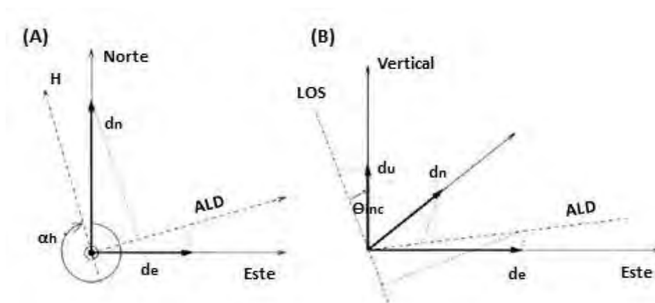
Figura 45: Proyección de los tres componentes de deformación sobre la línea de vista del sensor. (A) muestra la vista desde arriba de los componentes Este y Norte proyectados sobre la dirección de mirada en azimut (ALD), perpendicular a la trayectoria del satélite indicada con \alpha_h . (B) muestra un esquema 3D incluyendo la proyección del componente vertical a la línea de vista del sensor empleando el ángulo de incidencia (Hanssen, 2002, pág. 163).
