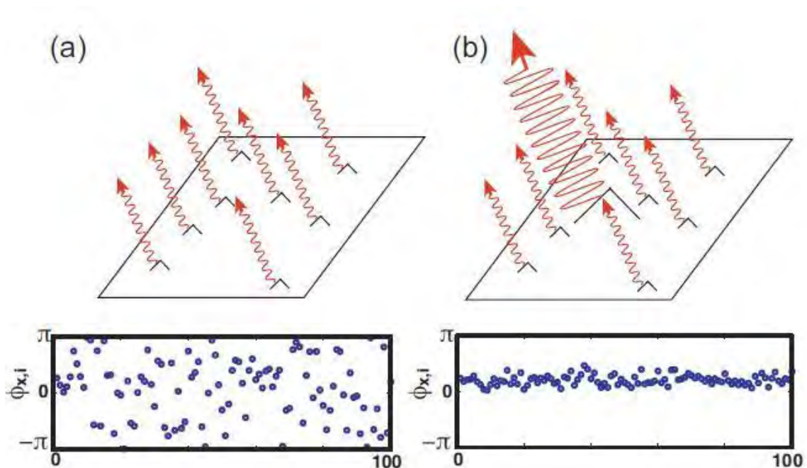
Figura 34: Simulaciones de fase para un píxel con dispersores distribuidos (a) y otro con un dispersor dominante o permanente (b). Los gráficos respectivos muestran las simulaciones de fase en 100 iteraciones (Hooper, 2006).
