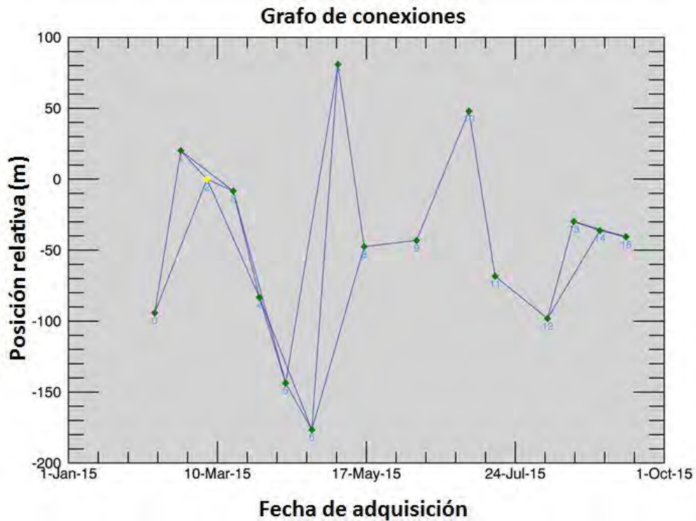
Figura 75: Gráfico de conexiones para imágenes Sentinel-1A Descendentes, mostrando todas las combinaciones posibles empleando un umbral de B_{TEMP} = 24 días.
