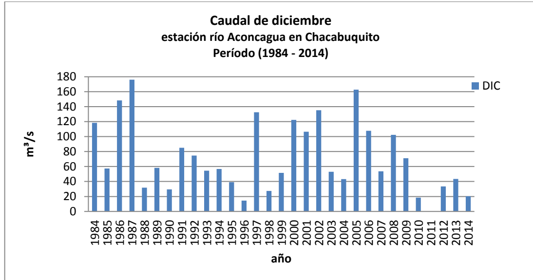
Gráfico 10: Caudal de diciembre, estación río Aconcagua en Chacabuquito
