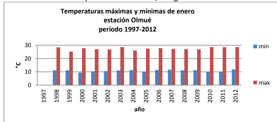
Gráfico 53: Temperaturas máximas y mínimas de enero, estación Olmué
