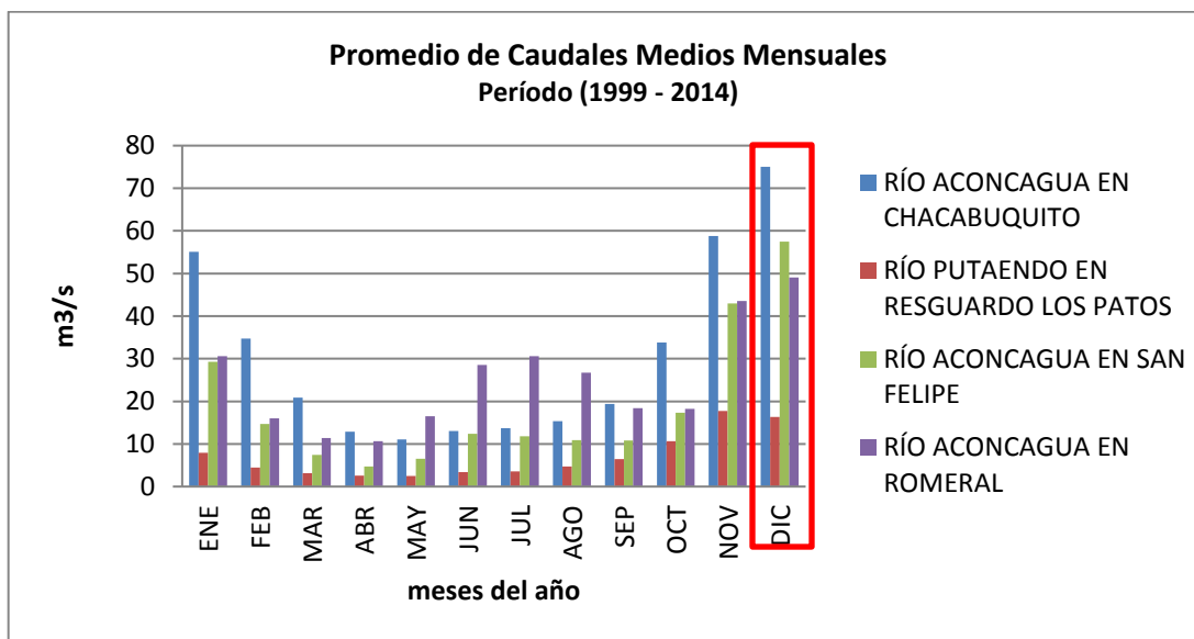
Gráfico 9: Promedio caudales mensuales en las estaciones fluviométricas de la cuenca del río Aconcagua
