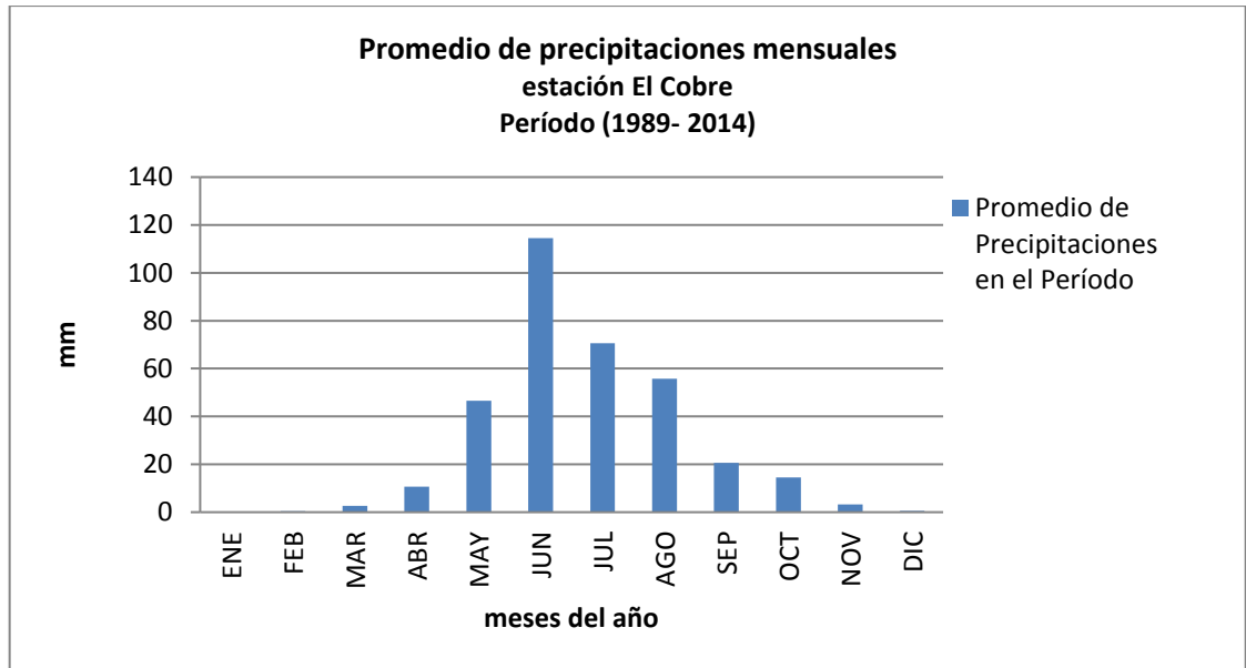
Gráfico 14: Promedio de precipitaciones mensuales, estación El Cobre
