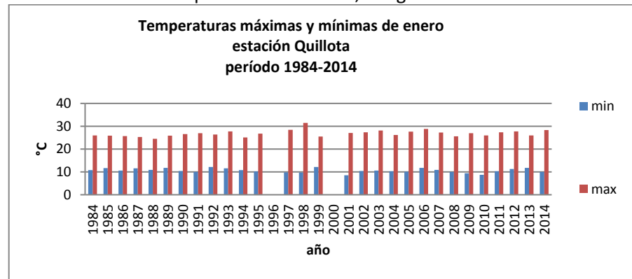
Gráfico 56: Temperaturas máximas y mínimas de enero, estación Quillota
