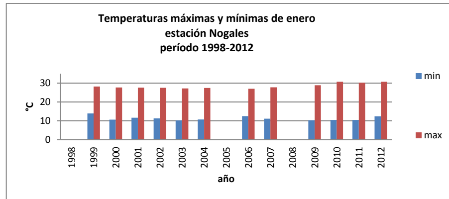
Gráfico 41: Temperaturas máximas y mínimas de enero, estación Nogales
