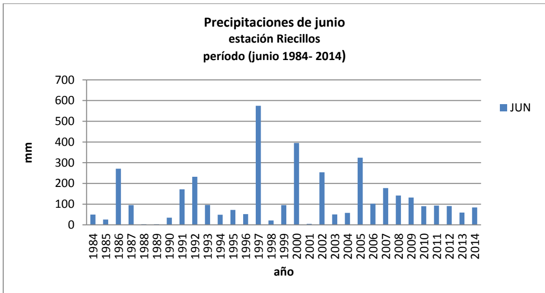
Gráfico 26: Precipitaciones de junio, estación Riecillos Fuente: elaboración propia.
