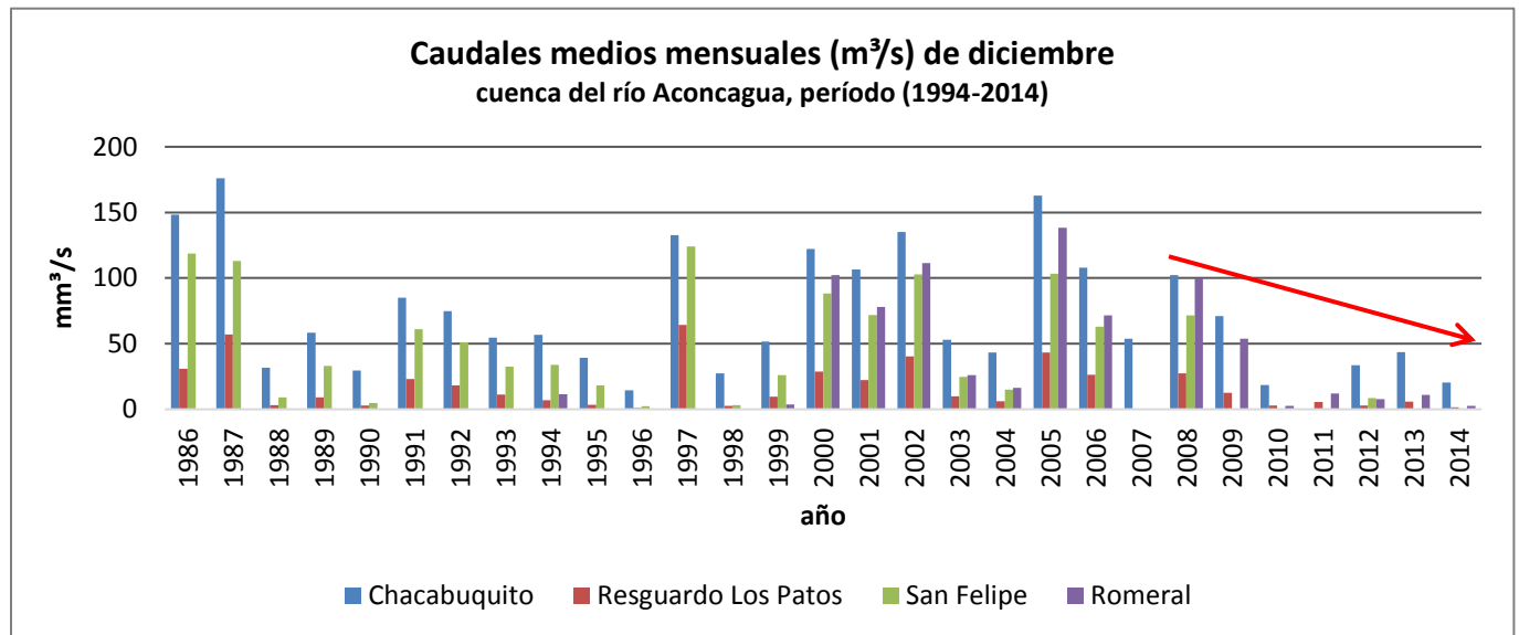
Gráfico 92: Caudales medios mensuales (m 3 /s) de diciembre en la cuenca de río Aconcagua
