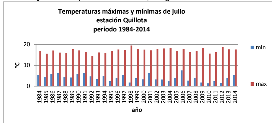
Gráfico 55: Temperaturas máximas y mínimas de julio, estación Quillota
