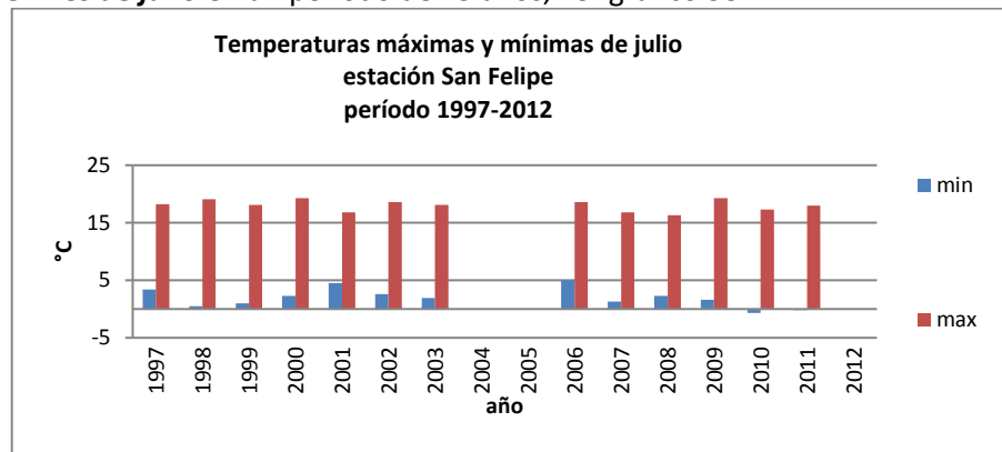
Gráfico 58: Temperaturas máximas y mínimas de julio, estación San Felipe
