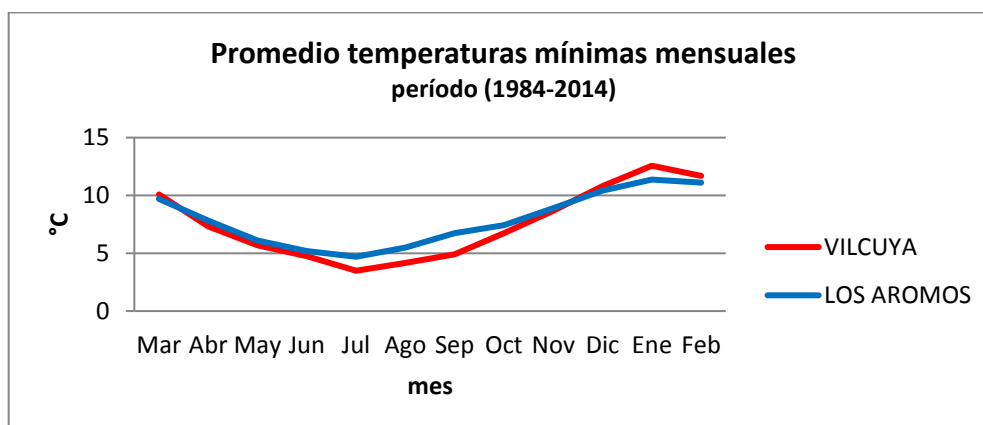
Gráfico 83: Promedio temperaturas mínimas mensuales en la cuenca del río Aconcagua
