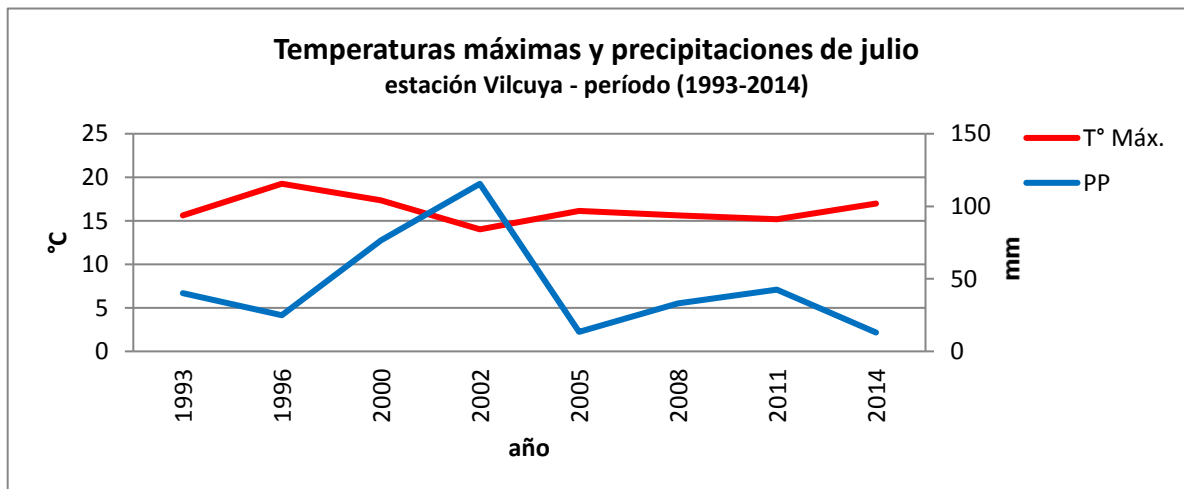
Gráfico 87: Temperaturas máximas y precipitaciones de julio en la estación Vilcuya Fuente: elaboración propia.
