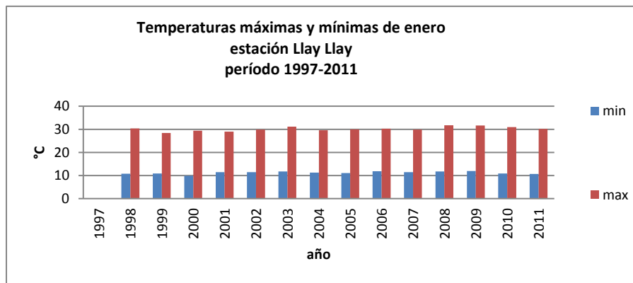
Gráfico 47: Temperaturas máximas y mínimas de enero, estación Llay Llay
