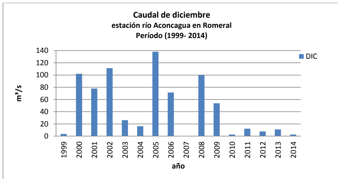
Gráfico 11: Caudal de diciembre, estación río Aconcagua en Romeral
