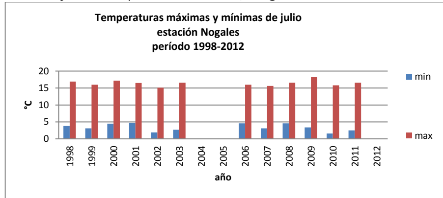
Gráfico 40: Temperaturas máximas y mínimas de julio, estación Nogales
