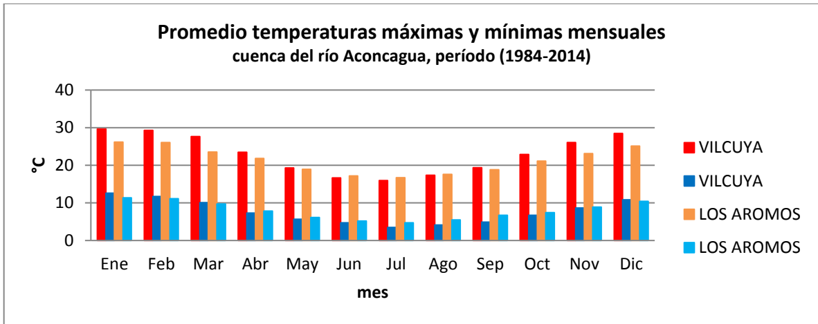
Gráfico 84: Promedio temperaturas máximas y mínimas mensuales en la cuenca del río Aconcagua Fuente: elaboración propia.
