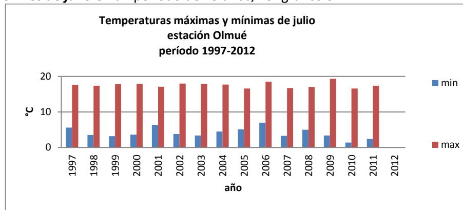
Gráfico 52: Temperaturas máximas y mínimas de julio, estación Olmué
