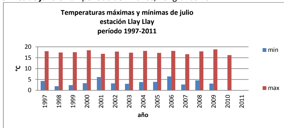
Gráfico 46: Temperaturas máximas y mínimas de julio, estación Llay Llay
