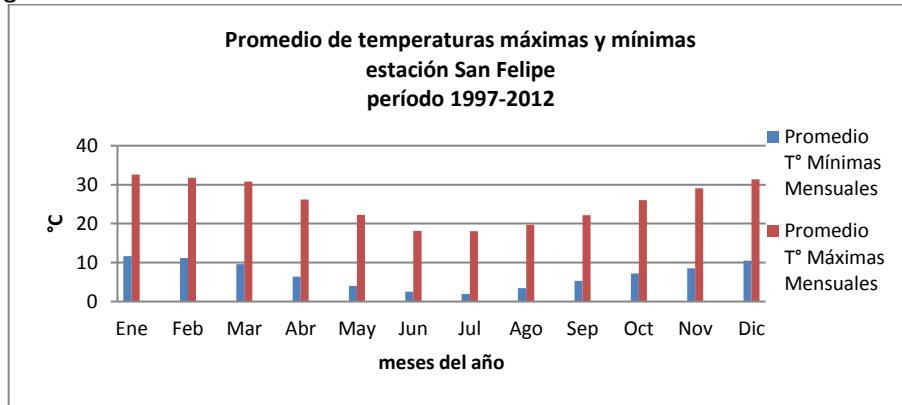
Gráfico 57: Promedios de temperaturas máximas y mínimas, estación San Felipe
