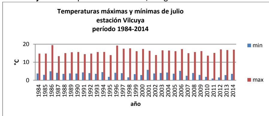
Gráfico 61: Temperaturas máximas y mínimas de julio, estación Vilcuya
