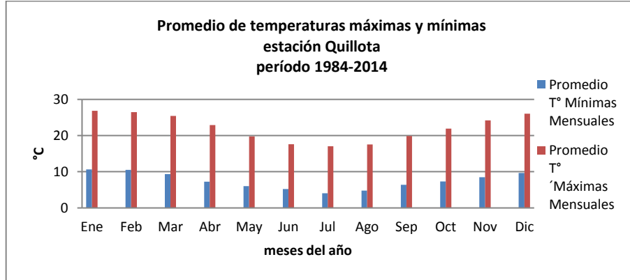
Gráfico 54: Promedios de temperaturas máximas y mínimas, estación Quillota
