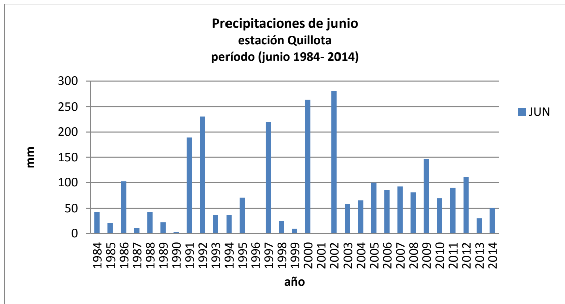
Gráfico 21: Precipitaciones de junio, estación Quillota
