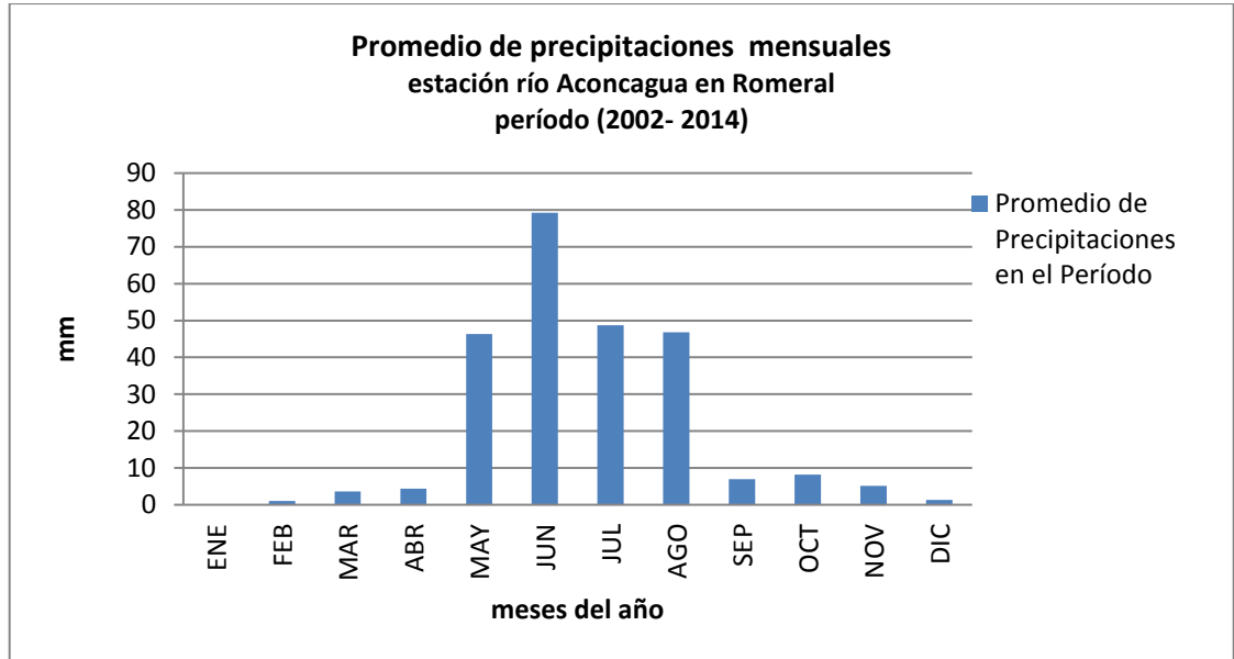
Gráfico 29: Promedio de precipitaciones mensuales, estación río Aconcagua en Romeral
