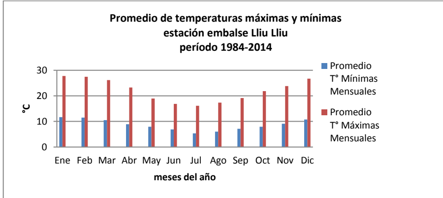
Gráfico 36: Promedios de temperaturas máximas y mínimas, estación embalse Lliu Lliu
