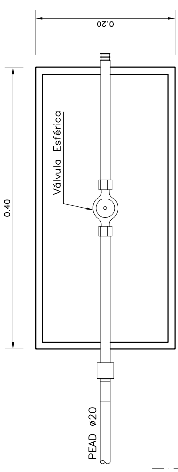
PLANTA POR A-A
