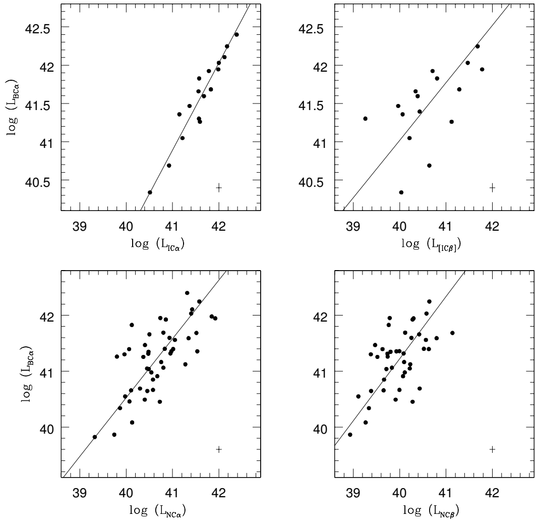
Figura 34: Luminosidad de la componente ancha (BC) de H\alpha comparada con la luminosidad de: la componente intermedia IC de H\alpha (arriba a la izquierda), IC\beta (arriba a la derecha), la componente delgada NC\alpha (abajo a la izquierda) y NC\beta (abajo a la derecha). Todos los valores de las luminosidades están en unidades de (\text{erg s}^{-1}) . Las líneas sólidas representan los mejores ajustes para los datos. Barras de errores típicas de 0.06 dex se indican en cada gráfico.
