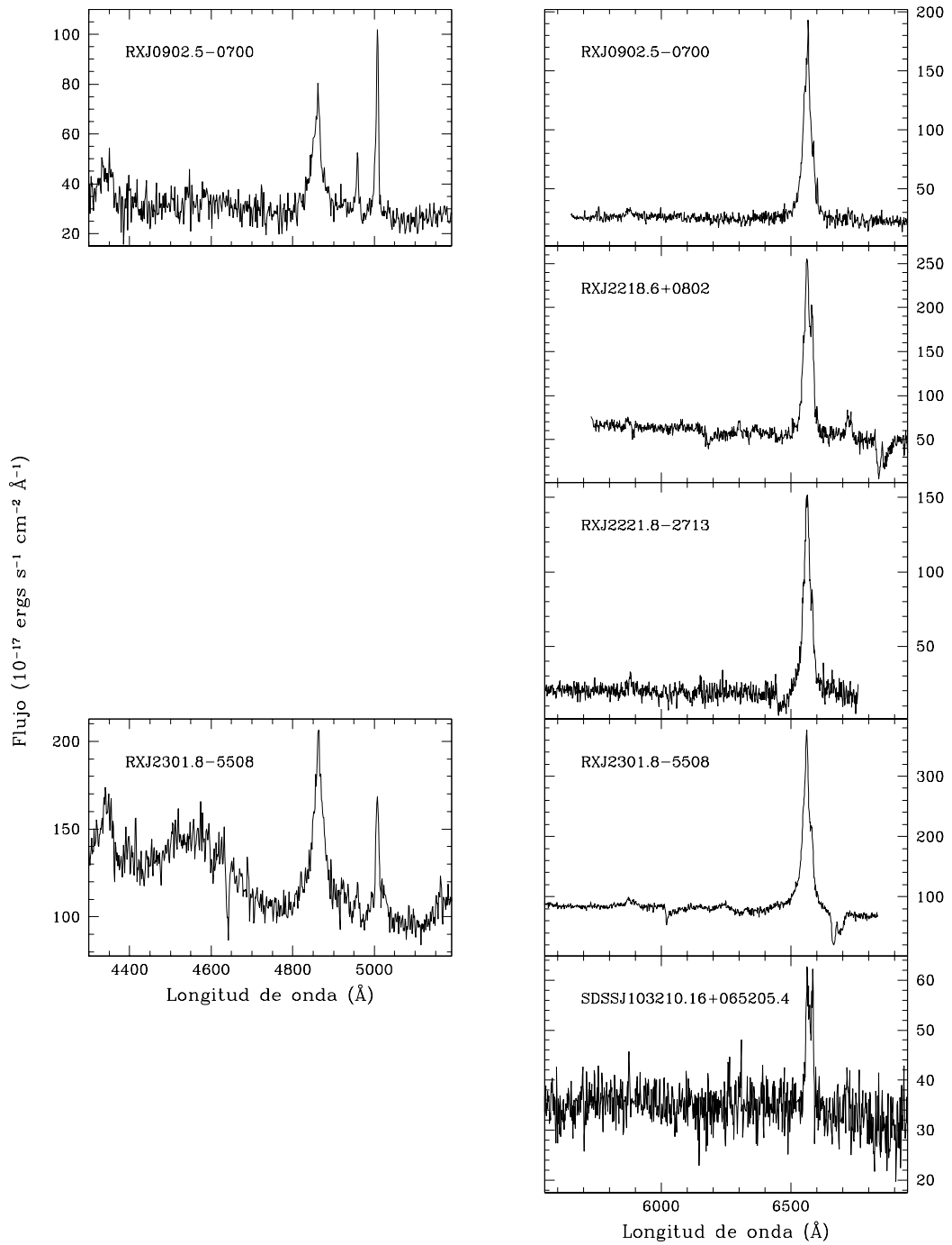
Figura 48: Espectros observados desde CASLEO en los rangos 4300\text{\AA} - 5200\text{\AA} y 5600\text{\AA} - 6900\text{\AA} . La ordenada está en unidades de 10^{-17} erg cm^{-2} s^{-1} \text{\AA}^{-1} y los espectros están en "rest-frame".
