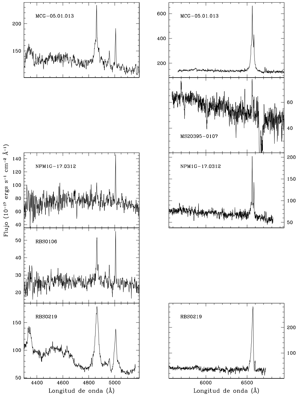
Figura 46: Espectros observados desde CASLEO en los rangos 4300Å - 5200Å y 5600Å - 6900Å. La ordenada está en unidades de 10^{-17} \text{ erg cm}^{-2} \text{ s}^{-1} \text{ Å}^{-1} y los espectros están en "rest-frame".
