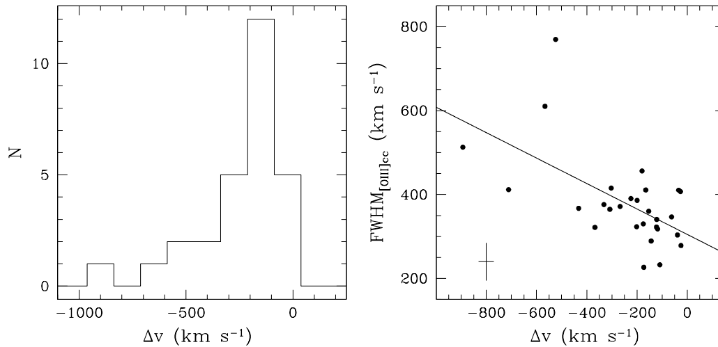
Figura 30: Histograma de \Delta v (izquierda) y relación entre \Delta v y \text{FWHM}_{[\text{OIII}]cc} (derecha) para las 28 galaxias de la muestra que presentan asimetrías en [OIII] \lambda 5007. La línea sólida en el panel derecho representa el mejor ajuste obtenido para estos datos. \Delta v y \text{FWHM}_{[\text{OIII}]cc} están en unidades de \text{km s}^{-1} . Se muestra además una barra de error típica.
