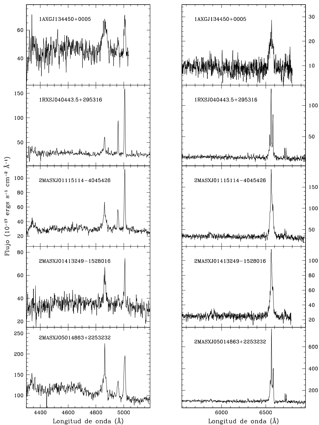
Figura 41: Espectros observados desde CASLEO en los rangos 4300 \text{\AA} - 5200 \text{\AA} y 5600 \text{\AA} - 6900 \text{\AA} . La ordenada está en unidades de 10^{-17} \text{ erg cm}^{-2} \text{ s}^{-1} \text{ \AA}^{-1} y los espectros están en "rest-frame".
