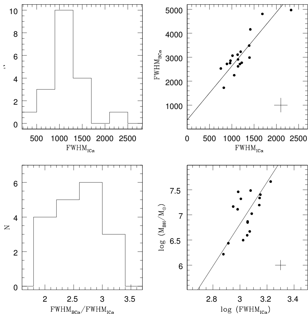
Figura 27: Histograma de los valores del FWHM la componente intermedia IC de H \alpha (panel superior izquierdo), relación entre el FWHM de la componente ancha BC de H \alpha (panel superior derecho), histograma del cociente \text{FWHM}_{\text{BC}}/\text{FWHM}_{\text{IC}} (panel inferior izquierdo) y relación entre el FWHM de IC y la masa de los agujeros negros (panel inferior derecho). Todos los valores de FWHM están en \text{km s}^{-1} y fueron desafectados por el ancho instrumental. Se muestran las barras de errores típicas. Las líneas sólidas representan el mejor ajuste de los datos.
