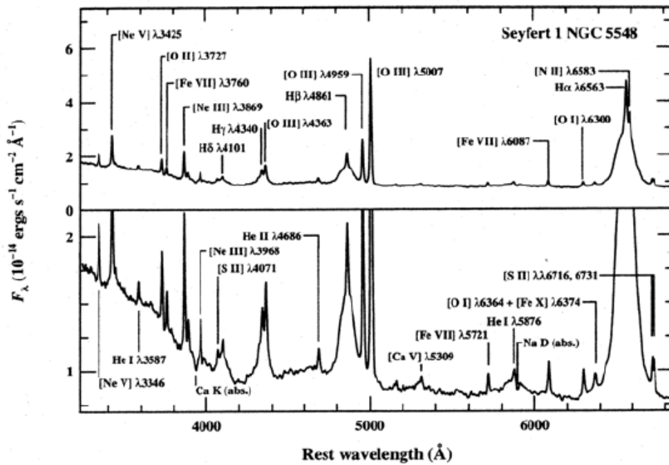
Figura 6: Espectro óptico de la galaxia Seyfert 1 NGC5548. El espectro muestra las líneas anchas de emisión de Balmer H \alpha , H \beta , H \gamma and H \delta y líneas prohibidas angostas como por ejemplo [OIII], [OII] y [NeIII]. Espectro obtenido por A. V. Filippenko en el Observatorio Lick (Estados Unidos).
