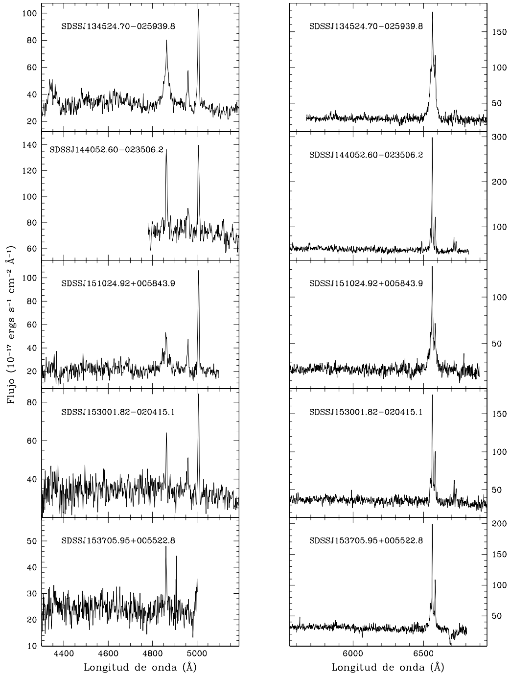
Figura 49: Espectros observados desde CASLEO en los rangos 4300Å - 5200Å y 5600Å - 6900Å. La ordenada está en unidades de 10^{-17} \text{ erg cm}^{-2} \text{ s}^{-1} \text{ Å}^{-1} y los espectros están en "rest-frame".
