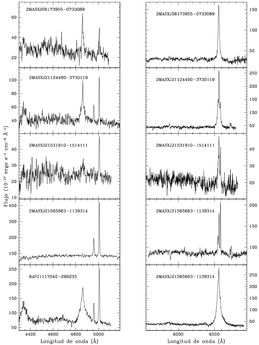
Figura 42: Espectros observados desde CASLEO en los rangos 4300\text{\AA} - 5200\text{\AA} y 5600\text{\AA} - 6900\text{\AA} . La ordenada está en unidades de 10^{-17} \text{ erg cm}^{-2} \text{ s}^{-1} \text{ \AA}^{-1} y los espectros están en "rest-frame".
