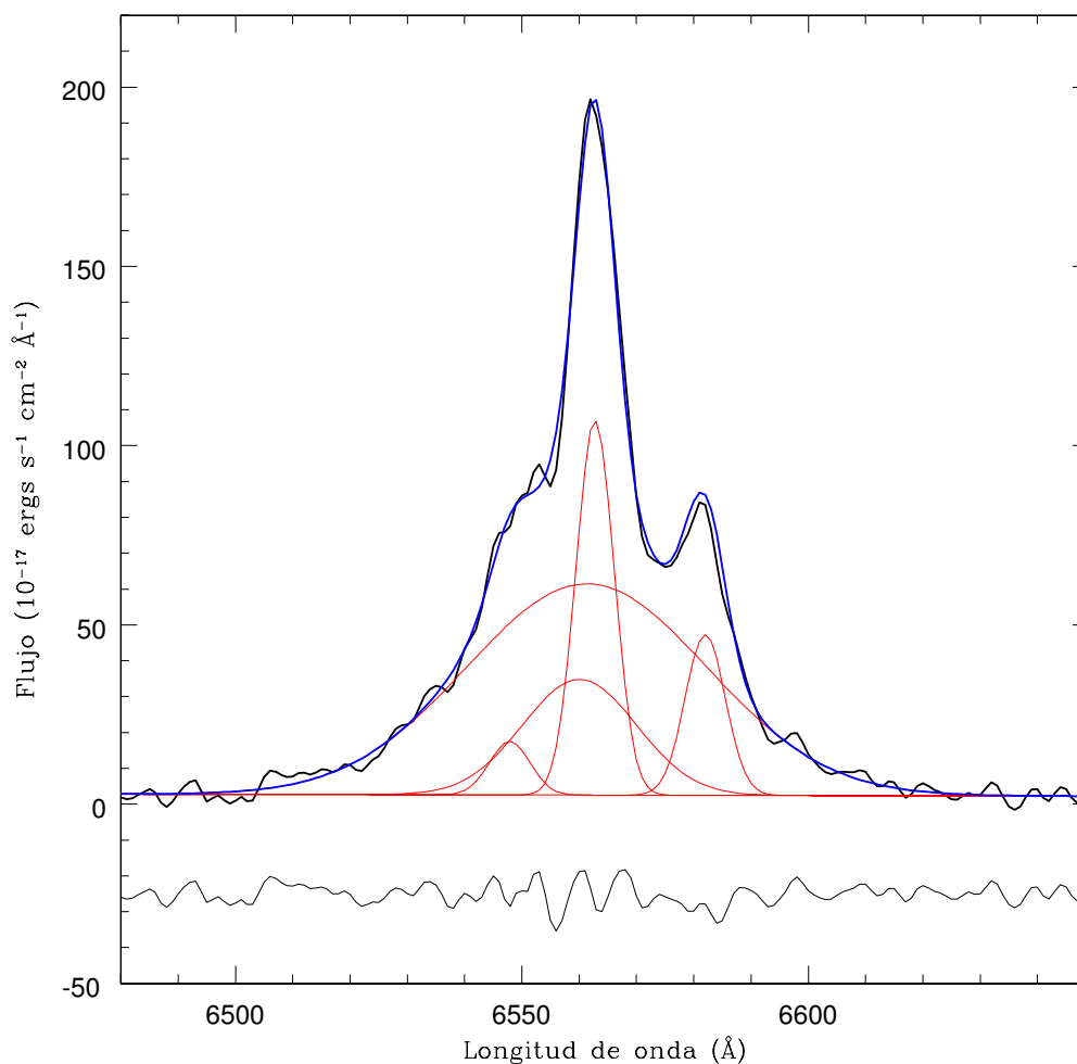
Figura 18: Descomposición de gaussianas realizada en el marco de este trabajo para el perfil H\alpha + [NII]\lambda\lambda 6549, 6584 del espectro de la galaxia 2MASX J21124490-3730119. El espectro observado se ve en negro, las componente ancha, delgada e intermedia de H\alpha , además de las dos líneas correspondientes a [NII]\lambda\lambda 6549, 6584 se ven en color rojo. El ajuste total (suma de todas las componentes) se ve en azul. El residuo (diferencia entre el espectro observado y el ajuste realizado) se muestra en negro en la parte inferior de la figura.
