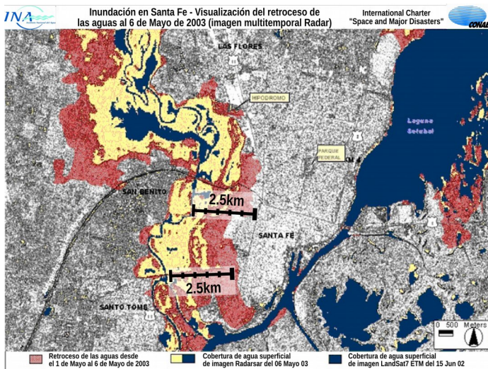
Fig.15: Imagen SAR (Radarsat) que muestra las zonas inundadas en la ciudad de Santa Fe en abril/mayo 2003. [Fuente: https://disasterscharter.org ]
