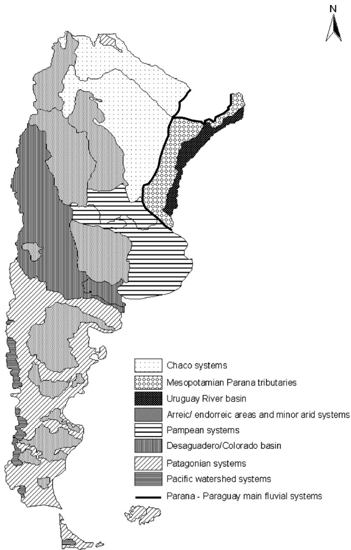
Imagen 1: Esquema de los sistemas hídricos en Argentina [8].
