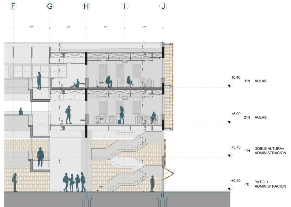
CORTE
