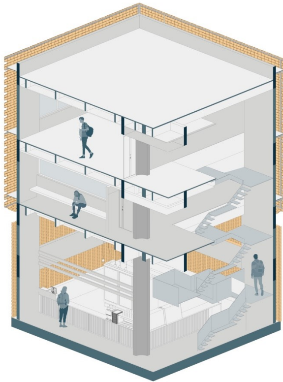
AXONOMETRICA
