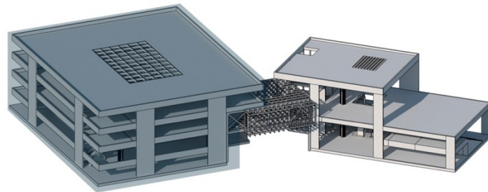
Esquema Estructural
