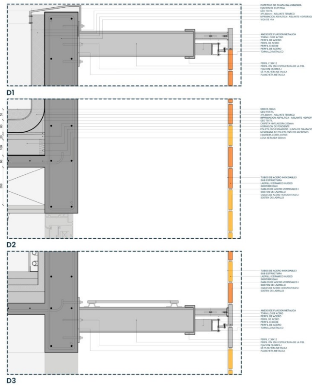
DETALLES
