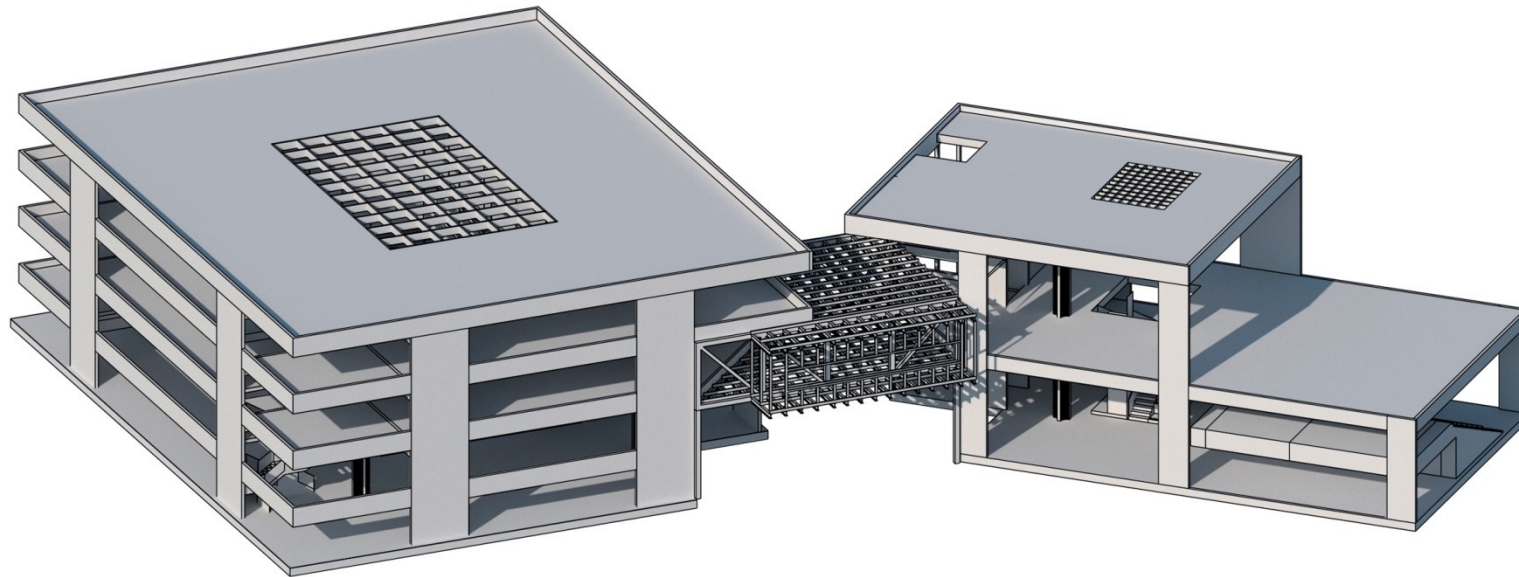
Esquema Estructural
