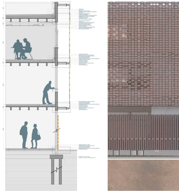
CORTE ESC: 1.20
