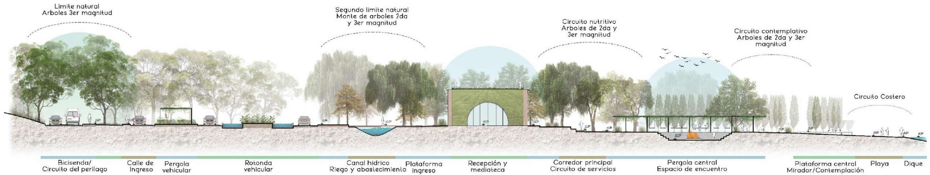
CORTE 1. 1:200 - tunel de platano - Ingreso - monte - vacio central - playa.
