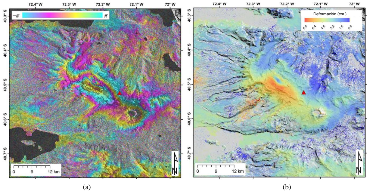
Figura 4.1: imágenes InSar abril y mayo 2011. (a) interferograma wrapped, (b) mapa de deformación.
