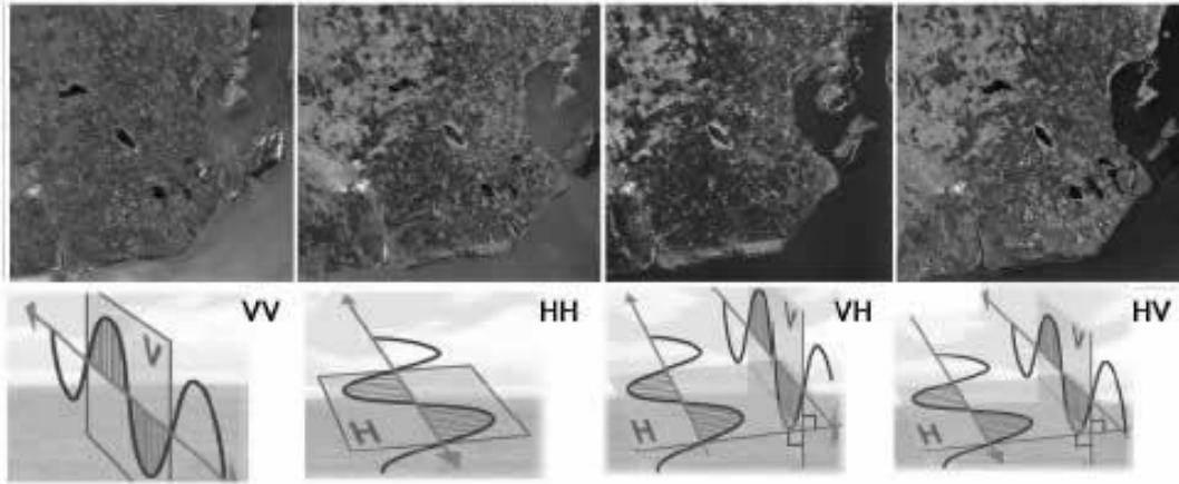
Figura 2.8: imágenes SAR de RADARSAT-2 del sur de la provincia de Buenos Aires adquiridas con distintas configuraciones de polarización paralela y cruzada (Proyecto SOAR). Fuente: Marchionni et al., 2014.
