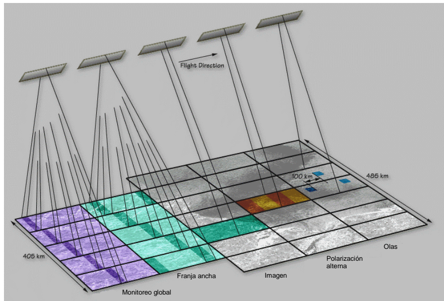
Figura 3.1: modos operativos Envisat. Fuente: ESA, 2007.
