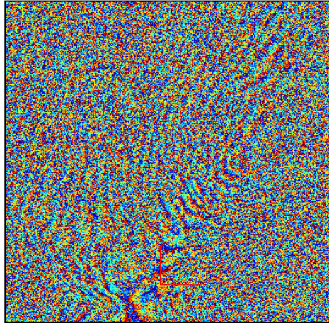
Figura 3.4: interferograma (Base). Área de ejemplo de una superficie aproximada de 9 x 9 km.
