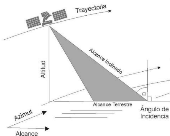
Figura 2.9: geometría de la observación de un sistema de radar (modificado Raney, 1992). Fuente: CCRS, 2014.
