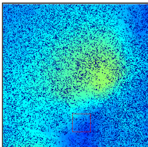
Figura 3.9: desenrollado de la fase “ unwrapping ”. Área de ejemplo de una superficie aproximada de 9 x 9 km.
