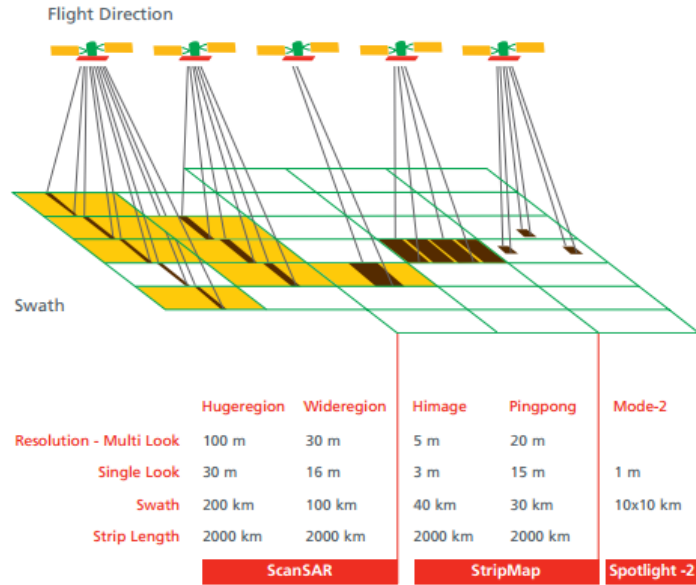
Figura 3.11: modo de adquisición imagen COSMO- SkyMed. Fuente: E-GEOS, 2015.
