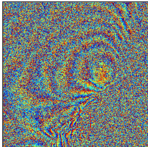
Figura 3.5: interferograma aplanado “flattening”. Área de ejemplo de una superficie aproximada de 9 x 9 km.
