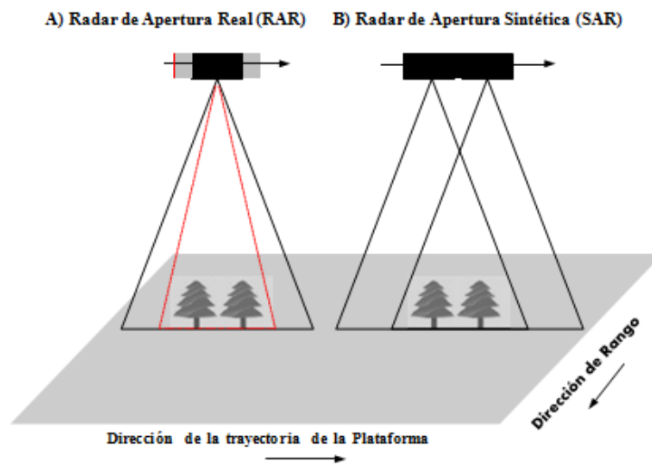
Figura 2.10: RAR y SAR. Fuente: De Ruyt, 2013.
