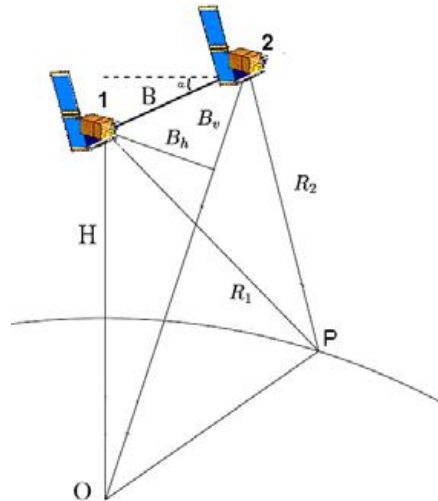
Figura 2.14: componentes de la base vertical y horizontal. Fuente: C. Rebelo 2007.
