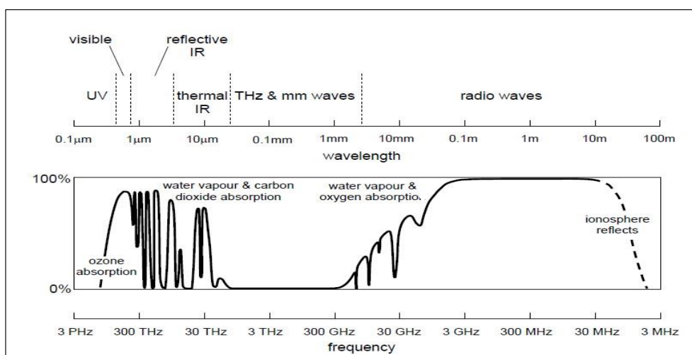
Figura 2.2: espectro electromagnético e interacción de los tipos de frecuencias con los diferentes componentes de la atmósfera. Fuente: J. Richards, 2009.
