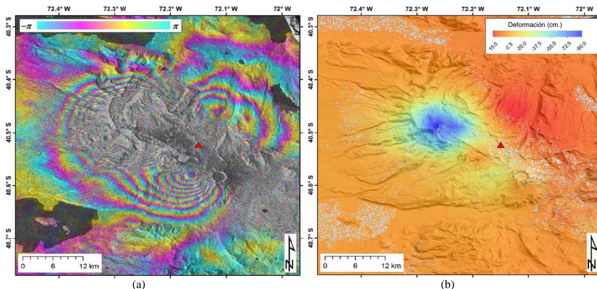
Figura 4.2: imágenes InSar mayo y junio 2011. (a) interferograma wrapped, (b) mapa de deformación.
