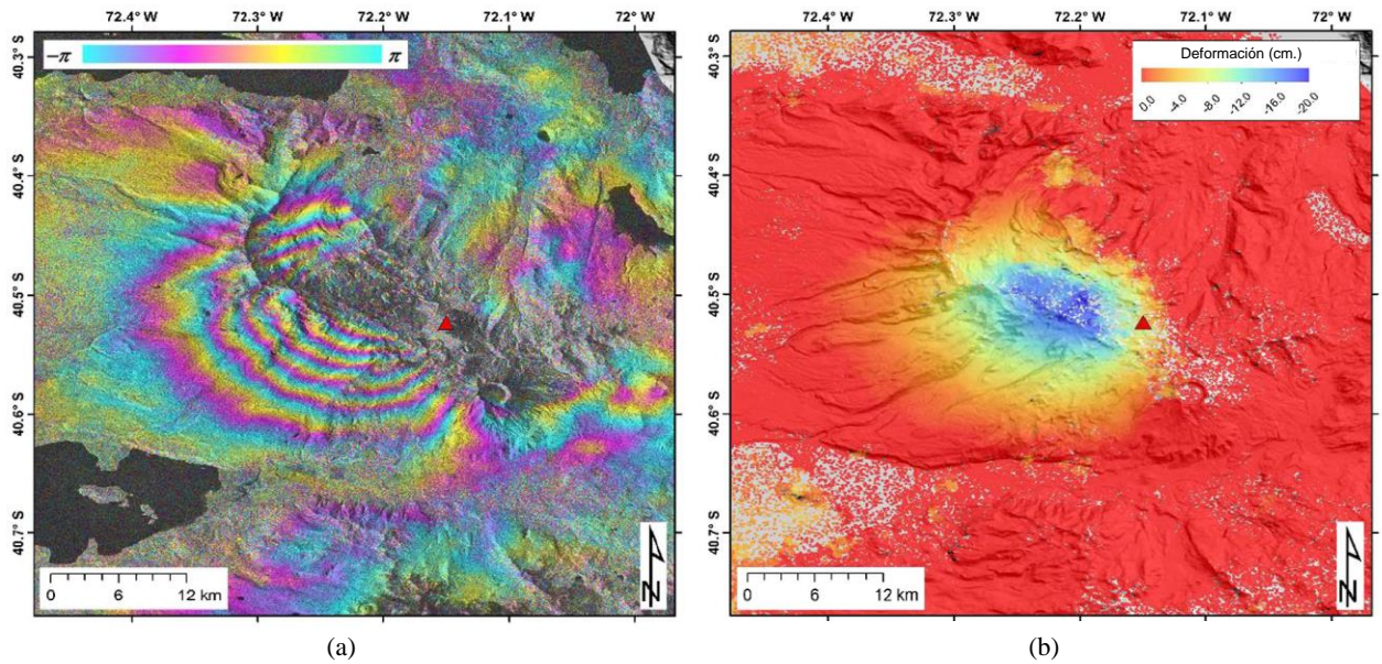
Figura 4.4: imágenes InSar octubre y diciembre 2011. (a) interferograma wrapped, (b) mapa de deformación.
