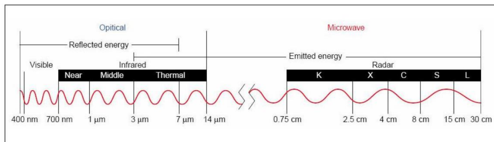
Figura 2.7: espectro electromagnético. Dominio de frecuencias de las microondas y bandas. Fuente: Marchionni et al., 2014.
