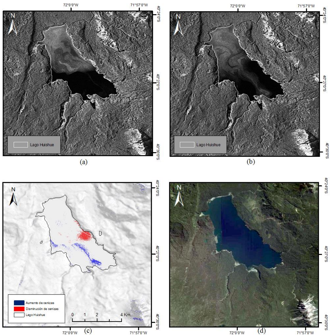
Figura 4.7: imagen COSMO-SkyMed (a) 19/06/2011, (b) 26/06/2011, (c) imagen de cambios entre las dos fechas (d) imagen óptica de referencia google earth 26/02/2015.
