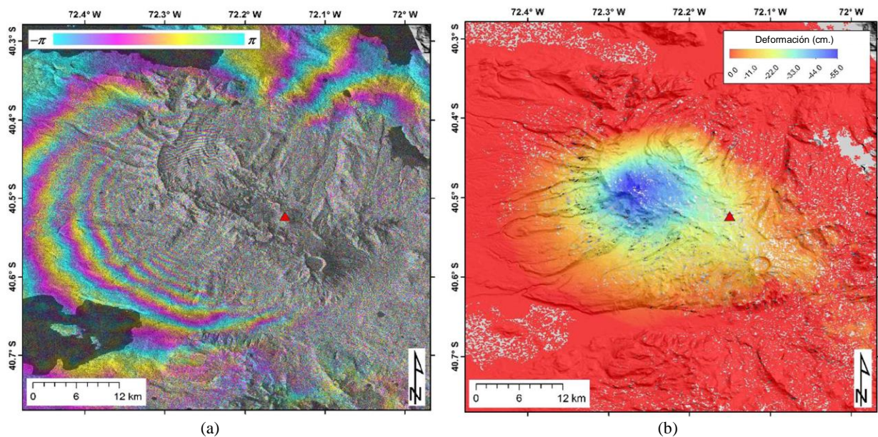
Figura 4.3: imágenes InSar junio y julio 2011. (a) interferograma wrapped, (b) mapa de deformación.
