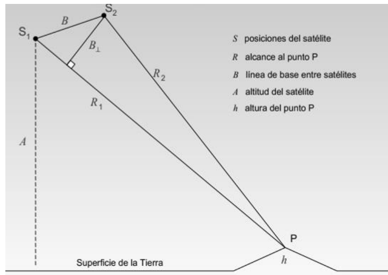
Figura 2.12: geometría de un satélite técnica interferometría SAR. Fuente: CCRS, 2014.
