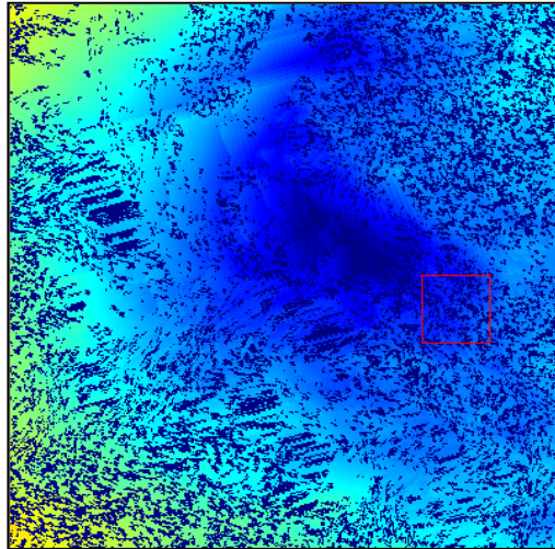
Figura 3.10: imagen de deformación. Área de ejemplo de una superficie aproximada de 9 x 9 km.
