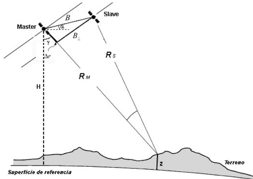
Figura 2.13: configuración geométrica de la interferometría. Fuente: C. Rebelo 2007.
