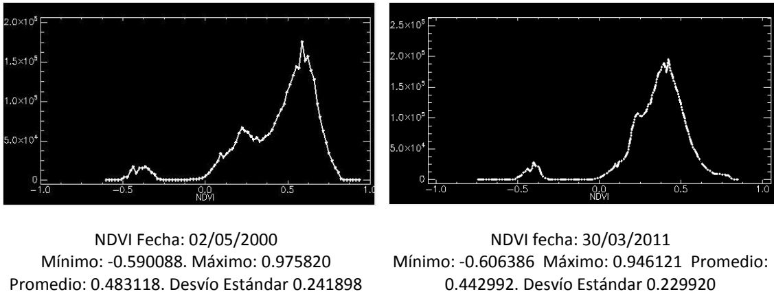
Figura 26. Estadísticos básicos e histogramas de frecuencia de los índices de vegetación normalizados para las diferentes fechas
