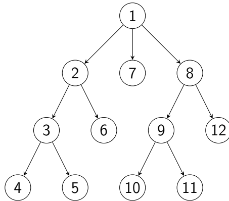
Figura 2.10: Orden en que los nodos del árbol son recorridos usando DFS
