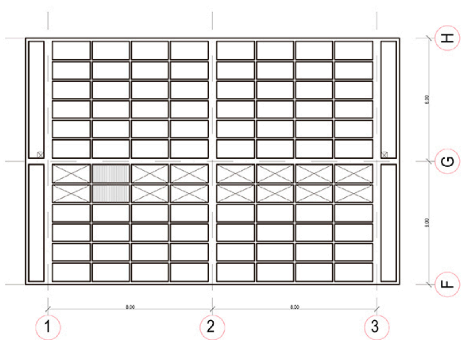
P. ESTRUC. BAJA ESC.1:200
