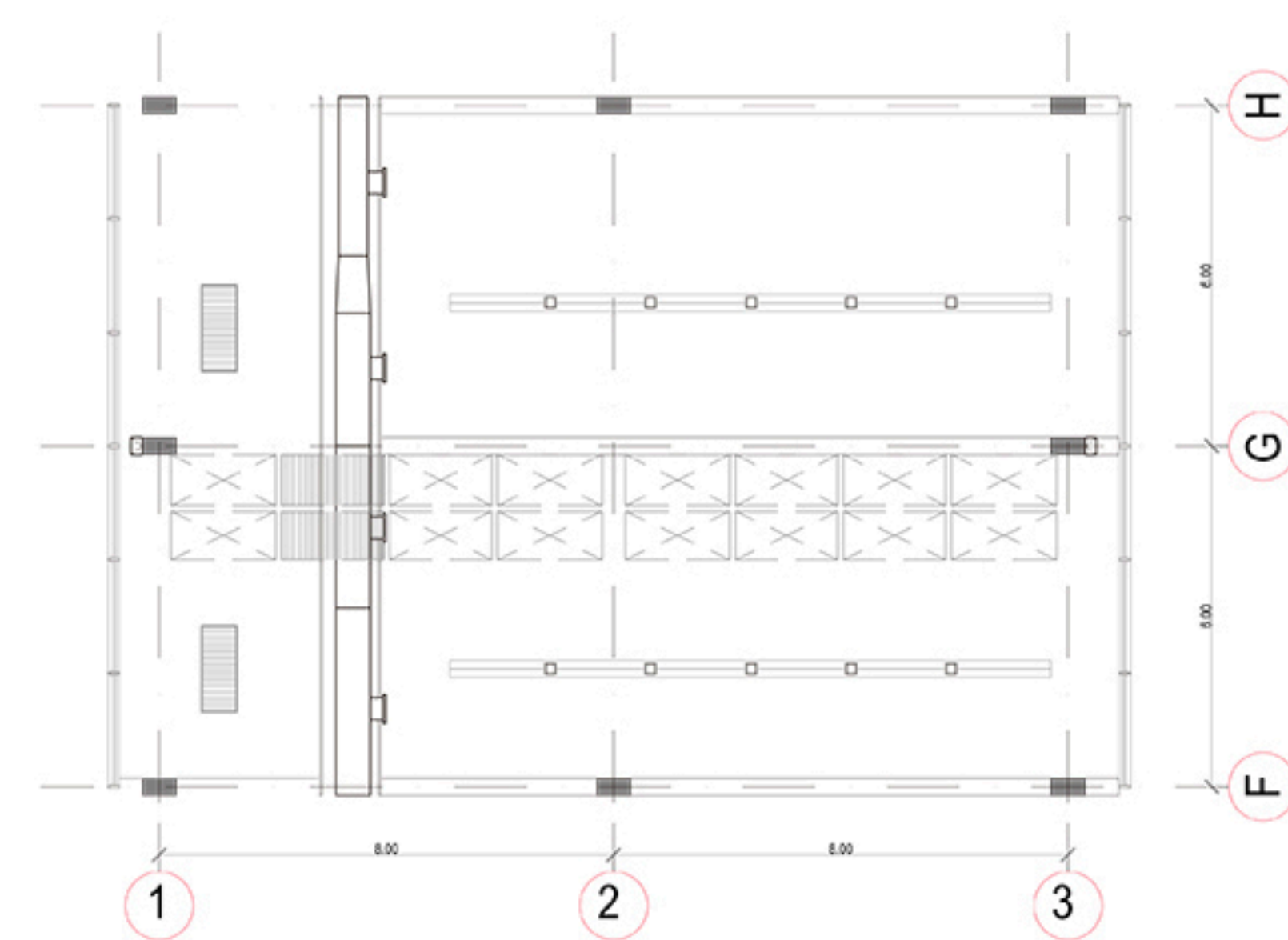
P. ESTRUC. FUNDACIÓN ESC.1:200
