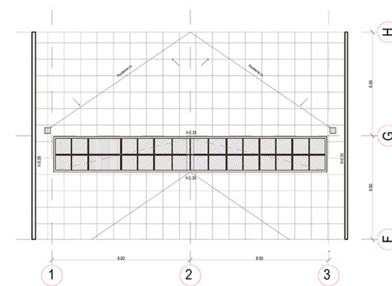
P. ESTRUC. ALTA ESC.1:200
