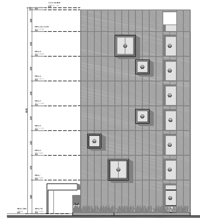
VISTA LATERAL 1
