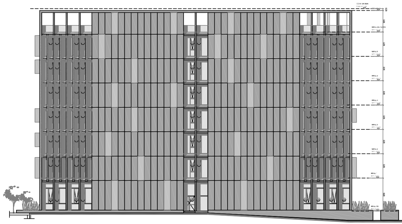
VISTA POSTERIOR
