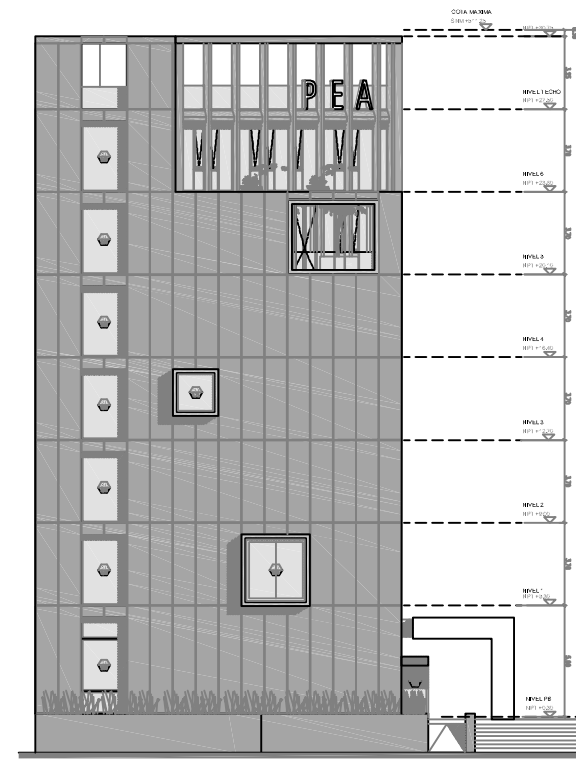
VISTA LATERAL 2
