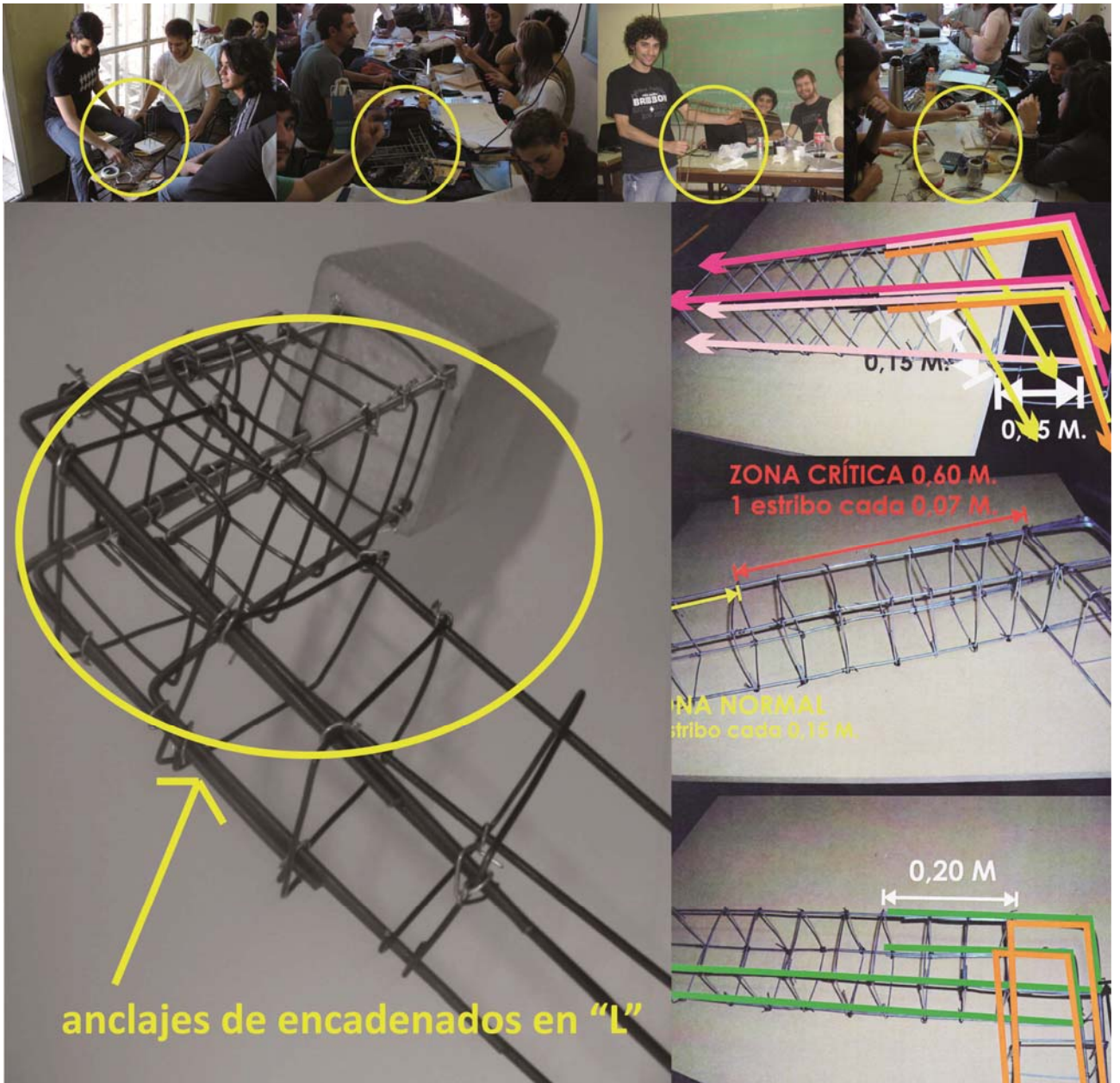
Figura 12 – Maqueta de encadenado / Trabajo en taller
