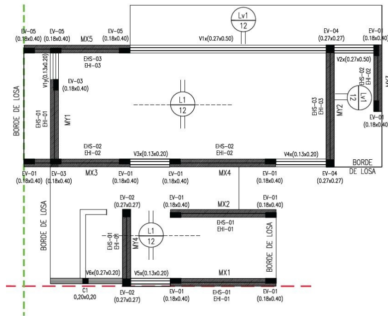
Figura 7 – Diseño de encadenados
