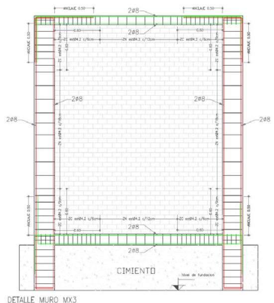
Figura 9 – Detalle de muro
