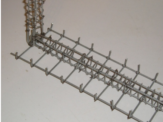
Figura 3 - Encadenado inferior dentro de una plantilla de fundación.
