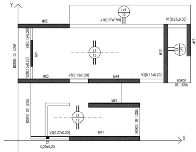
Figura 2 – Mecanismo estructural propuesto
