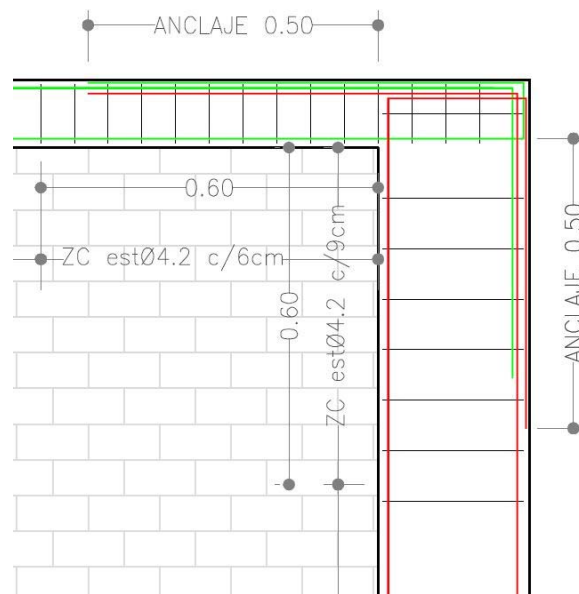
Figura 10 – Detalle de nudo
