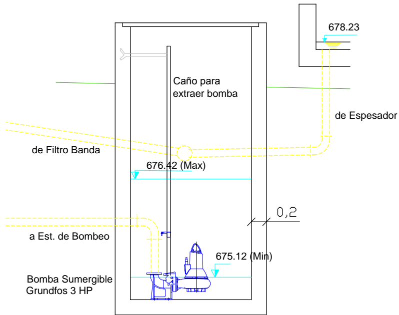
CORTE
