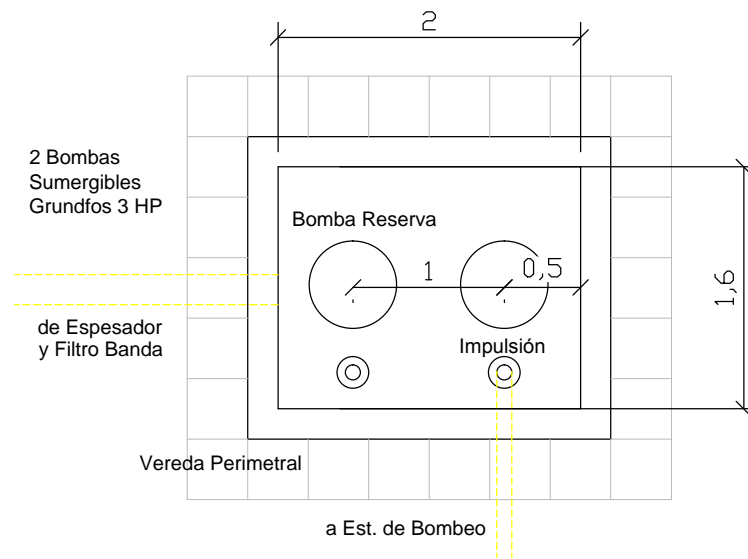
PLANTA
