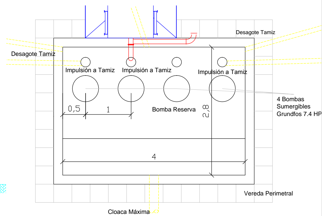
PLANTA
