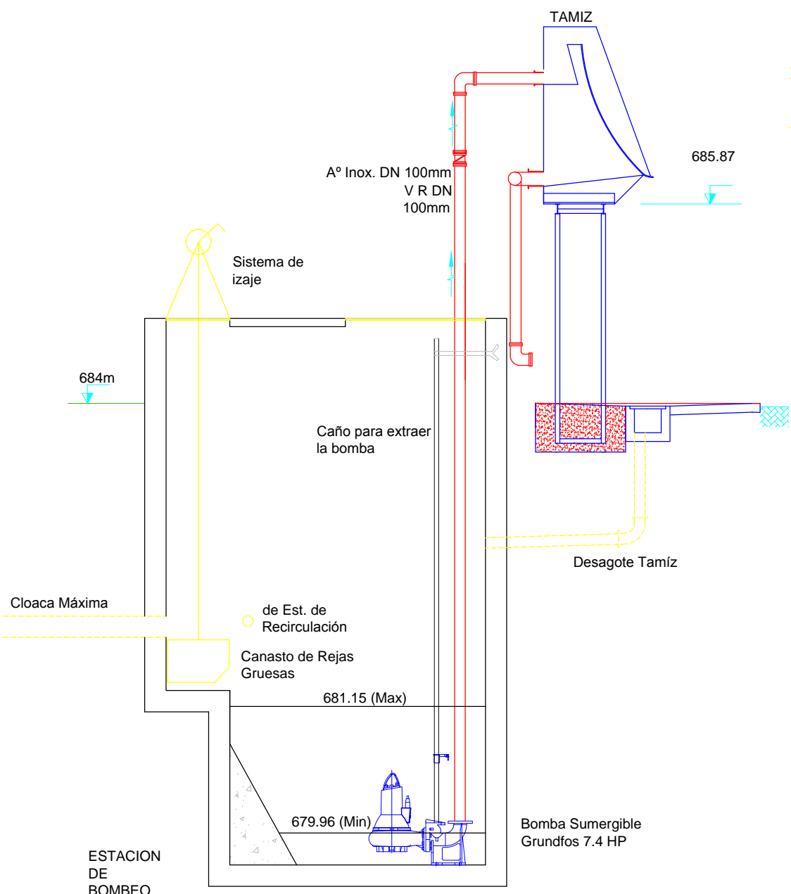
CORTE
