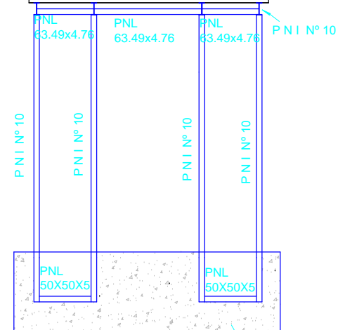
CORTE B-B
