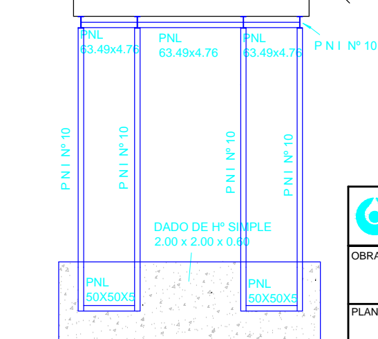
CORTE A-A
