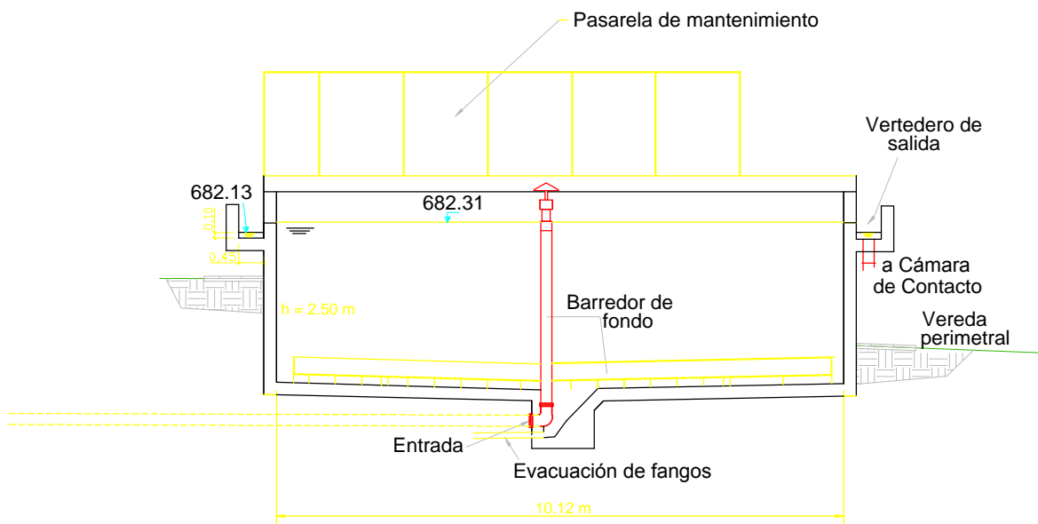
CORTE
