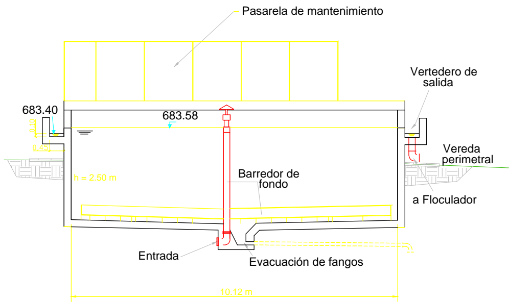
CORTE
