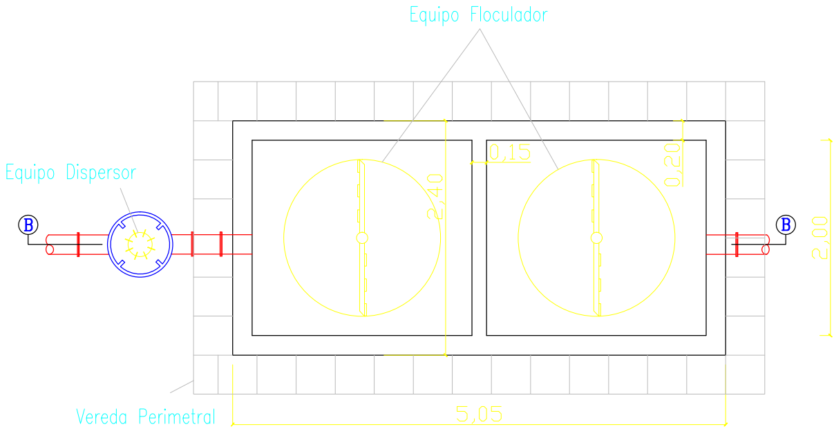
PLANTA
