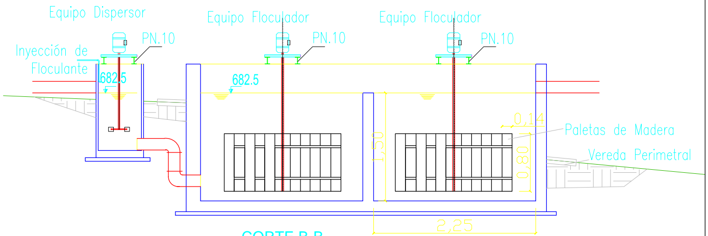
CORTE B-B
