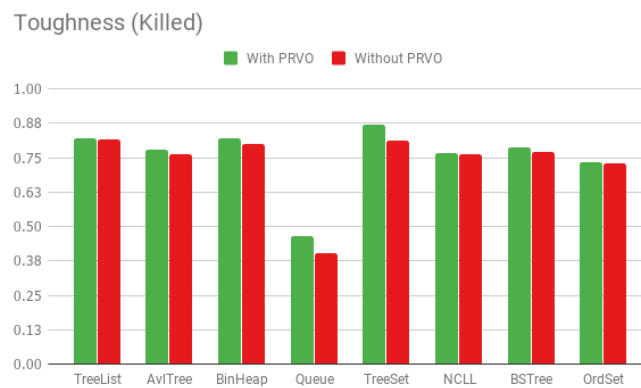
Figura 57: Comparación de Toughness Killed , cuantos tests “resiste” un mutante que fue detectado.
