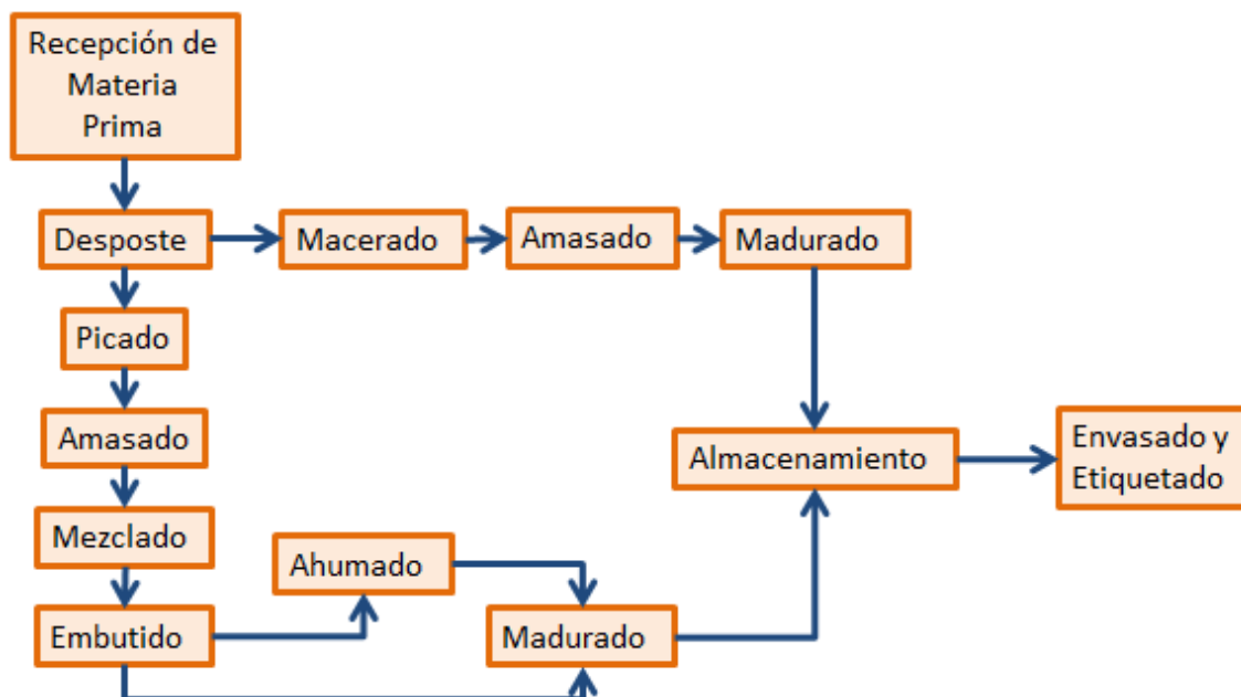
Figura 5: Proceso de producción de salazones secas y embutidos secos en la fábrica de chacinado y despostadero “Manjares Serranos”.
