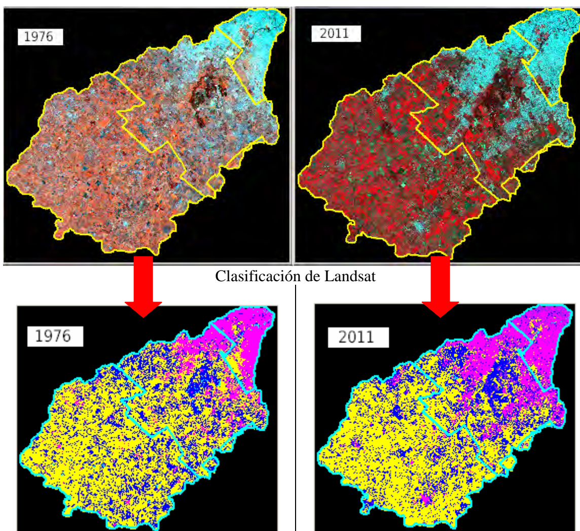
Figura 49 Arriba imágenes Landsat de la cuenca MR de los años 1976 y 2011 y abajo los productos clasificados correspondientes mostrando el área edificada (fucsia).
