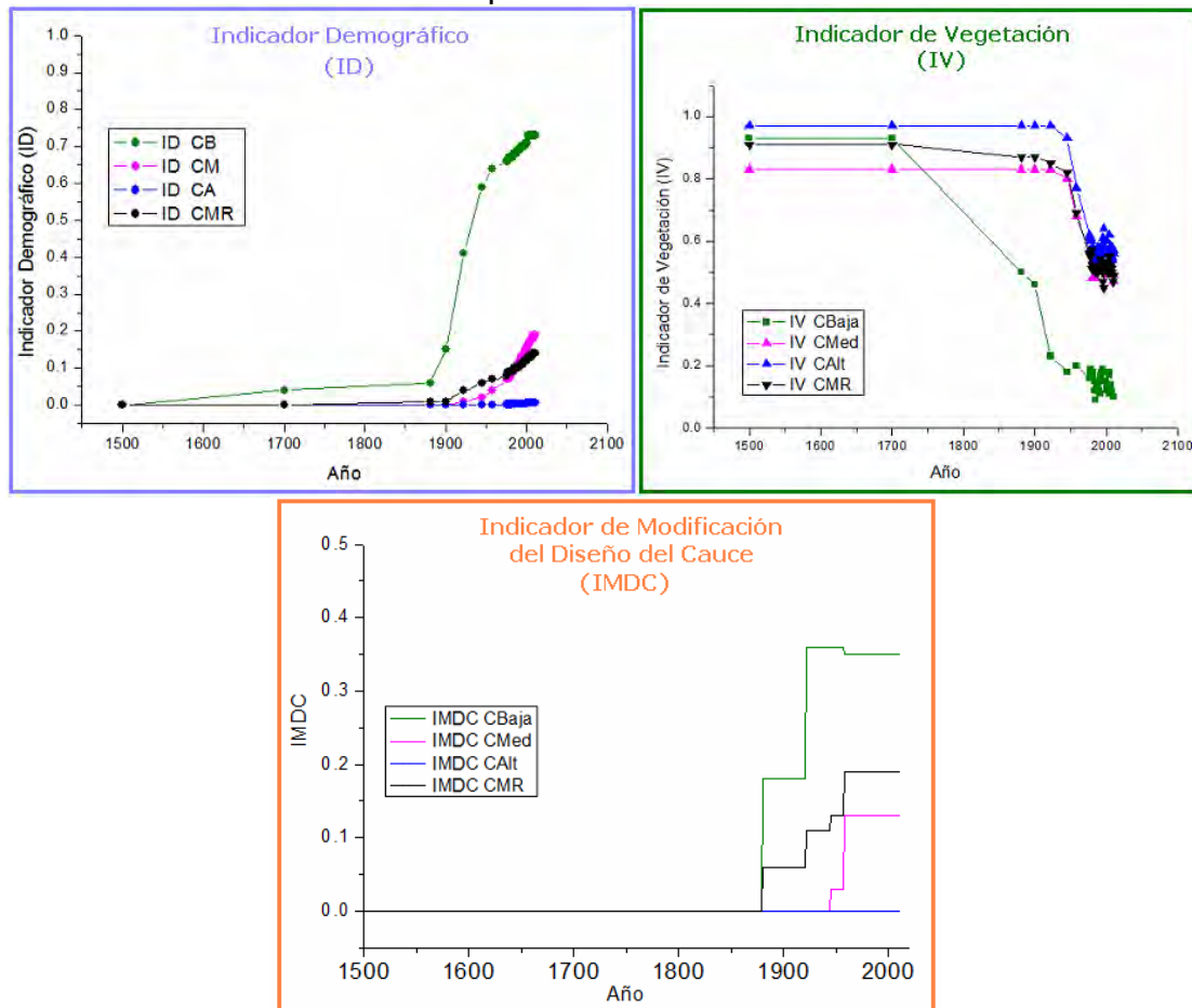
Figura 74 Indicadores entre 1500-2011.
