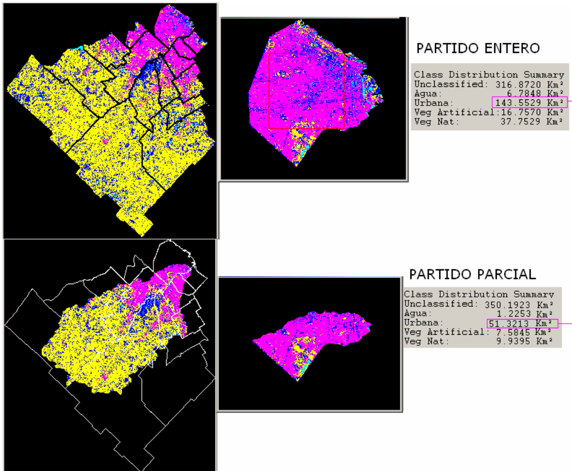
Figura 35 Determinación del área urbana en el partido entero y en el área de dicho partido que corresponde a la cuenca para el 2007.
