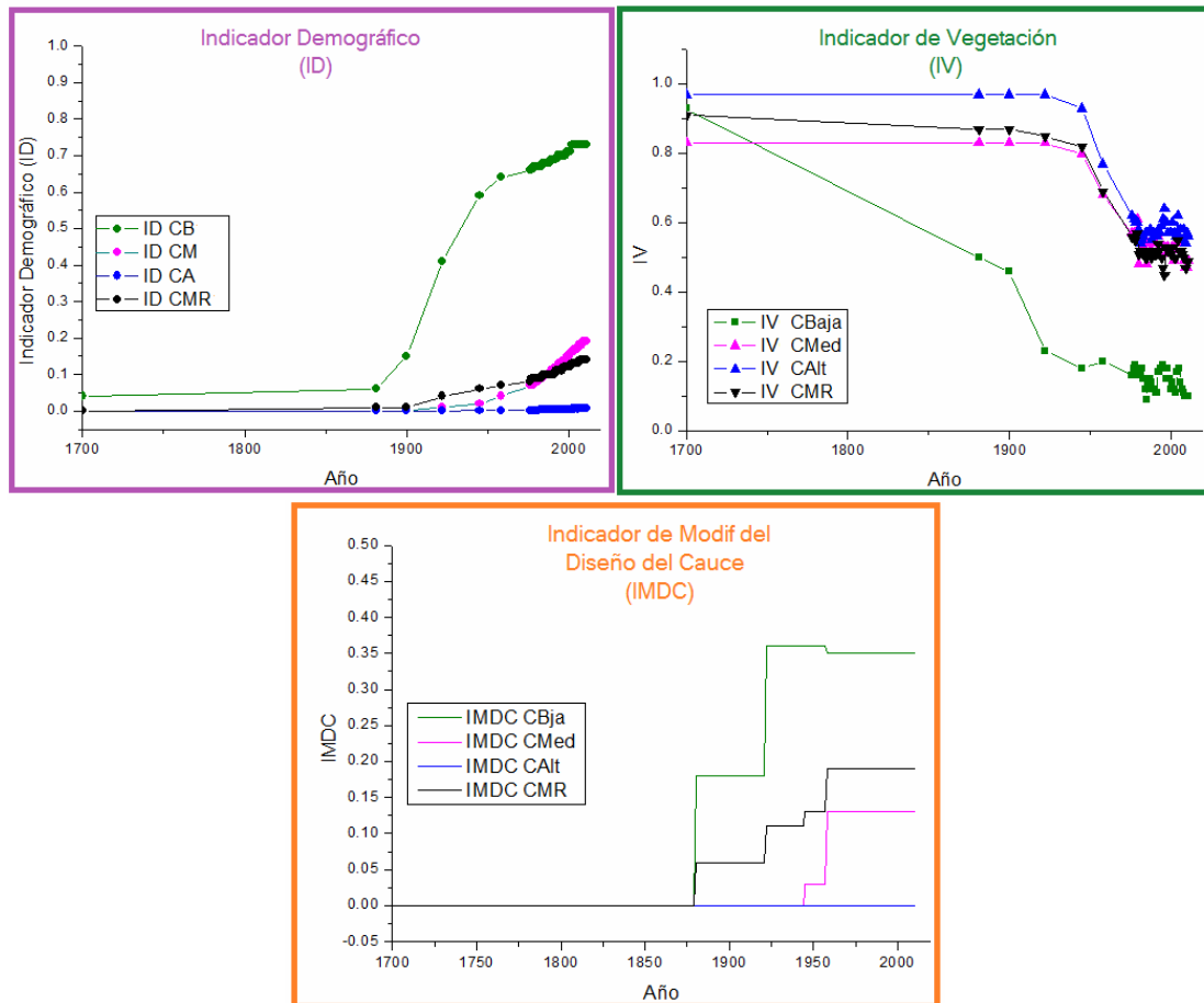
Figura 79 Indicadores 1900-2011.
