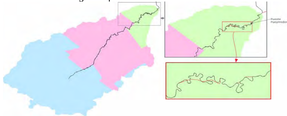
Figura 68 Primera rectificación (aproximadamente 1880)
