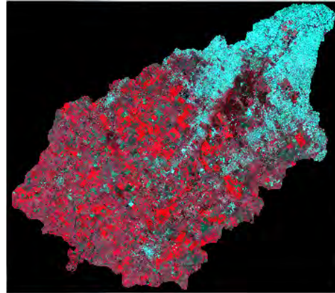
Figura 53 Imagen Landsat TM 2011 de la cuenca MR en falso color compuesto: 5,4,3.
