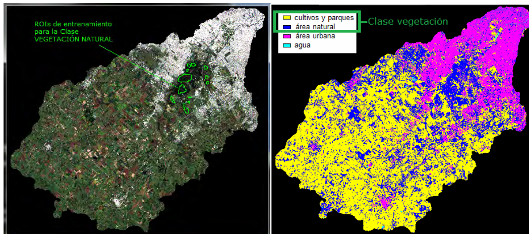
Figura 55 Imagen Landsat 2007 mostrando los ROIs para la clase vegetación natural (izquierda) y producto clasificado (derecha).
