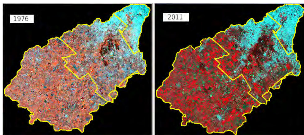
Figura 31 Imagen Landsat de la CMR en 1976 y 2011, donde se puede visulalizar la zona urbanizada en turquesa y la zona agrícola en rojo.
