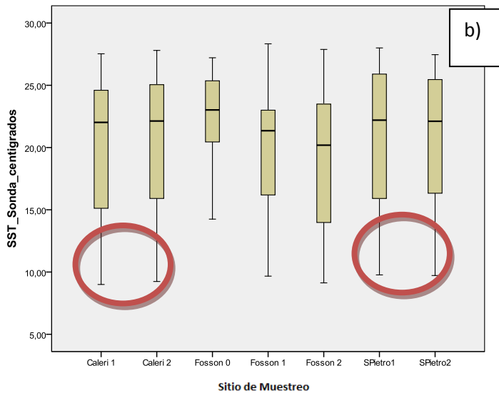
Graf. 29: Variación entre sitios de muestreo de datos de temperatura superficial del mar del sensor MODIS a) y de la sonda multiparametrica b). Los círculos granate señalan a las estaciones Caleri 1 y 2, San Pietro 1 y 2 que poseen un comportamiento muy similar para las mediciones in situ y por MODIS
