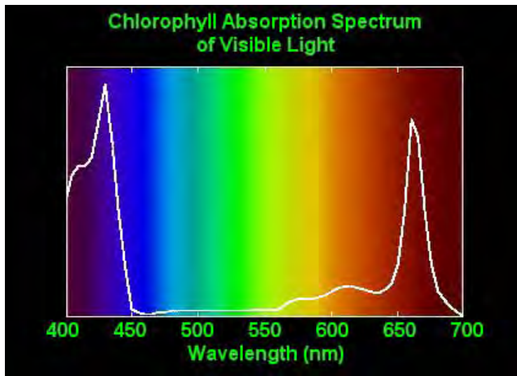
Graf. 1: Espectro de absorción de la clorofila para el rango visible
