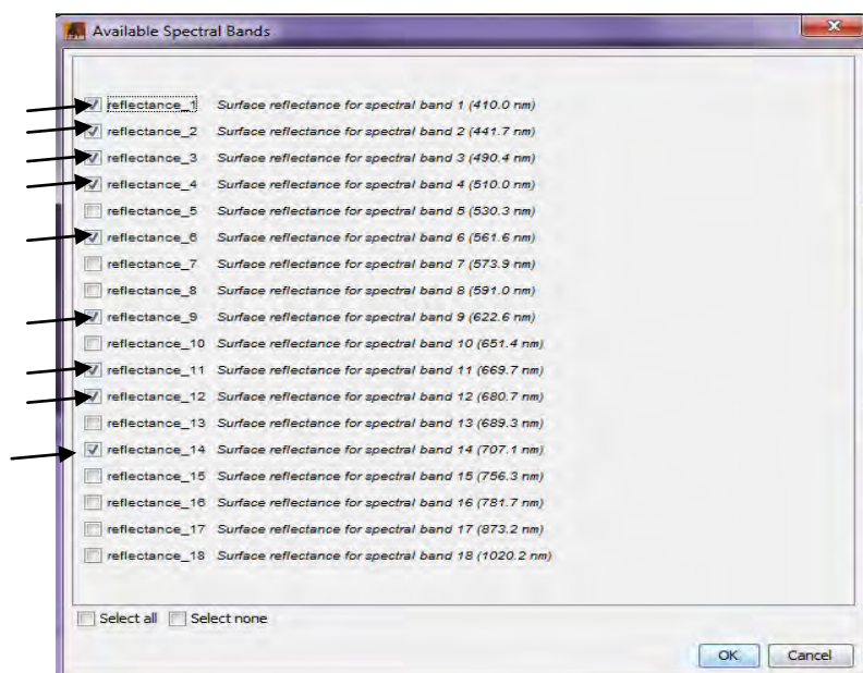
Fig.26 : bandas de reflectancia de CHRIS-Proba utilizadas (señaladas por las flechas negras) y su longitud de onda media
