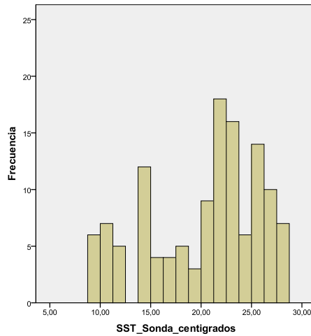
Graf. 17 b: distribución original de SST sensada por sonda multiparametrica (°C)
