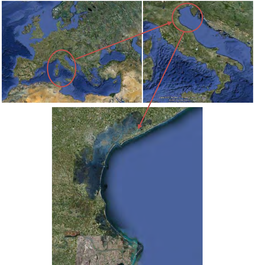
Fig. 10: Situación geográfica de la Costa Veneta en el Norte Adriático de Italia
