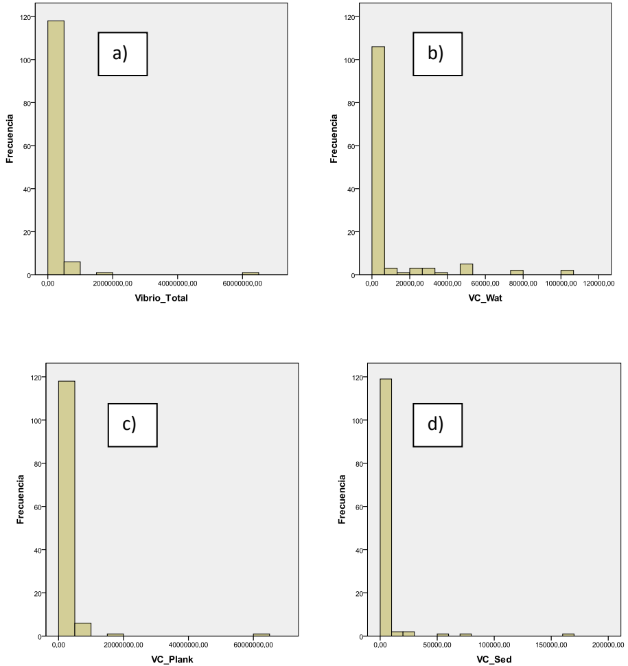
Graf. 22: Distribución original de la concentración de Total (a) dispersos en el agua (b), adheridos al plancton (c) y en el sedimento (d).
