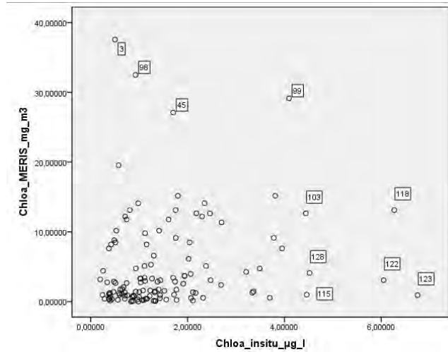
Graf.2: dispersión de puntos para el conjunto de valores original de clorofila-a
