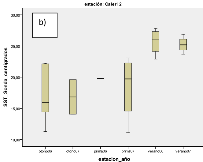
Graf. 30: Variación estacional del sitio de muestreo Caleri 2 como se midió por MODIS (a) y mediante sonda multiparametrica (b), muy similar a Caleri 1 (gráfico no mostrado) posiblemente por su cercanía geográfica.
