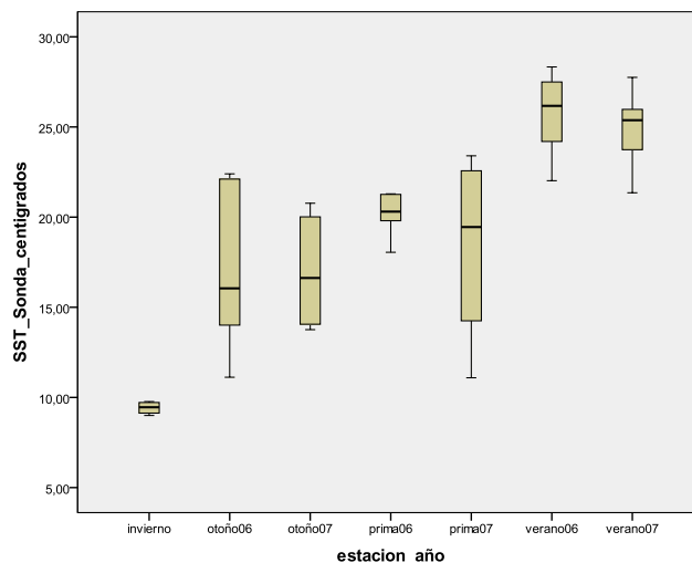
Graf. 27: Variación estacional de la temperatura superficial del mar, datos de la sonda multiparametrica para las diferentes estaciones del año
