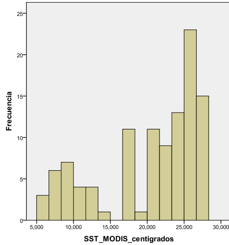
Graf. 17 a: distribución original de SST sensada por MODIS (°C)
