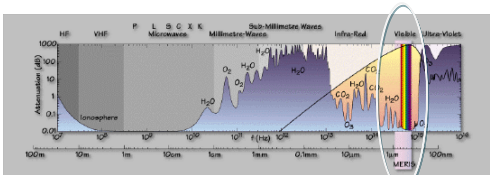
Fig. 14: Espectro electromagnético de los datos medidos por MERIS
