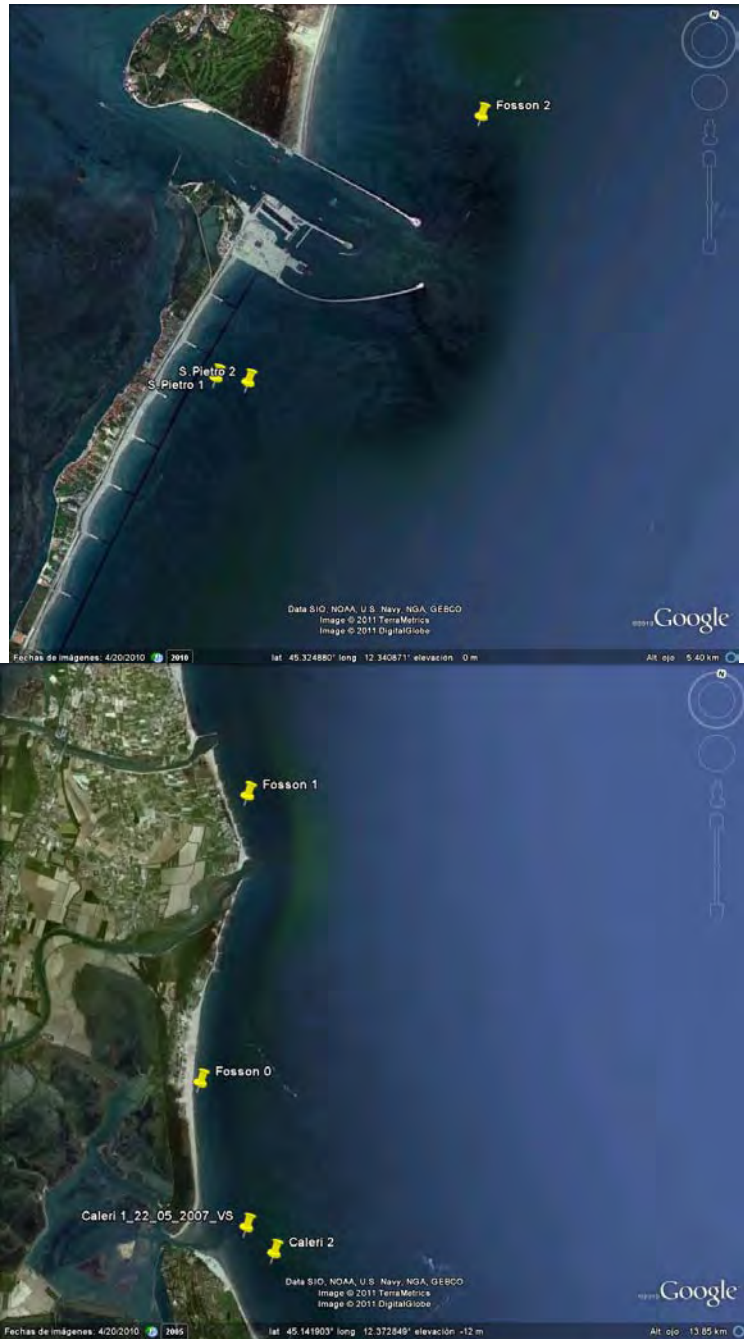
Fig. 13: Ubicación de los sitios de muestreo a lo largo de la costa Veneta
