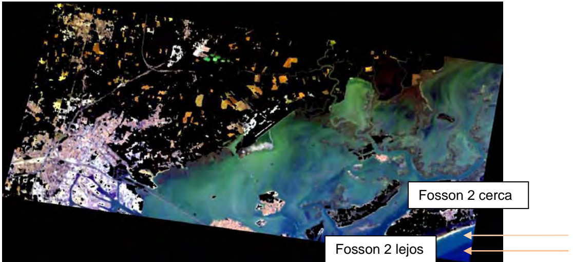
Fig.28: Imagen VN_040703 de CHRIS-Proba, obtenida del procesador VISAT, cubriendo solamente el sitio de muestreo Fossom 2. Se establecieron dos puntos uno más cercano y el otro más lejano a la costa. La composición de bandas RGB de 12, 7, 1 (longitudes de onda de 680.7nm, 573.9nm, 410nm)
