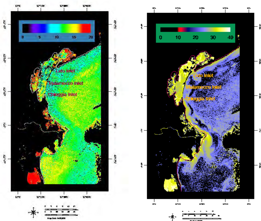
Fig. 15.a: Índice de pigmento de fitoplancton (Concentración de clorofila-a \mu\text{g/l} )
