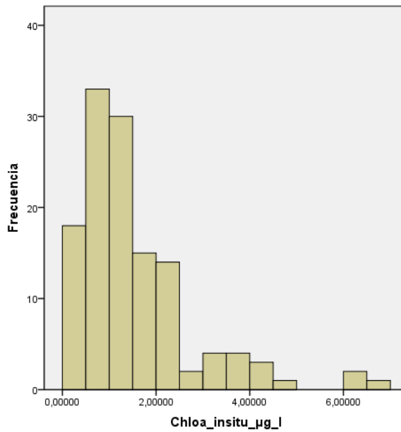
Graf. 6 b: distribución original de la clorofila-a sensada por sonda multiparametrica (µg_l)
