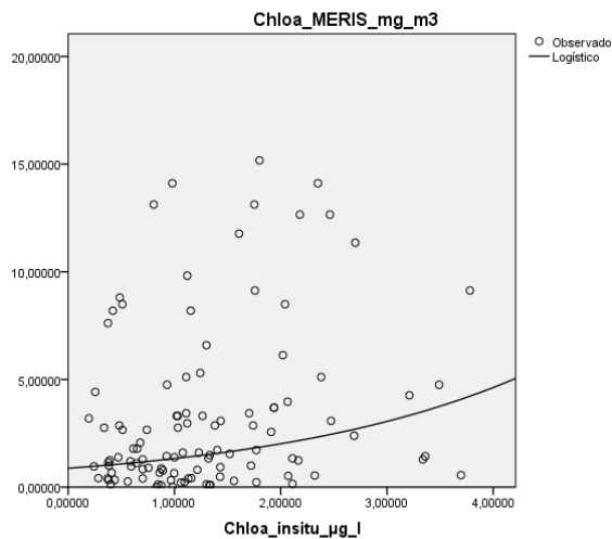
Graf. 10: la regresión logística con un R: 19.6% es el mejor ajuste entre datos in-situ y MERIS para concentración de clorofila-a
