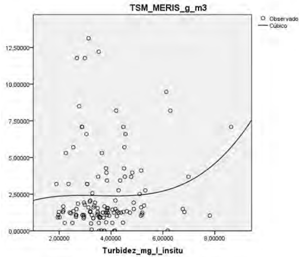
Graf. 16: la regresión cúbica con un R: 13.6\% es el mejor ajuste entre datos in-situ y MERIS para concentración de materia total en suspensión
