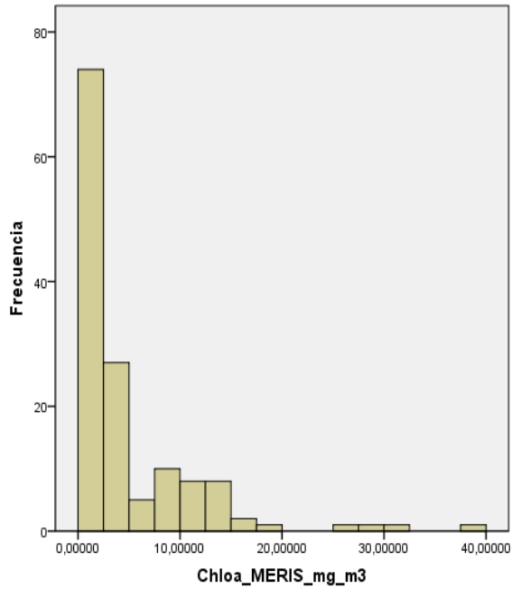
Graf. 6 a: distribución original de la clorofila-a sensada por MERIS (mg_m3)
