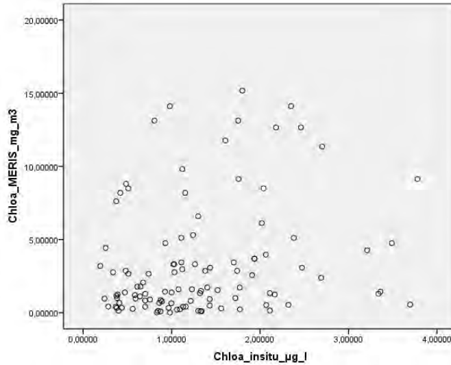
Graf. 3: patrón final de la nube de puntos de valores de clorofila-a utilizado para los análisis posteriores
