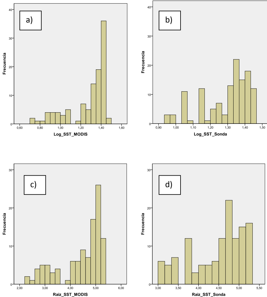
Graf. 19: Distribución de la temperatura superficial del mar por MODIS luego de aplicar logaritmo en base 10 y raíz cuadrada (a y c) y de temperatura superficial del mar medida por sonda multiparametrica luego de aplicar logaritmo en base 10 y raíz cuadrada (b y d).
