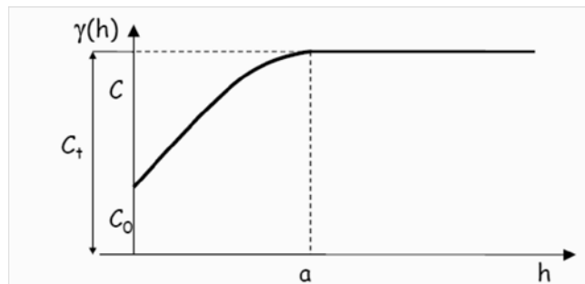
Fig. 17: forma tradicional de un Variograma, donde se grafica la semivarianza en función de diferentes distancias entre pares de puntos
