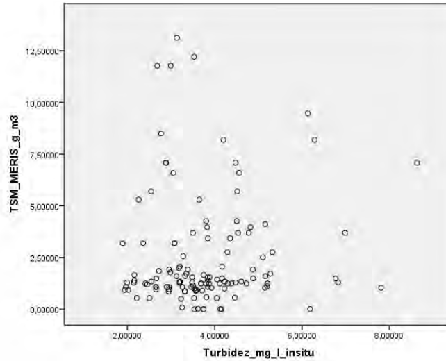
Graf. 5: patrón final de la nube de puntos de valores de materia total en suspensión utilizado para los análisis posteriores
