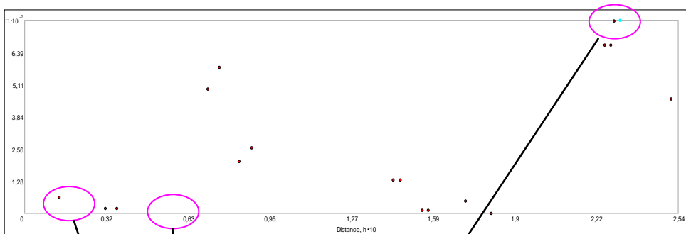
Graf. 35: gráfico de salida como semivariograma
