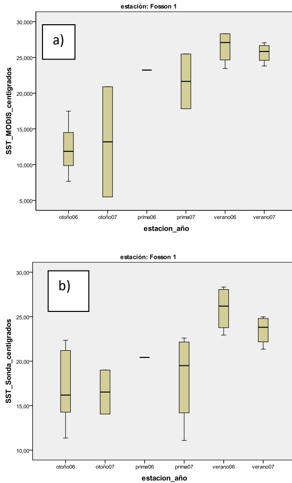
Graf. 31: Variación estacional del sitio de muestreo Fosso 1 como se midió por MODIS (a) y mediante sonda multiparametrica (b) enseñando la disparidad en la variabilidad captada por ambos sistemas de medición
