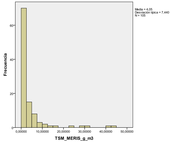
Graf. 14 a: distribución original de TSM sensada por MERIS ( \text{g}/\text{m}^3 )
