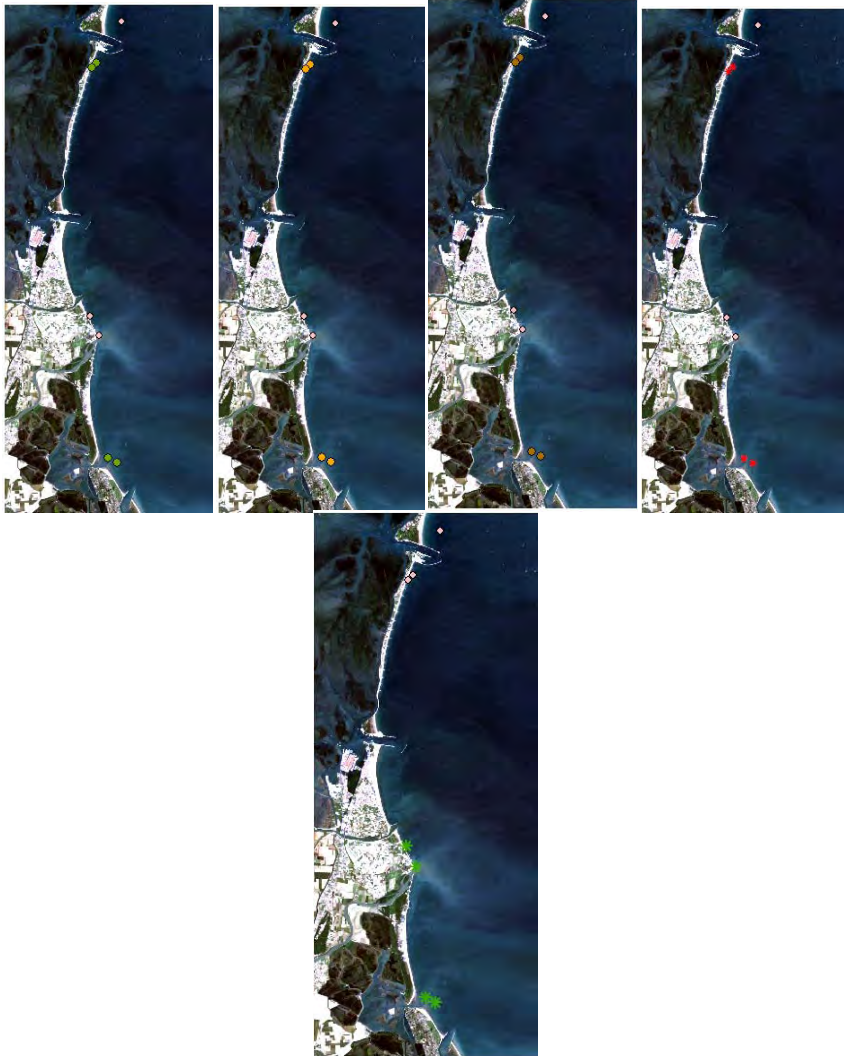
Fig. 19 : distribución de las estaciones de muestreo con similares co-variaciones en sus valores analizadas durante el 2007 (imagen color real LANDSAT5 TM Abril 2010)
