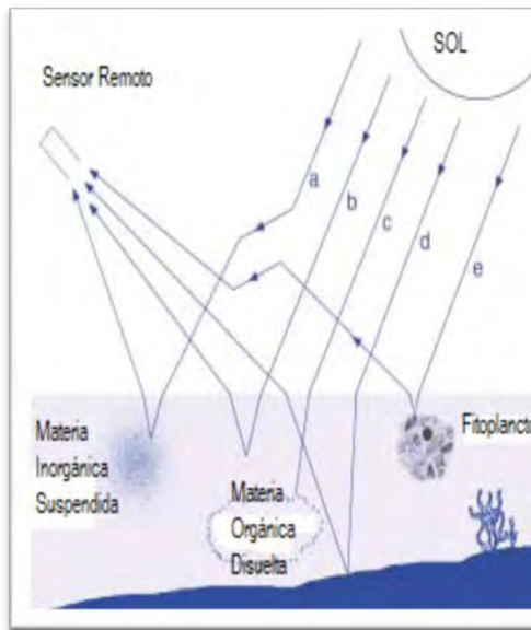
Fig. 3: Factores que influyen la Luz que alcanza al sensor. Adaptado de Sathyendranath (1986).
