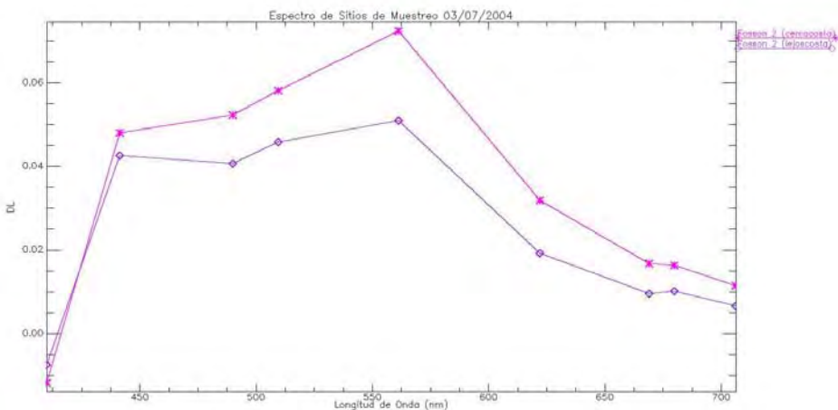
Graf. 42: firma espectral de Fossom 2 mas cerca y mas lejos de la costa obtenida de VN_040703
