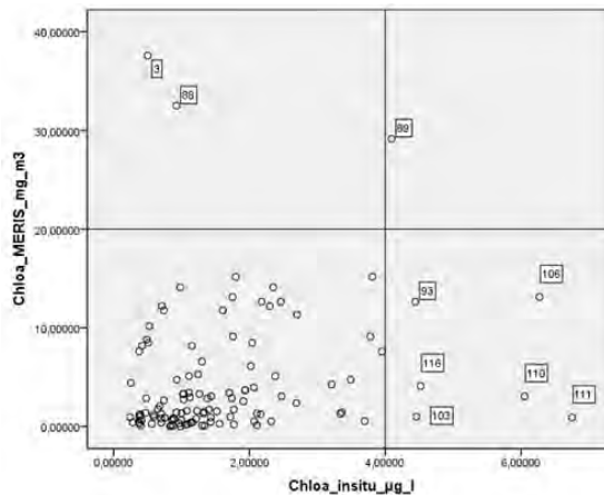
Graf. 8: conjunto de datos con los que la correlación presenta un R: 0.24
