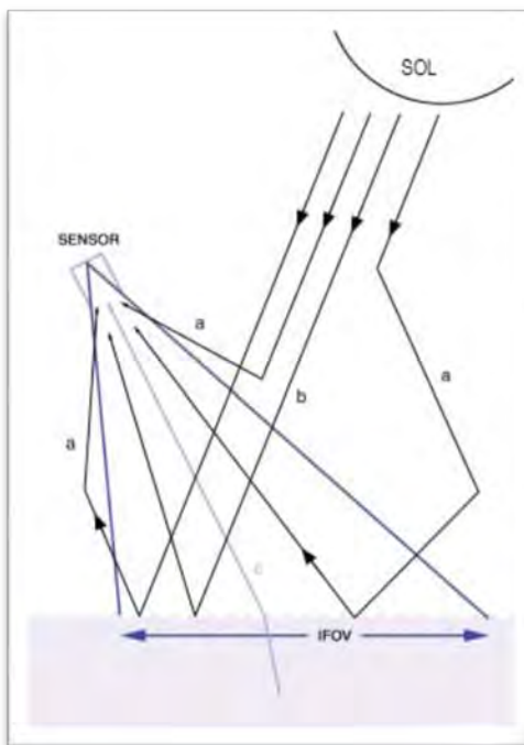
Fig. 2: ¿Cómo llega la luz al sensor remoto?
