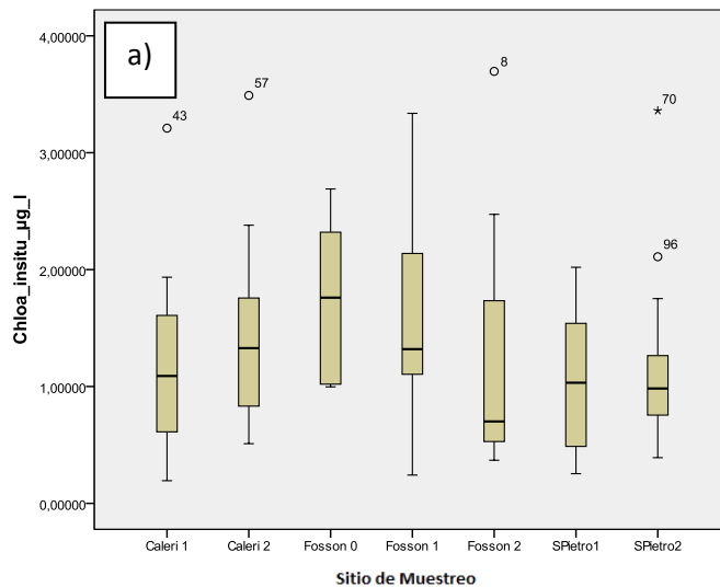
Graf. 25 a): Variación entre sitios de muestreo de clorofila-a datos medidos por sonda multiparametrica
