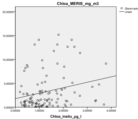
Graf. 11: regresión lineal entre datos in-situ y MERIS para concentración de clorofila-a
