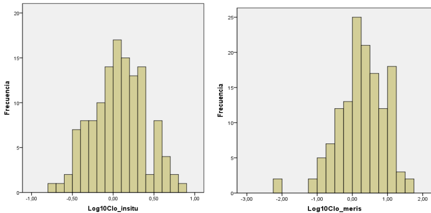
Graf. 12: distribución logarítmica de la clorofila-a in-situ y clorofila-a sensada por MERIS
