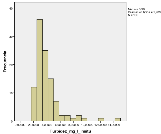
Graf. 14 b: distribución original de TSM sensada por sonda multiparametrica ( \text{mg}/\text{l} )
