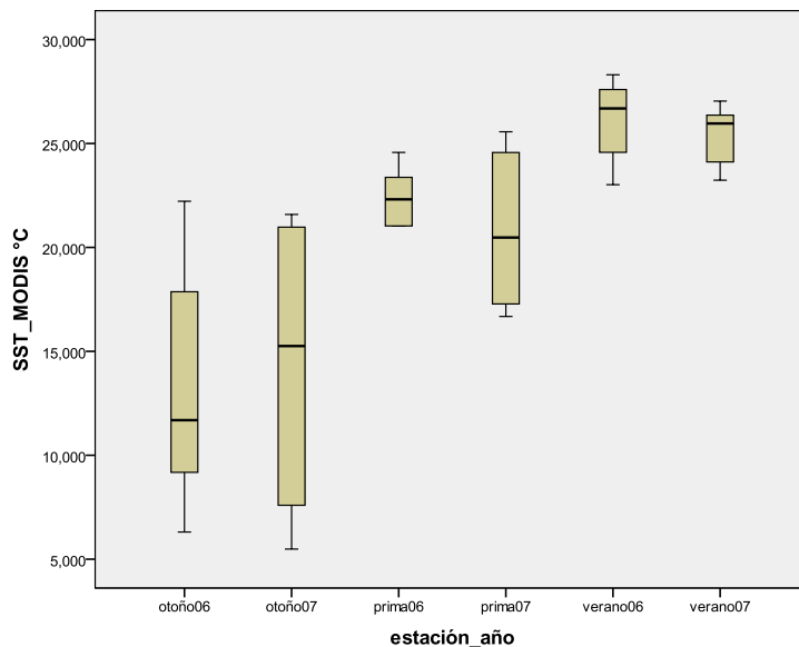
Graf. 26: Variación estacional de la temperatura superficial del mar, datos del sensor MERIS para las diferentes estaciones del año.
