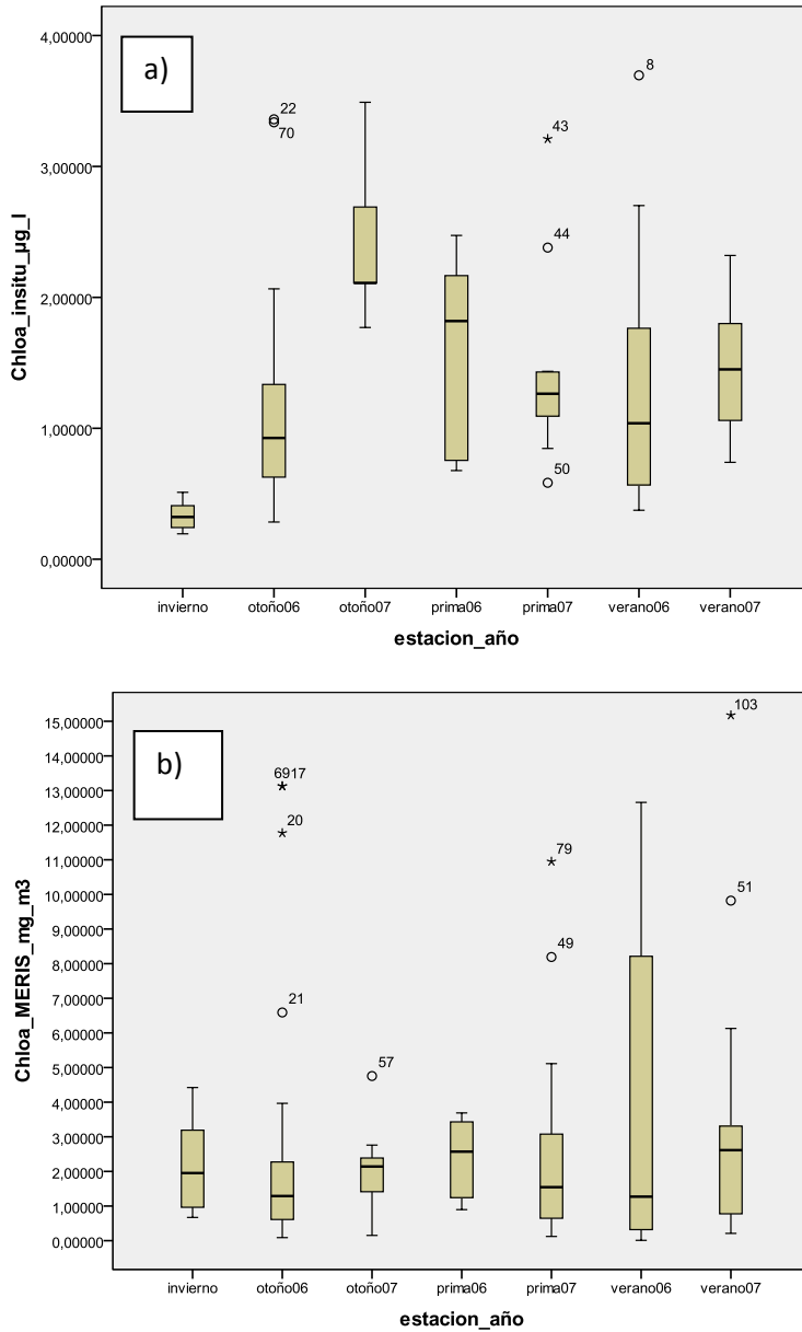
Graf. 24: Variación estacional de clorofila-a; a) datos medido in-situ, b) datos del sensor MERIS para las diferentes estaciones del año.
