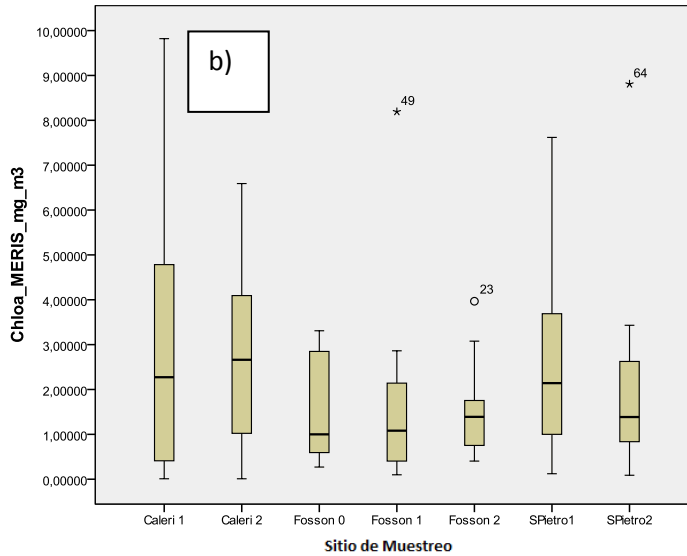
Graf. 25 b): Variación entre sitios de muestreo de clorofila-a datos del sensor MERIS a lo largo de los dos años de muestreo.
