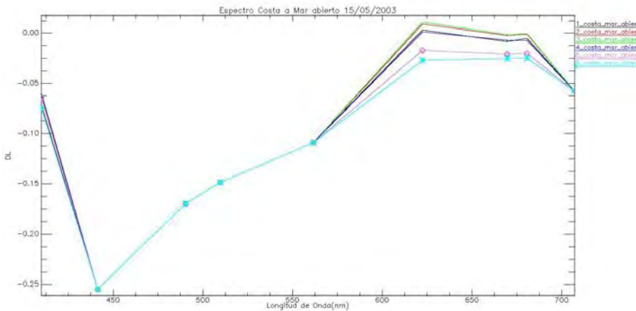
Graf.44 : firma espectral de zonas ubicadas a distancias mayores de la costa, obtenida de VN_030515
