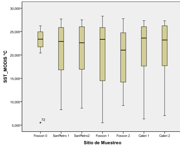
Graf. 28: Variación entre sitios de muestreo de datos de temperatura superficial del mar del sensor MODIS a lo largo de los dos años de muestreo.
