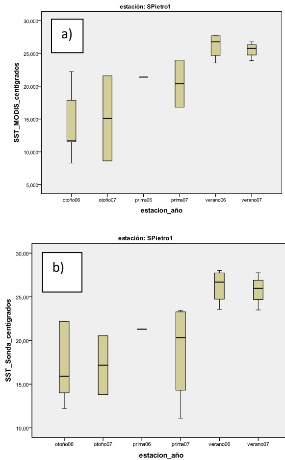
Graf. 32: Variación estacional del sitio de muestreo San Pietro 1 como se midió por MODIS (a) y mediante sonda multiparametrica (b) enseñando la disparidad en la variabilidad captada por ambos sistemas de medición
