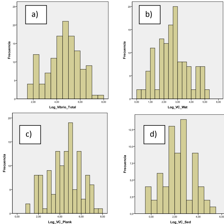
Graf. 23: : Distribución de la concentración de Total (a) dispersos en el agua (b), adheridos al plancton (c) y en el sedimento (d) luego de aplicar logaritmo en base 10 a los datos
