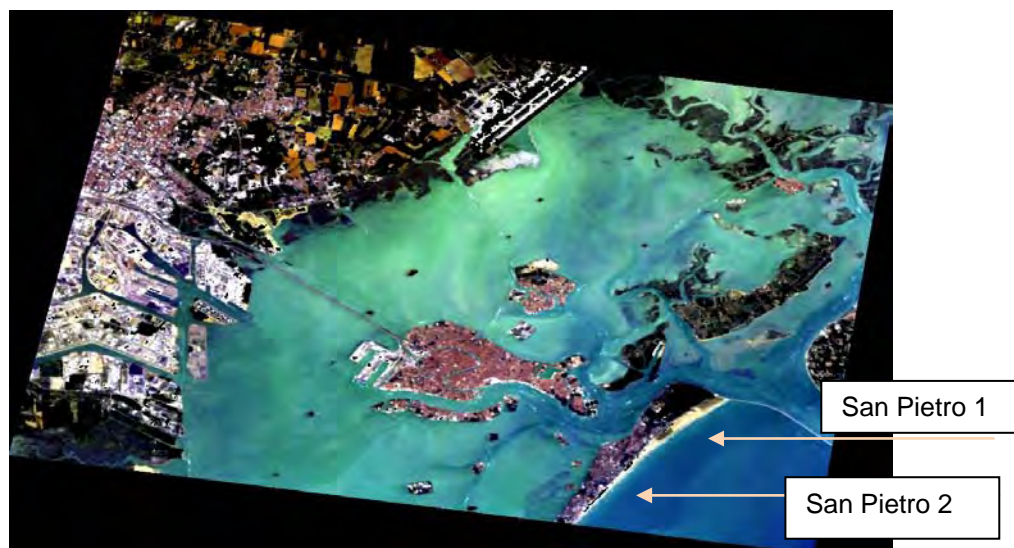
Fig.29: Otra sección de la imagen VN_040703 de CHRIS-Proba, obtenida del procesador VISAT, cubriendo solamente los sitios de muestreo San Pietro 1 y 2. La composición de bandas RGB de 12, 7, 1 (longitudes de onda de 680.7nm, 573.9nm, 410nm)
