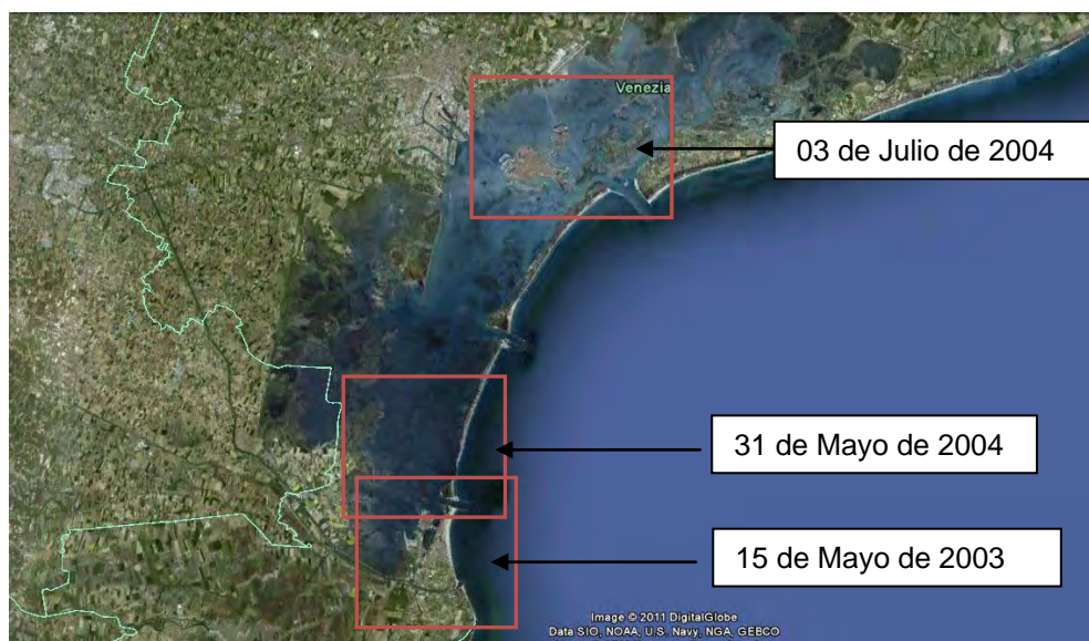
Fig. 25 : localización de las imágenes adquiridas por CHRIS_Proba y utilizadas en el análisis junto con sus respectivas fechas de adquisición
