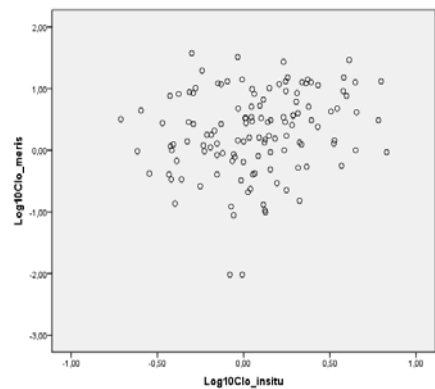
Graf. 12: distribución logarítmica de la clorofila-a in-situ y clorofila-a sensada por MERIS
