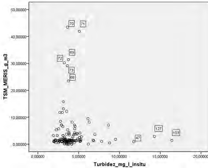
Graf.4: dispersión de puntos para el conjunto de valores original de materia total en suspensión
