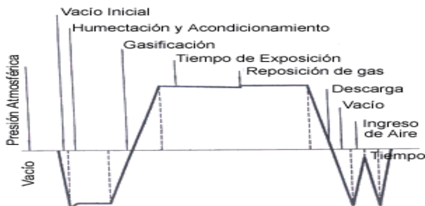
Figura 4. Grafico ciclo de esterilización por óxido de etileno.
