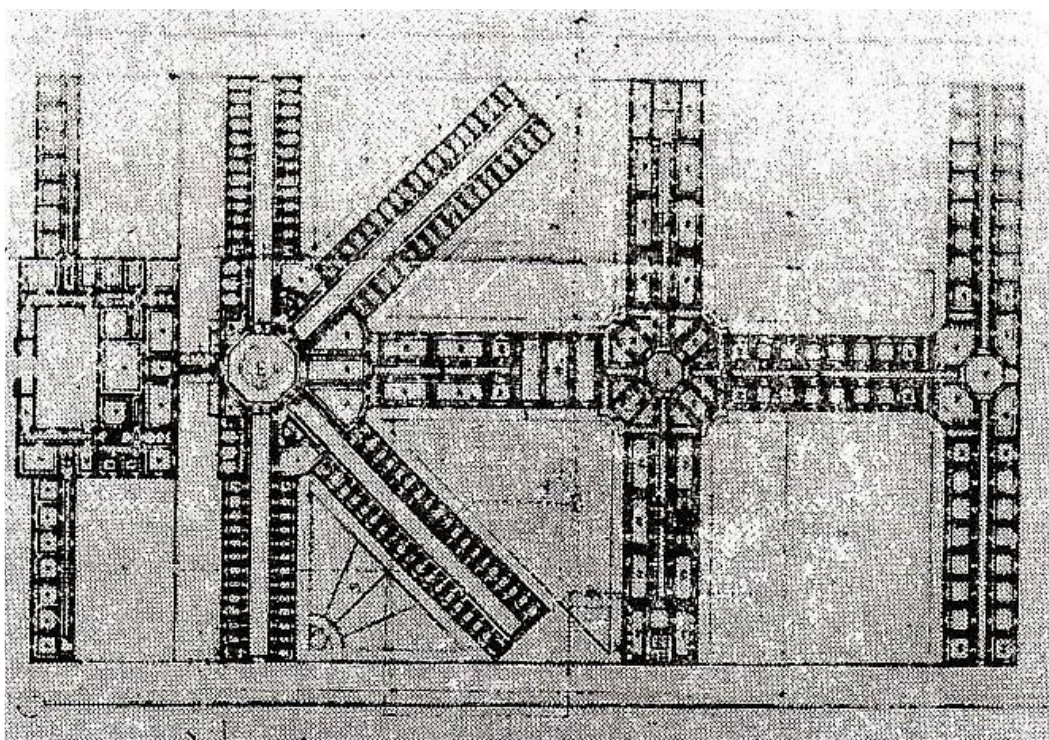
2. Planos del proyecto original de la penitenciaría de Córdoba (Planta en abanico). Archivo de la Dirección de Arquitectura de la Provincia de Córdoba.
